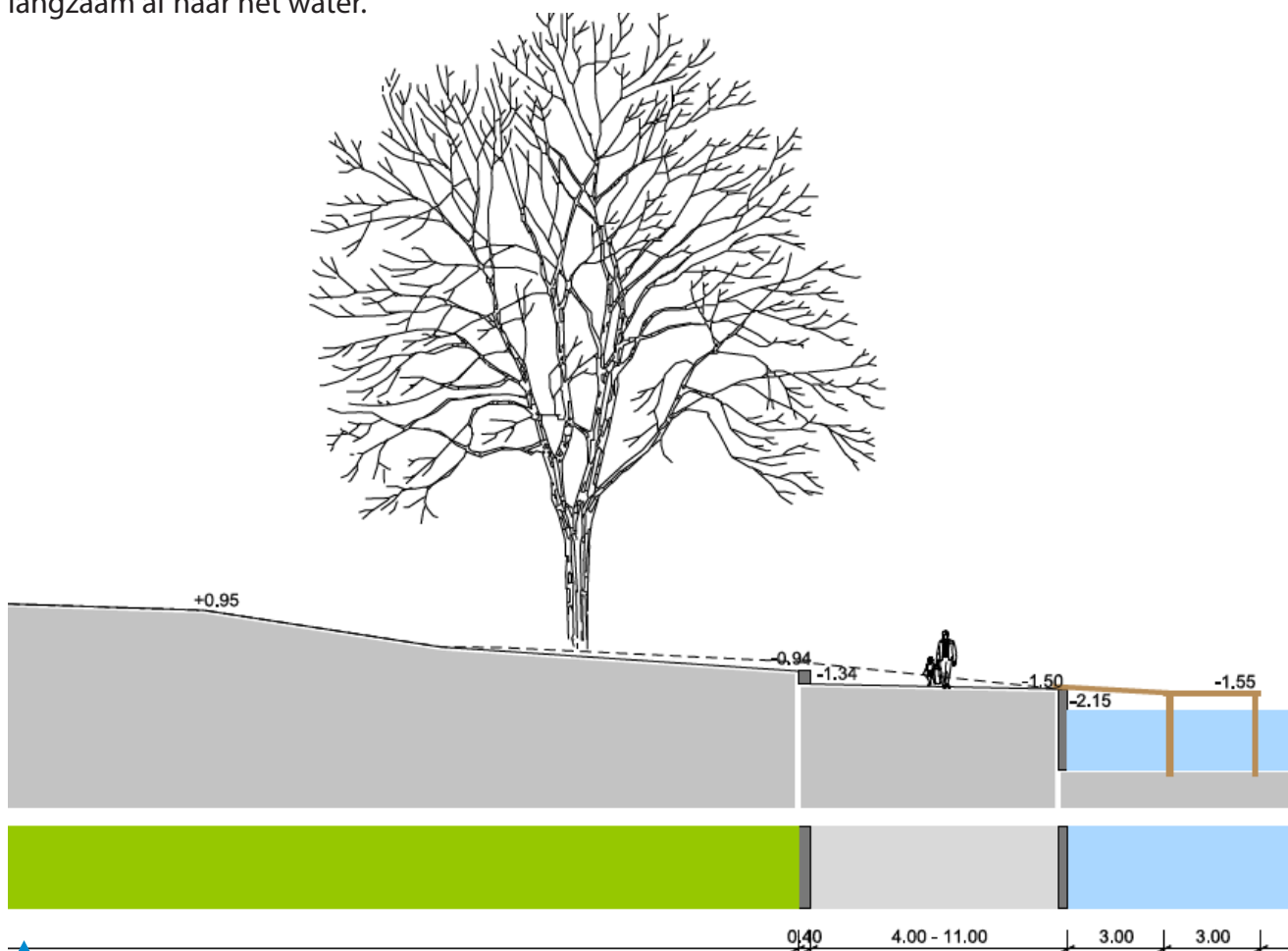
▲ Hoogte verschil rand en midden van landtong
