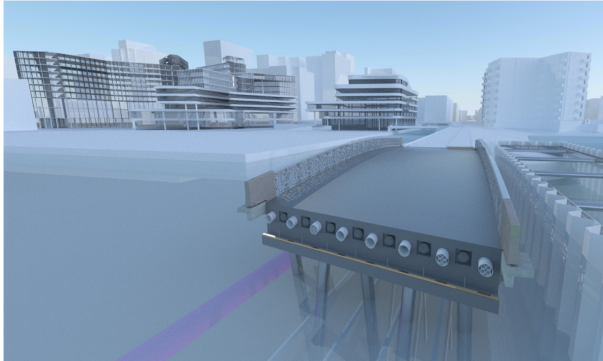
Kabels en Leidingen in brug Beatrixpark
