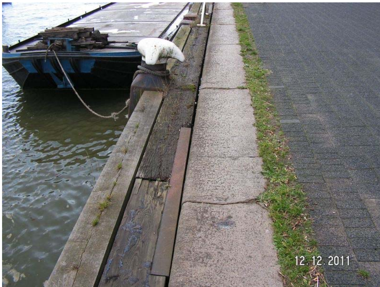
Foto 12 koningspaal en gordingen
