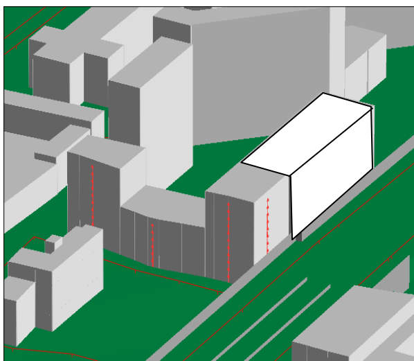
Figuur 9: variant GD-5 met ligging waarneempunten
