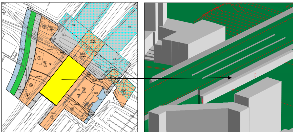
Figuur 10: GD-6 met ligging waarneempunten
