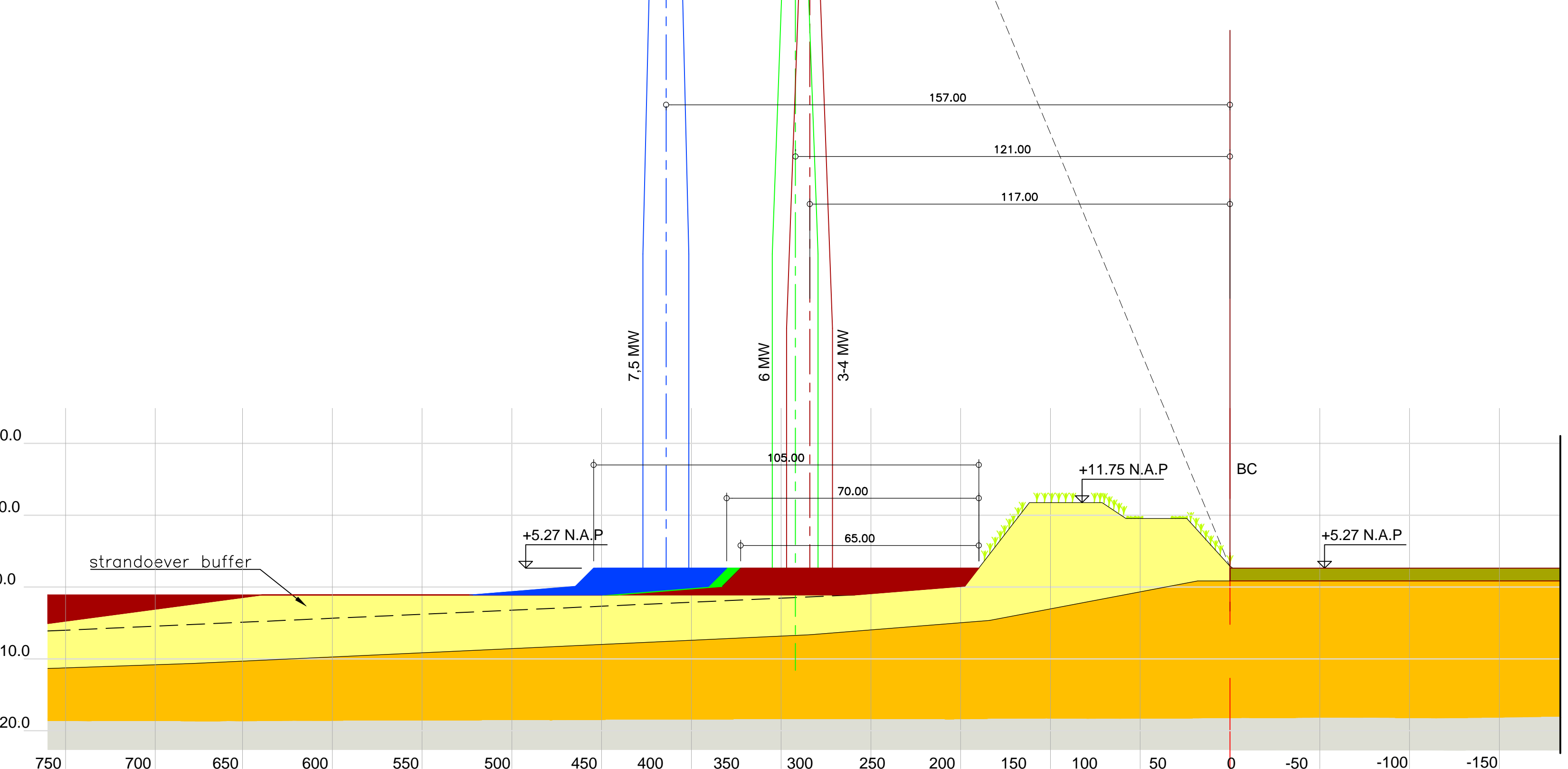
Dwarsdoorsnede Horizontaleschaal 1:1000 Verticaleschaal 1:1000
