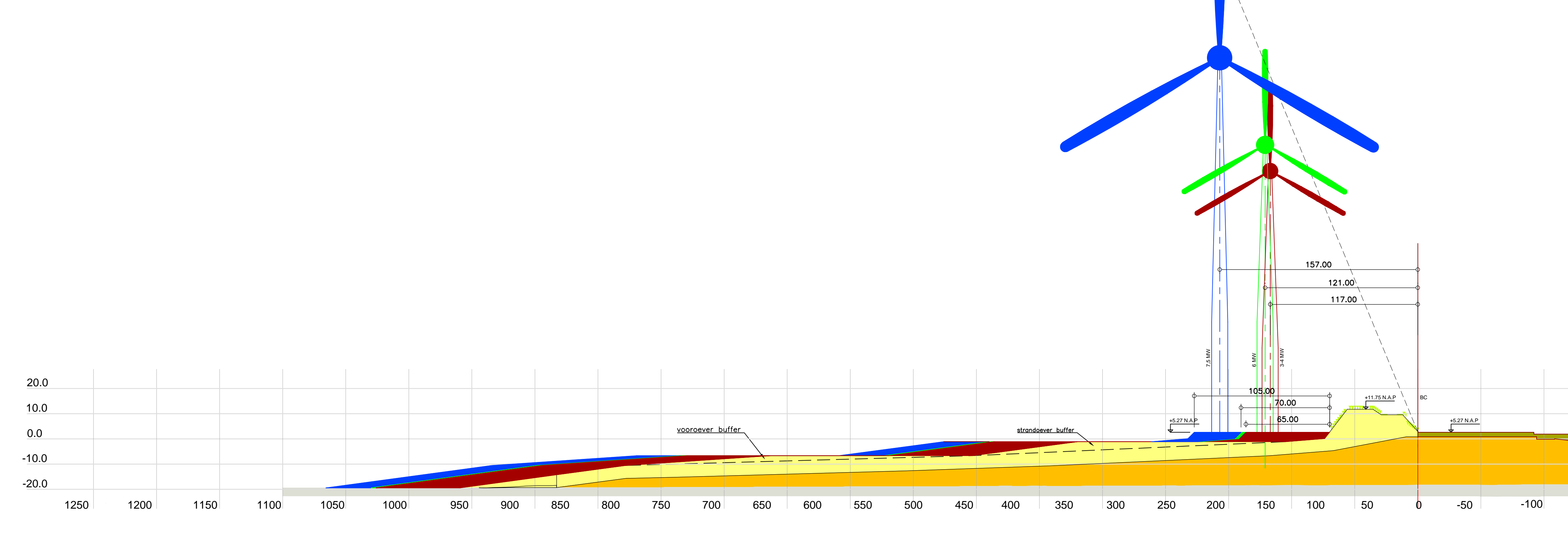
Dwarsdoorsnede Horizontaleschaal 1:2000 Verticaleschaal 1:1000
