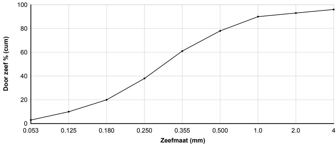
Korrelverdelingsdiagram
