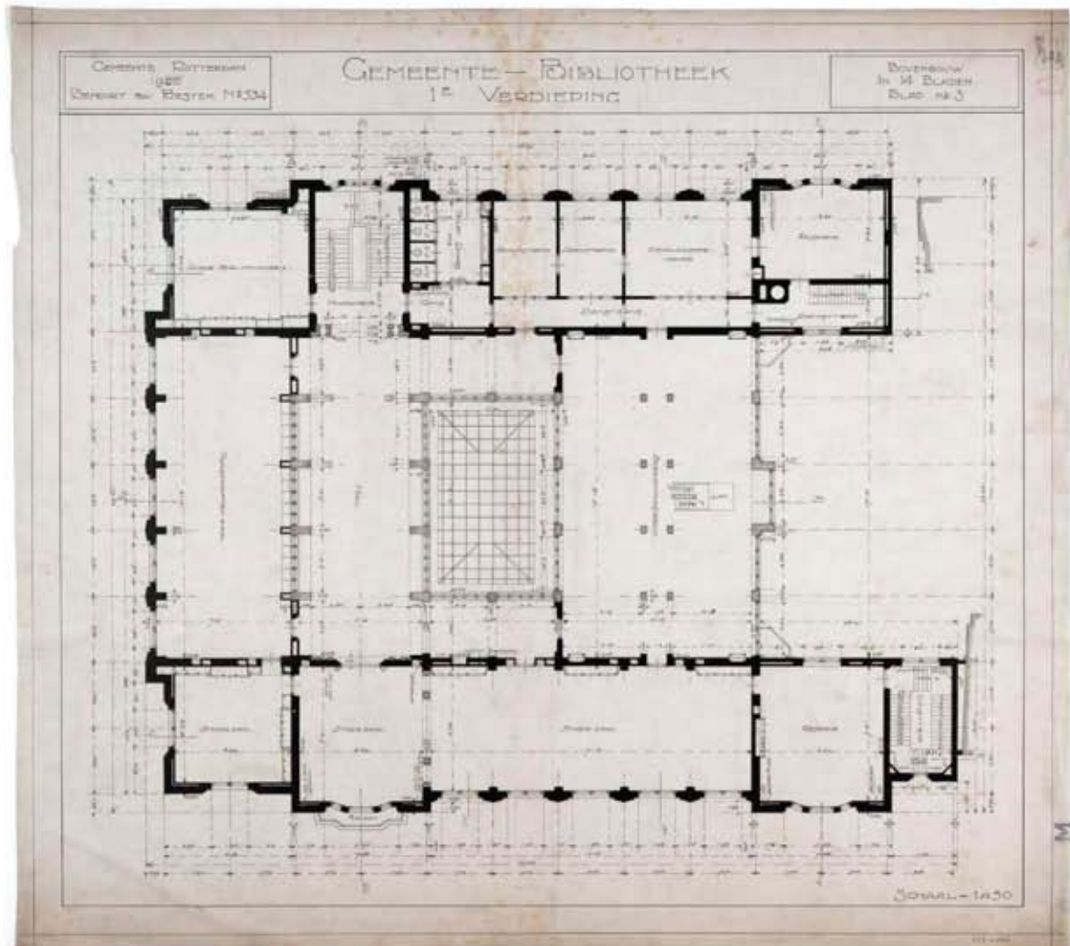
Afb. 3. Plattegrond eerste verdieping; bestektekening 1920 [Gemeentearchief Rotterdam, Archief Fabricage, Commissie Plaatselijke werken, Dienst van Gemeentewerken, inv.nr. 3646]
