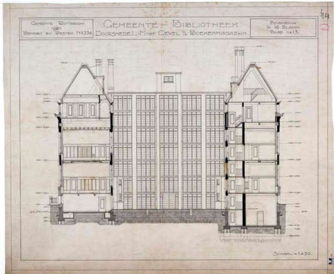
Afb. 13. Doorsnede L - K met gevel van het boekenmagazijn; bestektekening 1920 [Gemeentearchief Rotterdam, Archief Fabricage, Commissie Plaatselijke werken, Dienst van Gemeentewerken, inv.nr. 3646]
