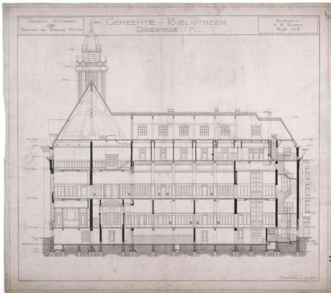
Afb. 12. Doorsnede I-K; bestektekening 1920 [Gemeentearchief Rotterdam, Archief Fabricage, Commissie Plaatselijke werken, Dienst van Gemeentewerken, Inv.nr. 3646]
