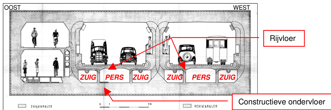
Figuur 1: Maastunnel doorsnede Riviertunnel
