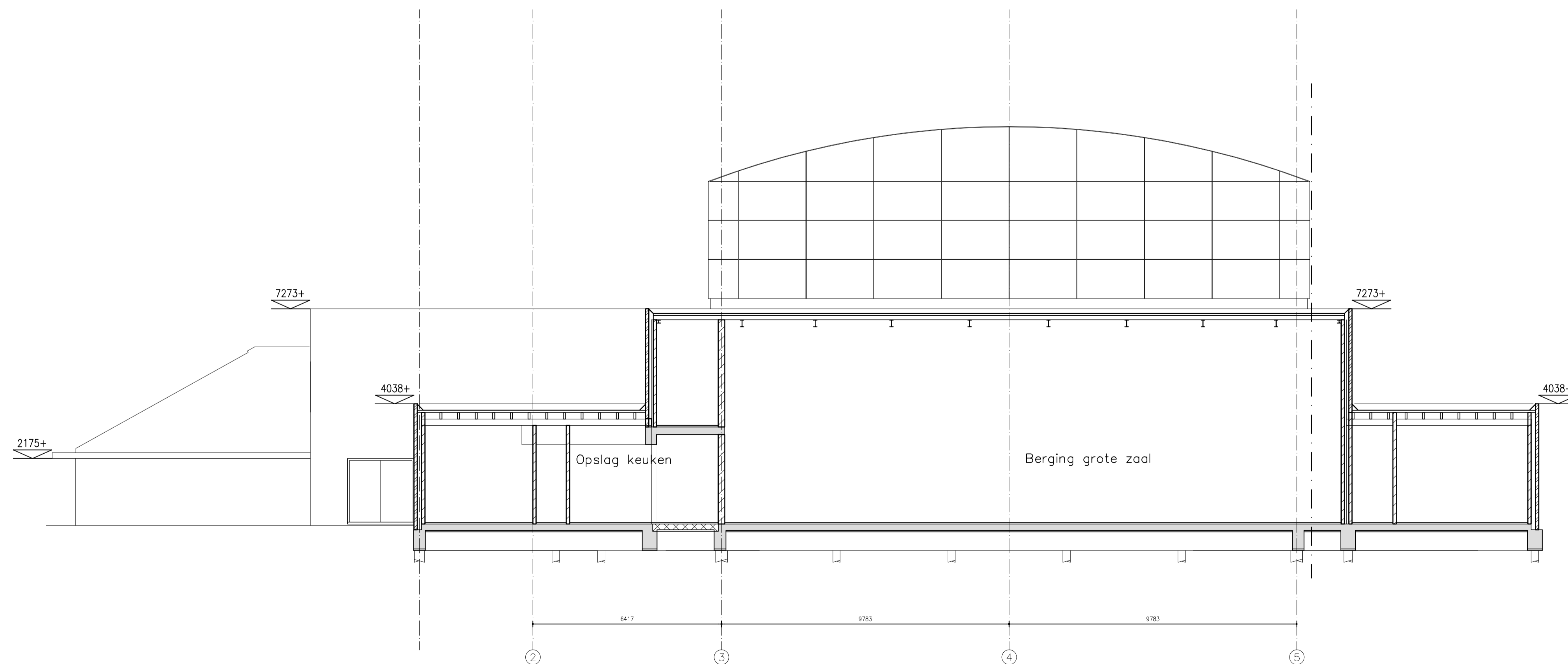
Doorsnede d-d'
