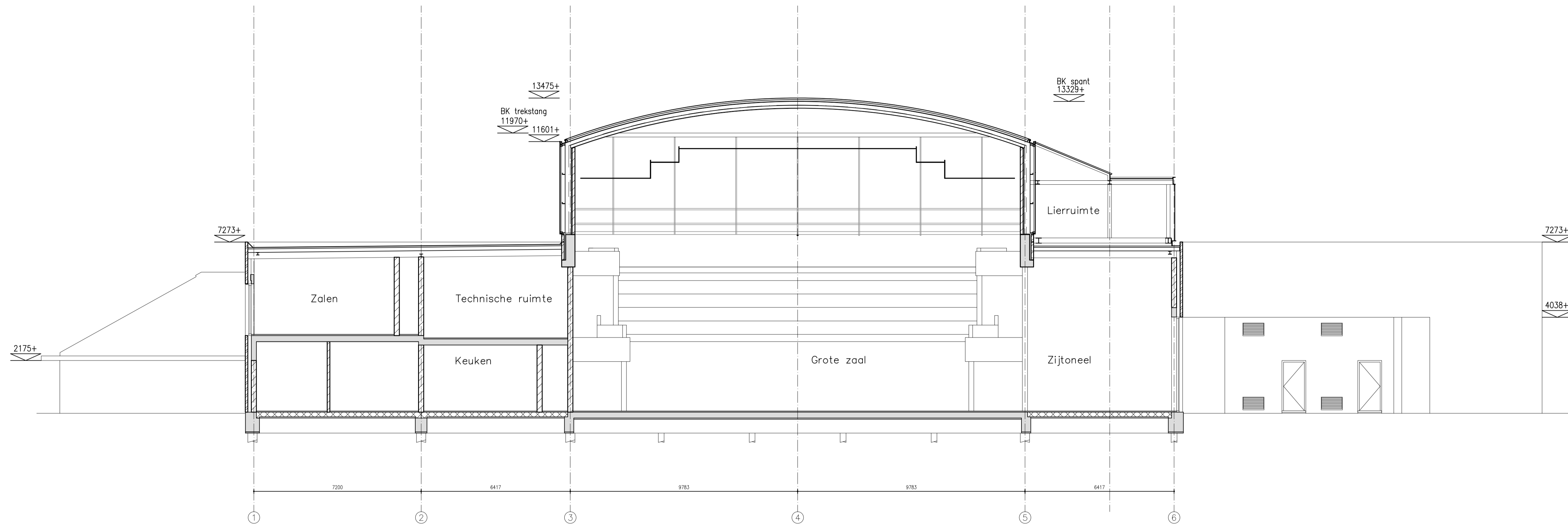
Doorsnede c-c'
