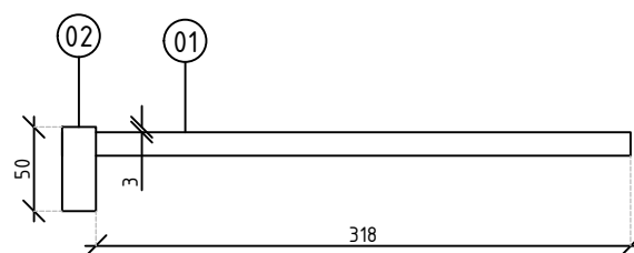
Detail (vol)staf zijaanzicht
