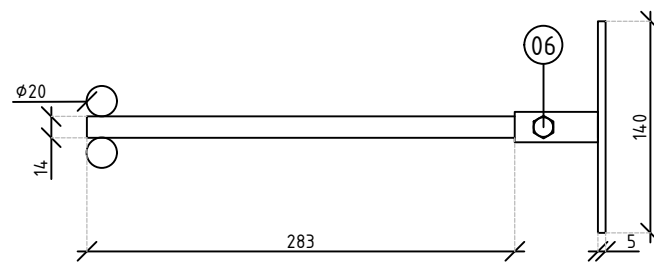
Detail geleidebuis houder bovenaanzicht
