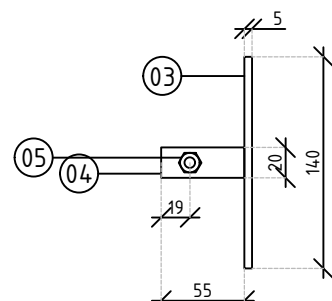
Detail koker bovenaanzicht
