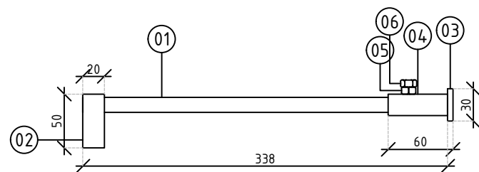
Detail geleidebuis houder zijaanzicht
