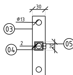
Detail koker vooraanzicht
