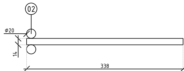
Detail (vol)staf bovenaanzicht
