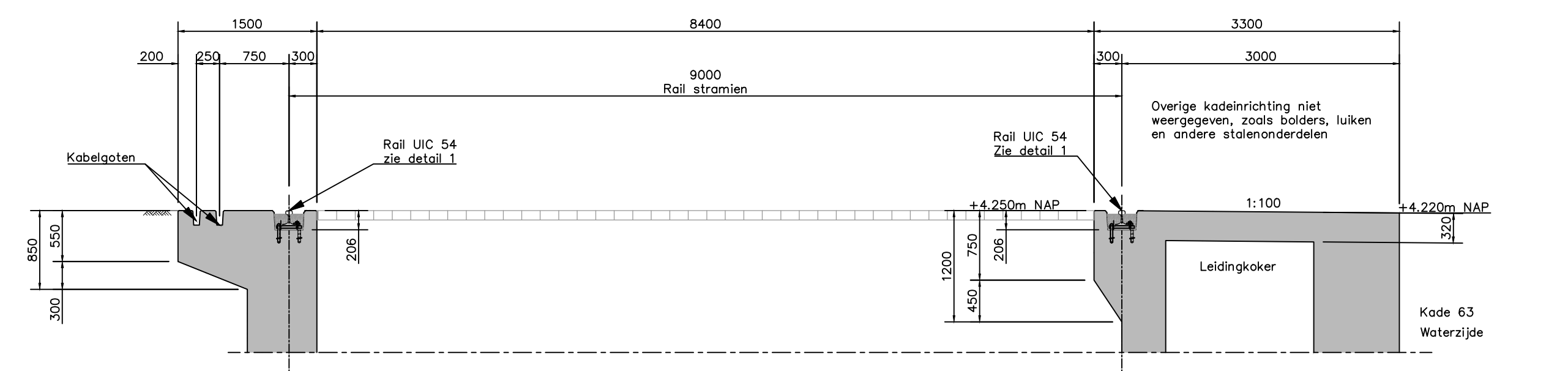
Principedoorsnede Kade 63 Schaal 1:50
