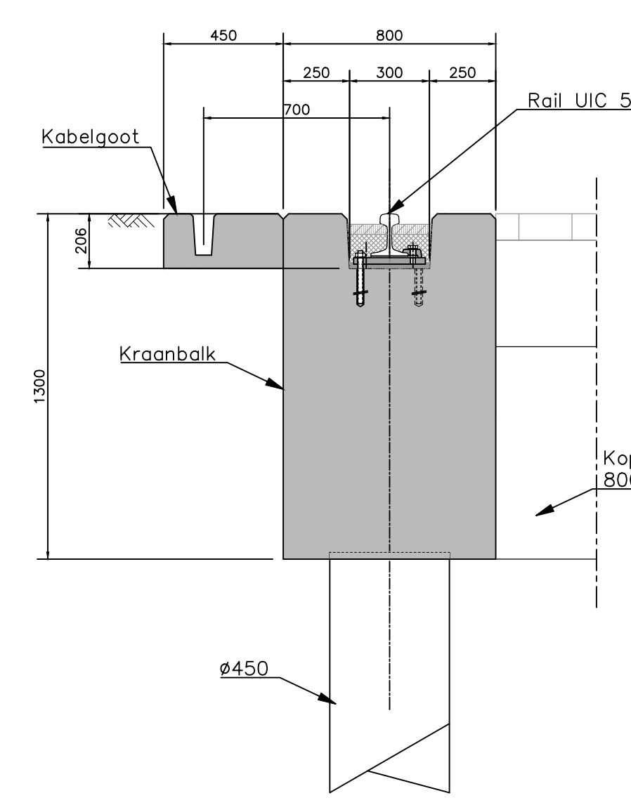
Detail 2: kraanbalk Schaal 1:20
