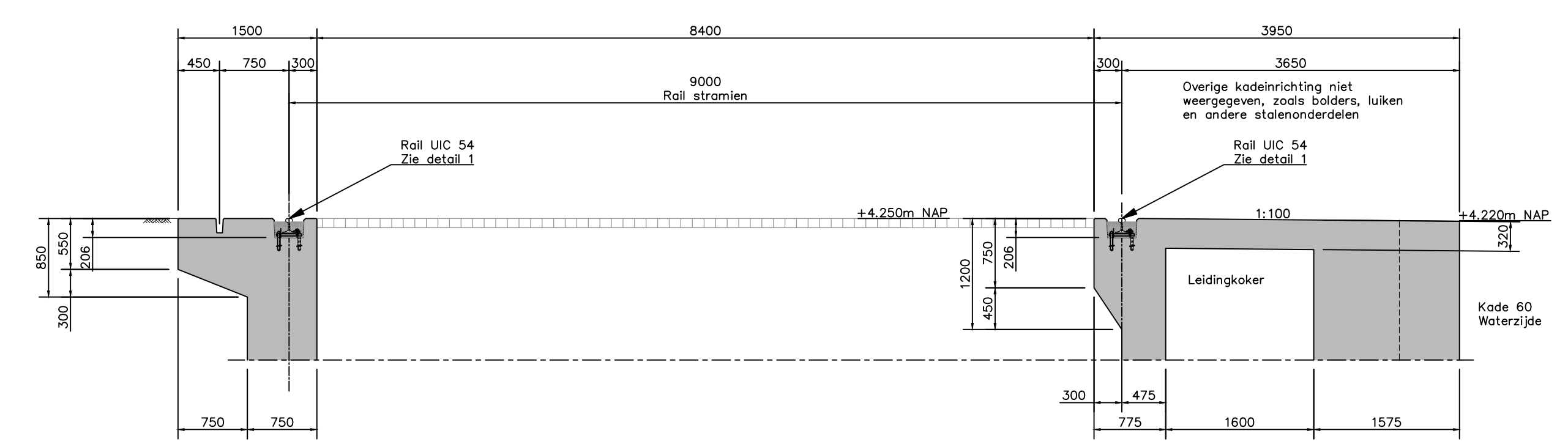
Principedoorsnede Kade 60 Schaal 1:50
