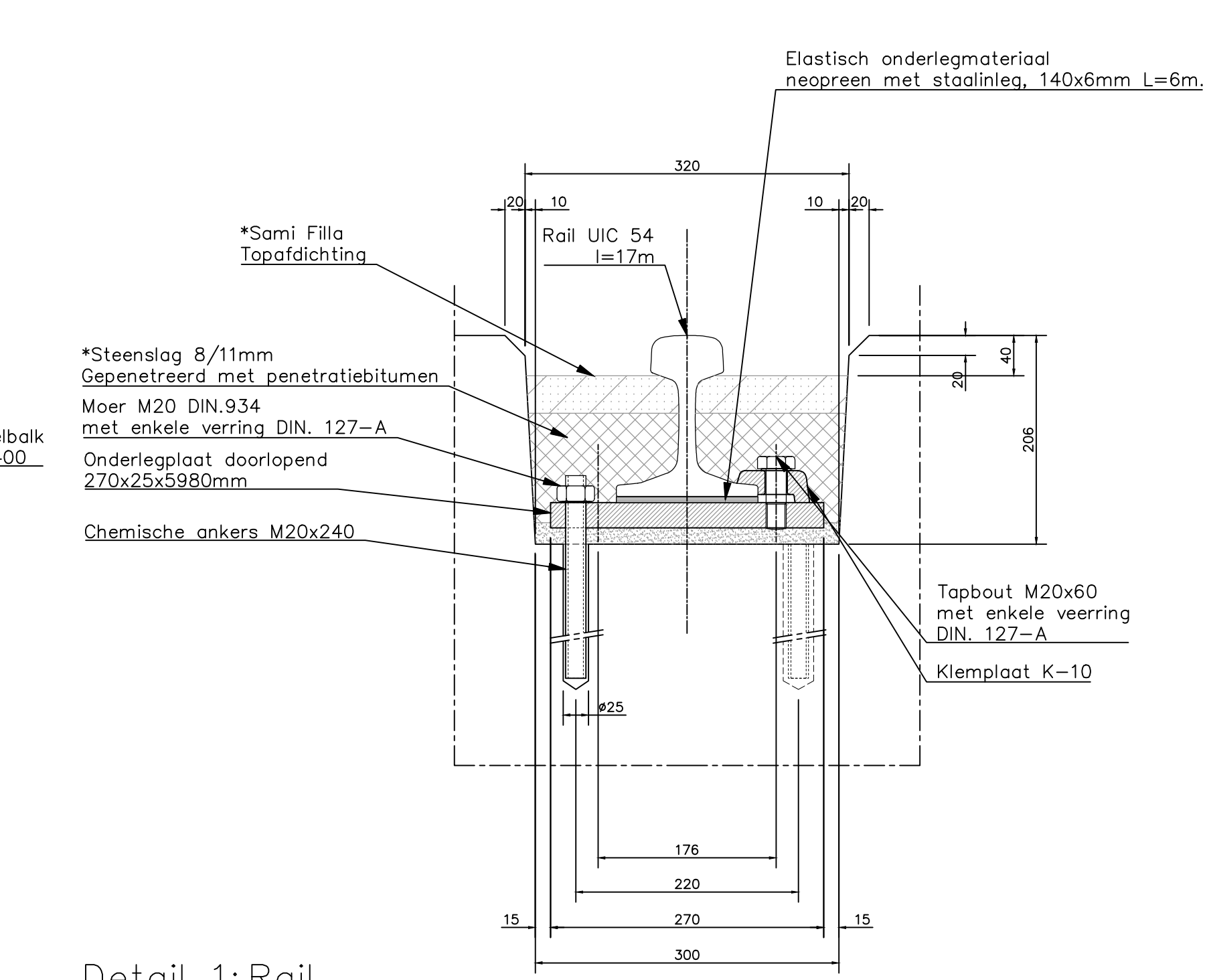
Detail 1: Rail Schaal 1:5 *Oortuiling gedeeltelijk verwijderd
