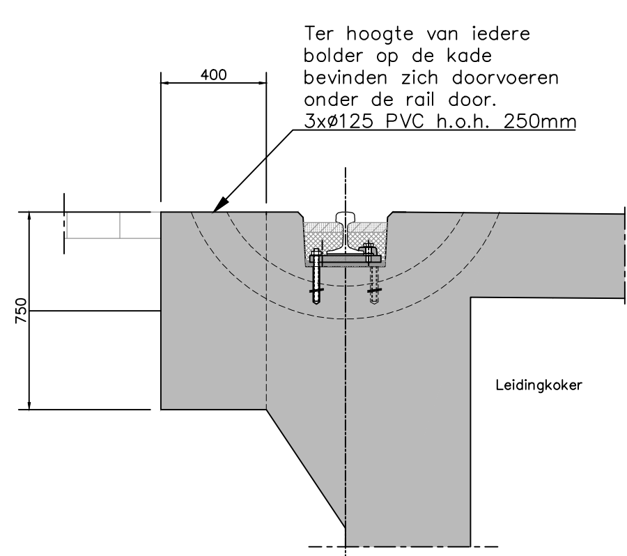
Detail 2: Doorvoeren Schaal 1:20
