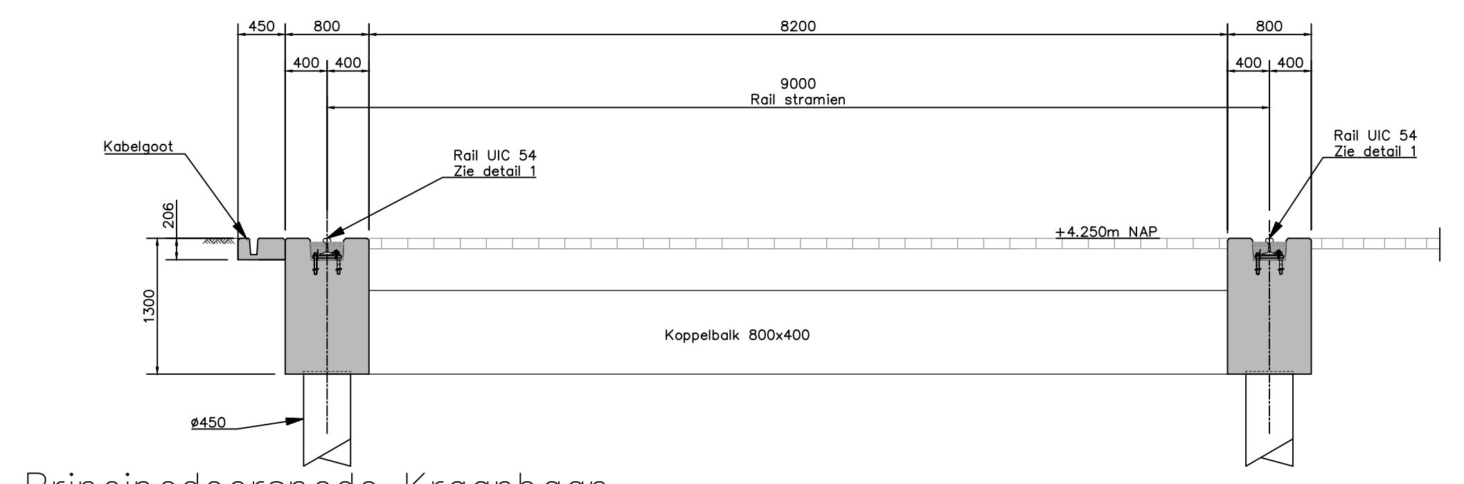
Principedoorsnede Kraanbaan Schaal 1:50
