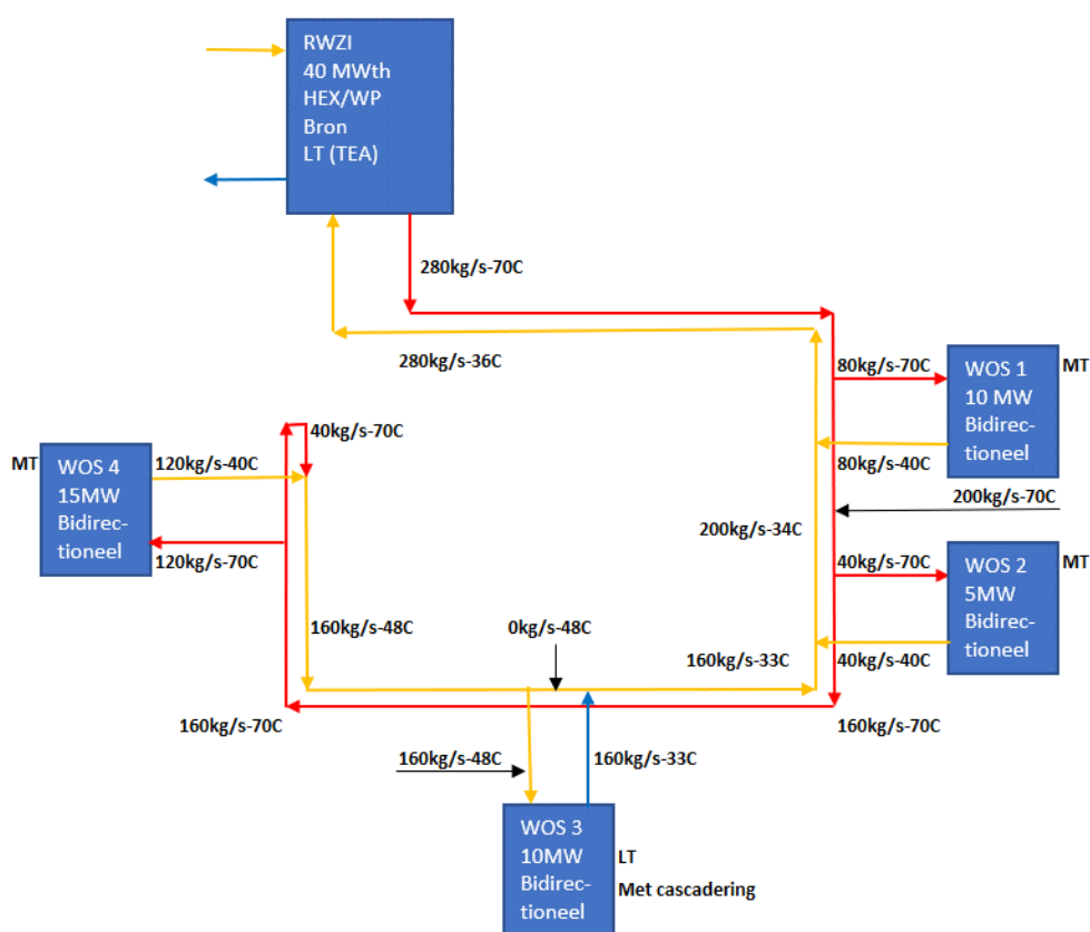
Figuur 24: Open rotonde met cascadering en secundaire pompen
