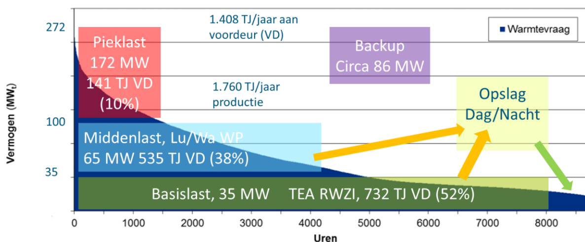
Figuur 13: Jaarduurcurve warmtevraag en de invulling met verschillende soorten warmtebronnen leidend tot een bronnenstrategie voor de warmterotonde
