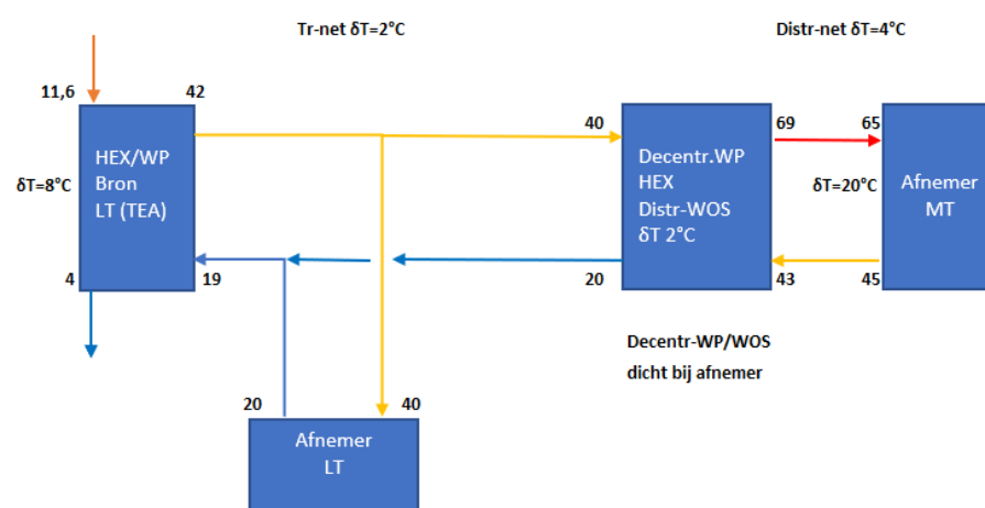
Figuur 21: Principeschema van LT-net met decentrale opwaardering naar MT-warmte
