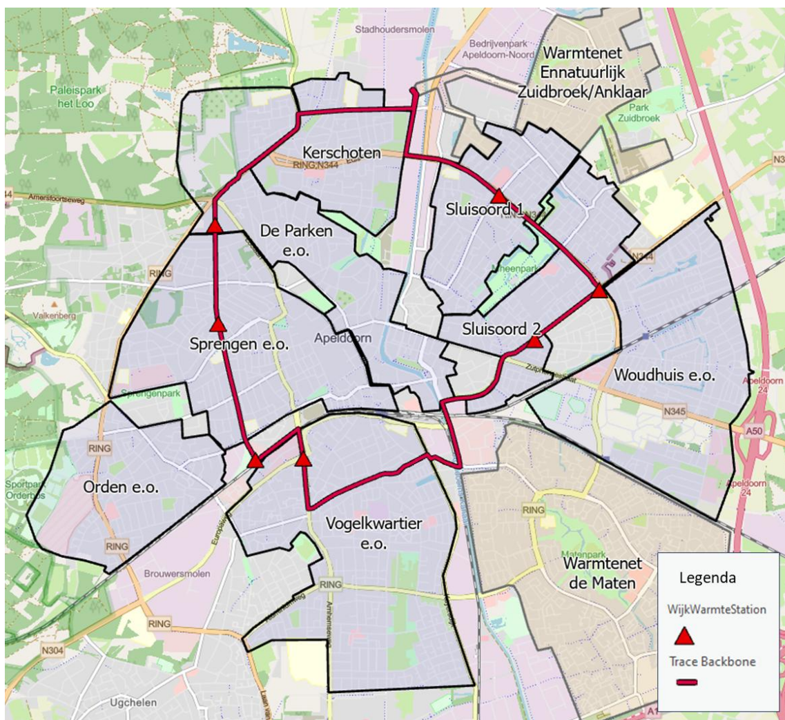
Figuur 27: Schetsontwerp van de warmterotonde infrastructuur in de stad Apeldoorn inclusief de aanpassingen naar aanleiding van de sessie ruimtelijke implicaties WRA. De rode driehoeken zijn mogelijke locaties voor de wijkwarmtestations. Noot: Het voorgestelde tracé en de locaties voor de wijkwarmtestations zijn indicatief. Nader onderzoek moet uitwijzen hoeveel ruimte nodig en beschikbaar is
