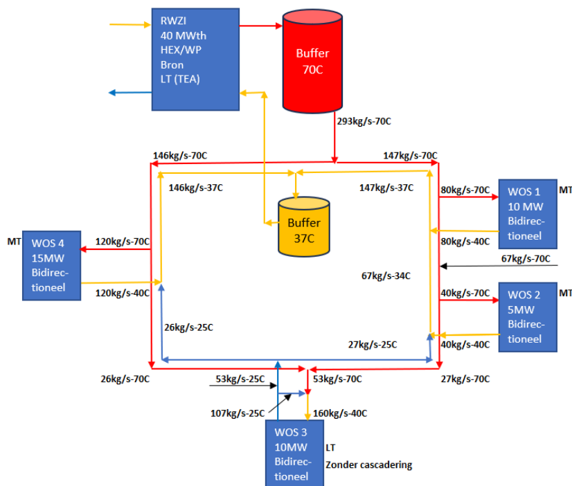
Figuur 26: Gesloten systeem zonder cascadering
