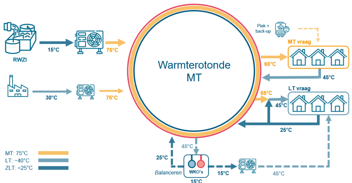
Figuur 19: Principeschema van de warmterotonde, basisvariant
