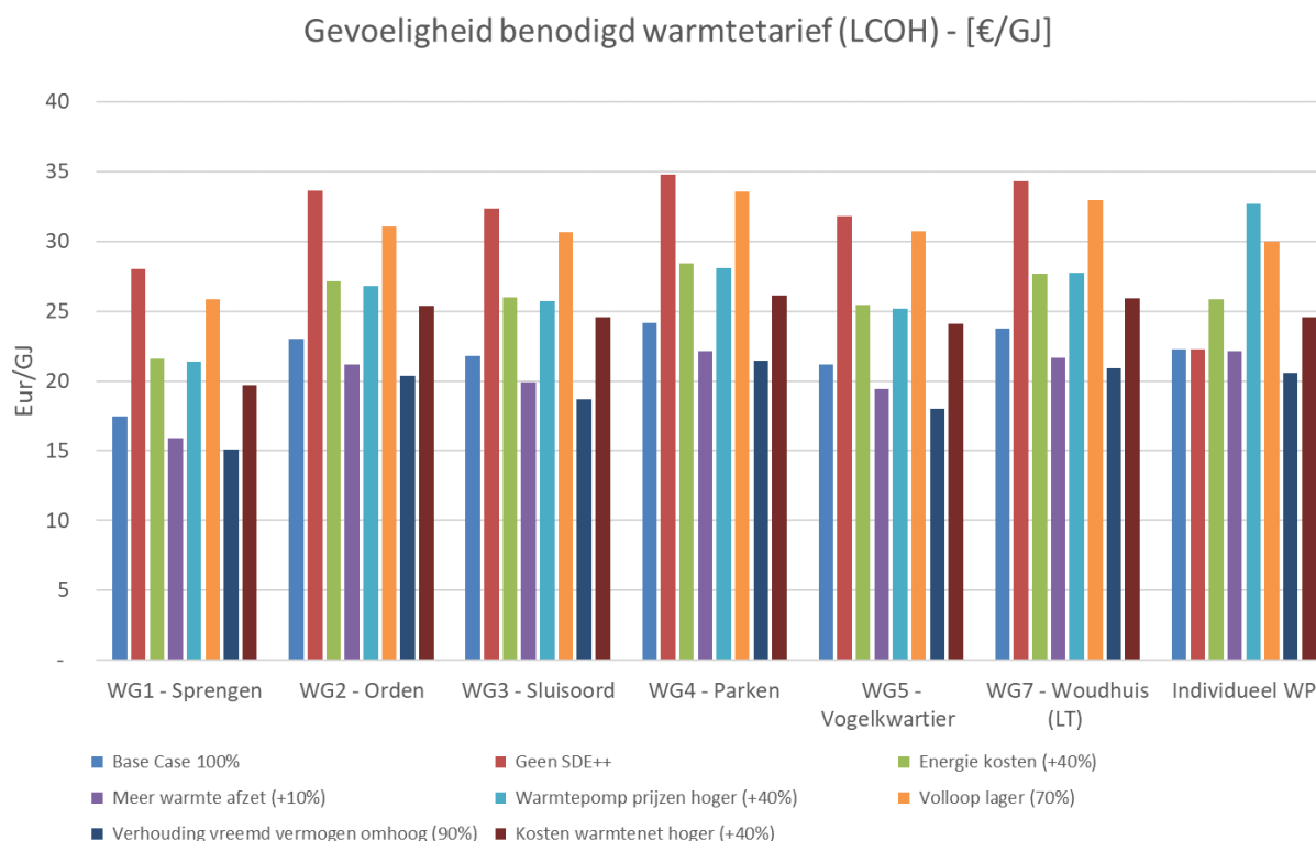
Figuur 40: Gevoeligheidsanalyse op benodigd warmtetarief (LCOH)
