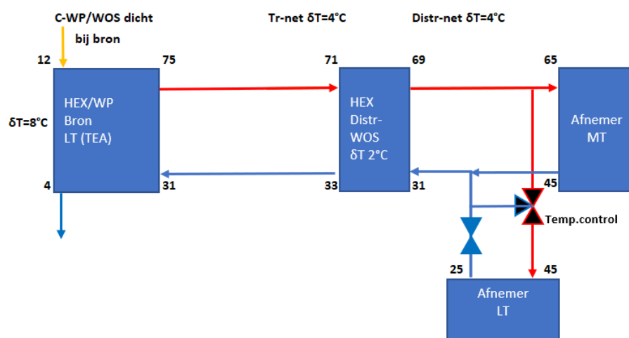
Figuur 20: Principeschema van MT-net met daarnaast mogelijkheid van levering LT-warmte
