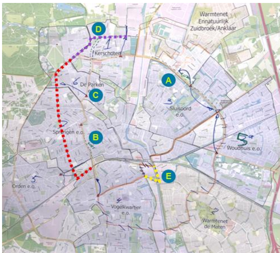
Figuur 28: Visuele weergave van de besproken aanpassingen voor het tracé en de wijkwarmtestations van de warmteronde
