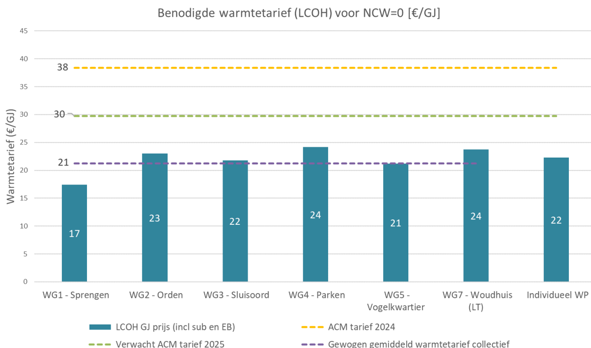
Figuur 39: Benodigd warmtetarief (LCOH) voor NCW = 0 (netto contante waarde). Bij een BAK van € 5.600 en alle relevantie subsidies meegenomen
