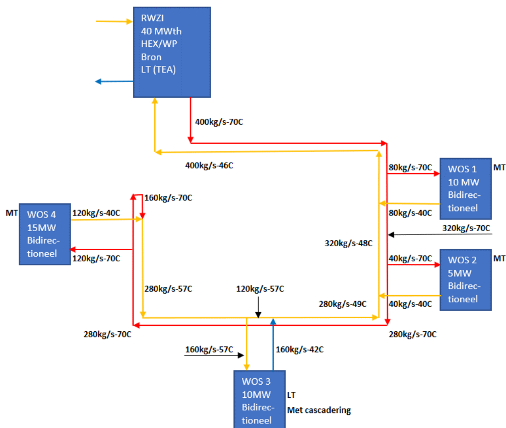
Figuur 23: Open rotonde met cascadering
