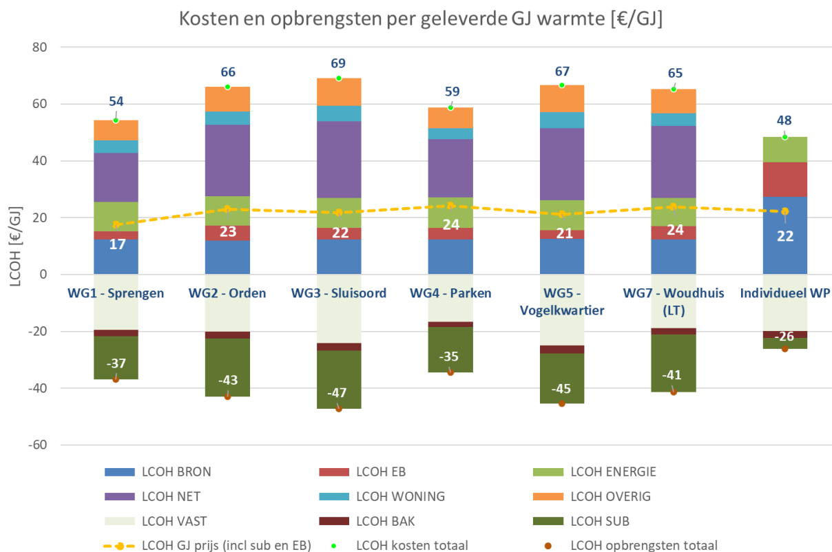
Figuur 38: Kosten en opbrengsten per geleverde GJ aan warmte [€/GJ]
