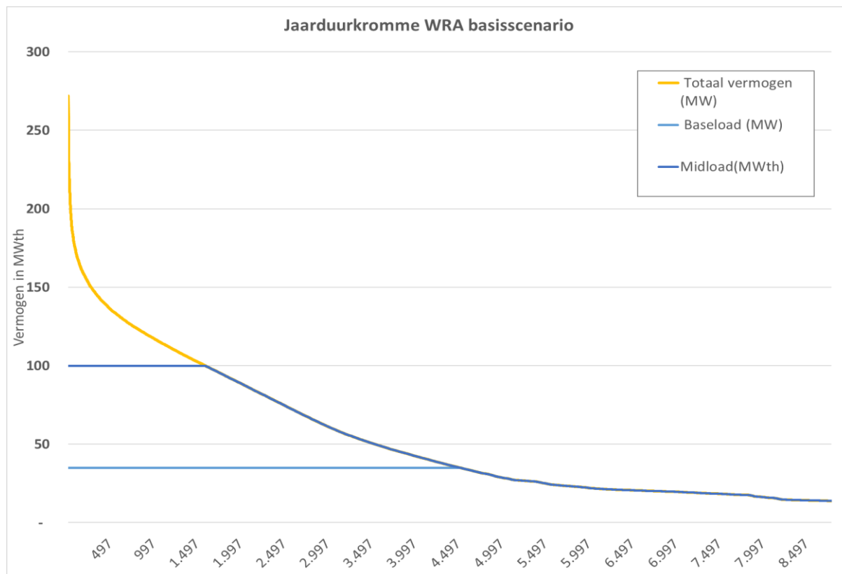
Figuur 12: Jaarduurkromme op basis van de totale warmtevraag voor de gehele warmteronde. Gebruikte uitgangspunten: warmtevraag o.b.v. MT-ready, afname warmtevraag 10%, Volloopgraad warmtenet 90%, warmteverliezen 20%
