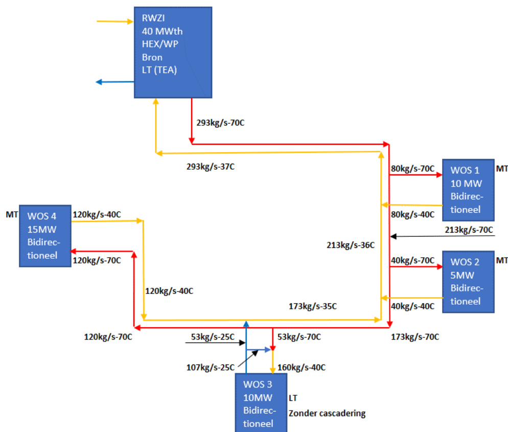
Figuur 25: Open rotonde zonder cascadering
