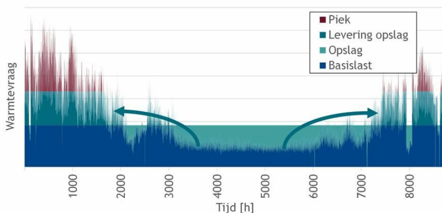
Figuur 17: Voorbeeld van het inpassen van een HTO op basis van de warmtevraag door het jaar heen. Warmteoverschot in de zomer wordt opgeslagen in de HTO om vervolgens in koude perioden te worden ingezet
