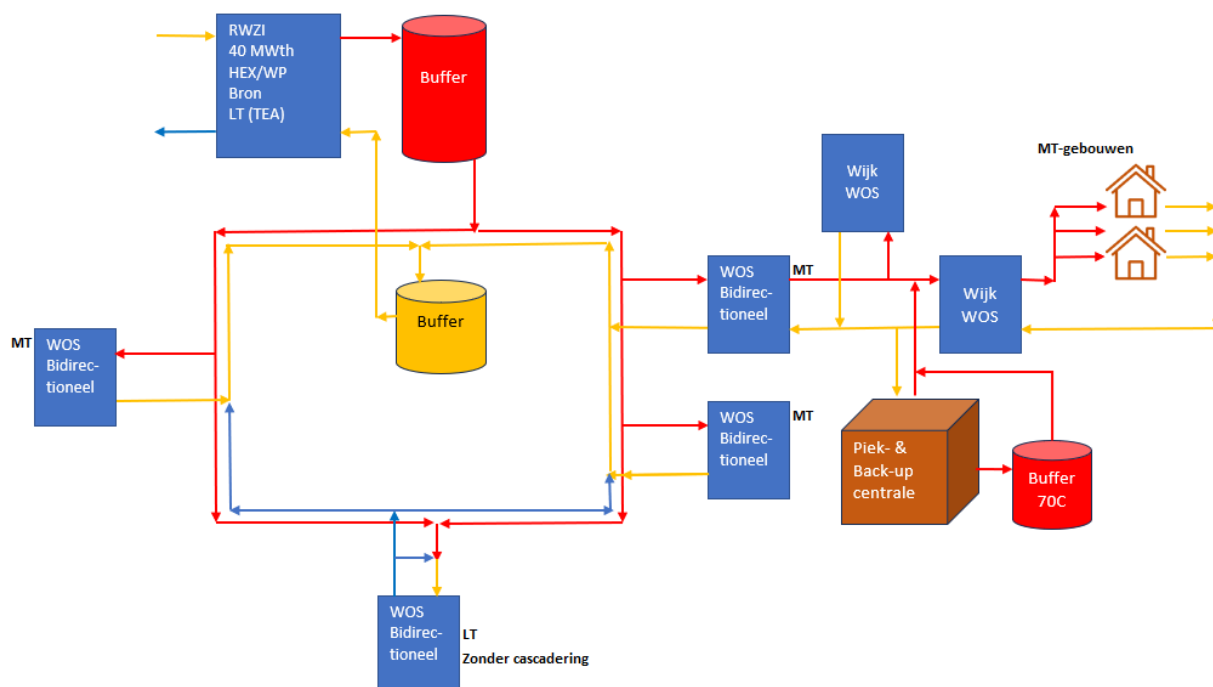
Figuur 29: Integraal schematisch overzicht van de warmterotonde
