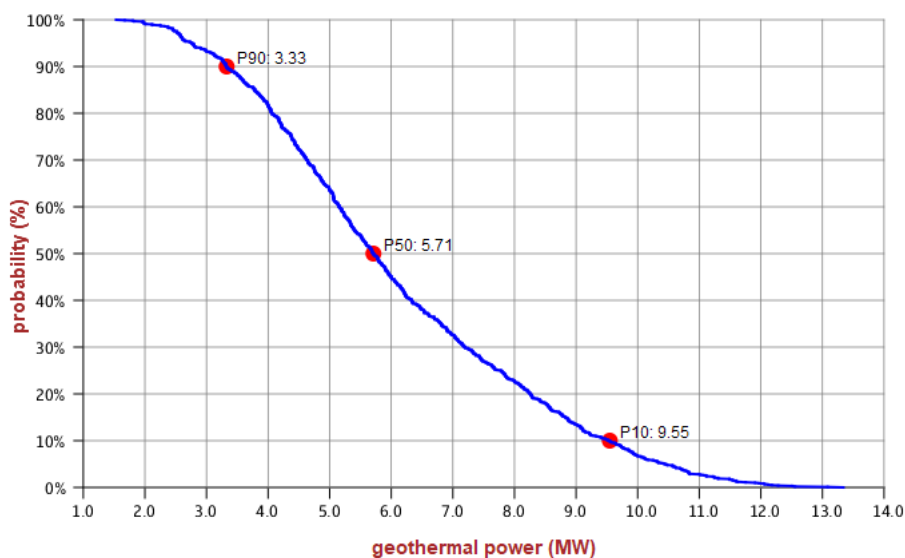
Figuur 8.6 | Waarschijnlijkheidsverdeling van het thermisch vermogen van het geothermiedoublet in de Formatie van Slochteren op locatie 5.
