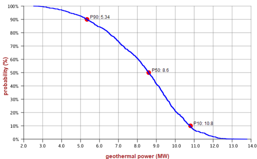
Figuur 8.3 | Waarschijnlijkheidsverdeling van het thermisch vermogen van het geothermiedoublet in de Formatie van Slochteren op locatie 2.
