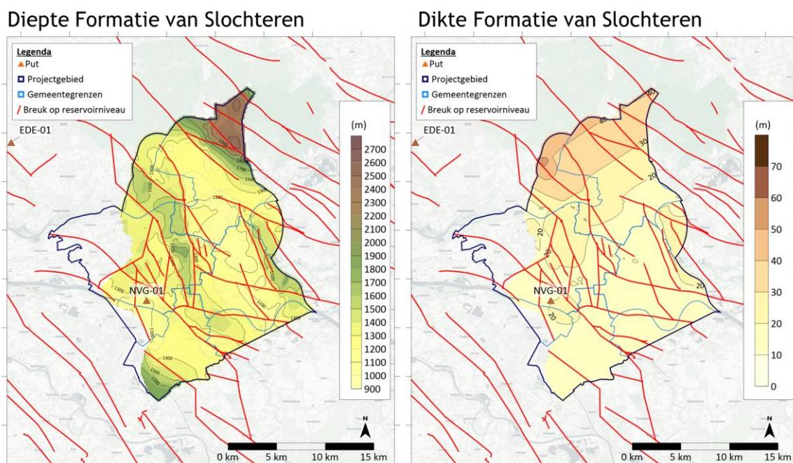
Figuur 4.1 | Links) diepte van de Formatie van Slochteren. Rechts) dikte van de Formatie van Slochteren.
