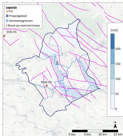
Figuur 5.3 | Boven) Base case doorlatendheid van de Hoofd Bontzandsteen Subgroep (begravingsanomalie + 0 m). Links onder) Low case doorlatendheid van de Hoofd-Bontzandsteen Subgroep (begravingsanomalie + 300 m). Rechts onder) High case doorlatendheid van de Hoofd-Bontzandsteen Subgroep (begravingsanomalie - 300 m).
