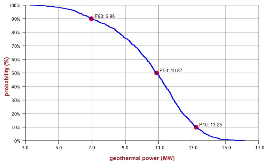
Figuur 8.5 | Waarschijnlijkheidsverdeling van het thermisch vermogen van het geothermiedoublet in de Formatie van Slochteren op locatie 4.
