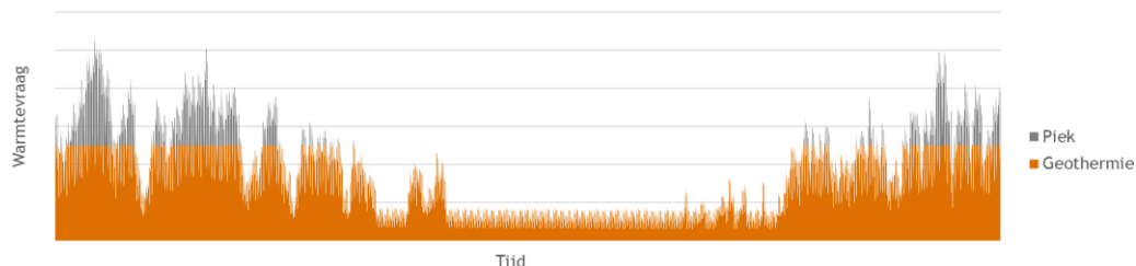
Figuur 8.9 | Een typisch warmtevraag van een warmtenet in de gebouwde omgeving.
