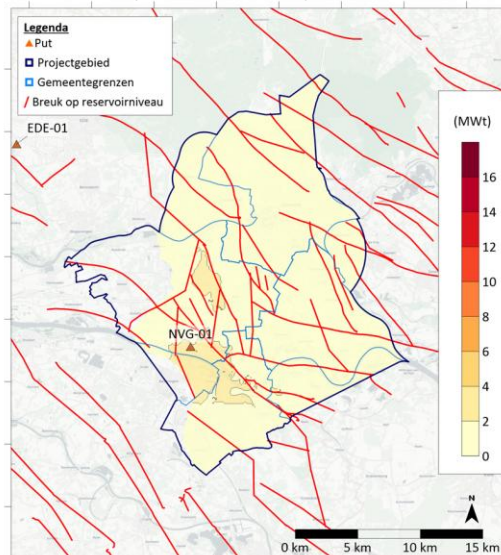
Figuur 4.4 | Boven) Base case potentie (MWt) van de Formatie van Slochteren (begravingsanomalie + 0 m). Links onder) Low case potentie (MWt) van de Formatie van Slochteren (begravingsanomalie + 300 m). Rechts onder) High case potentie van de Formatie van Slochteren (begravingsanomalie -300 m).
