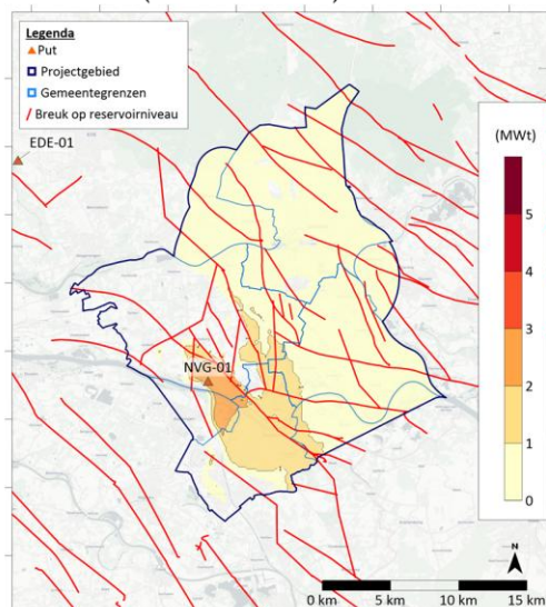
Figuur 6.4 | Boven) Base case potentie (MWt) van de Nederweert Zandsteen Formatie (begravingsanomalie + 0 m). Links onder) Low case potentie (MWt) van de Nederweert Zandsteen Formatie (begravingsanomalie + 300 m). Rechts onder) High case potentie van de Nederweert Zandsteen Formatie (begravingsanomalie -300 m).
