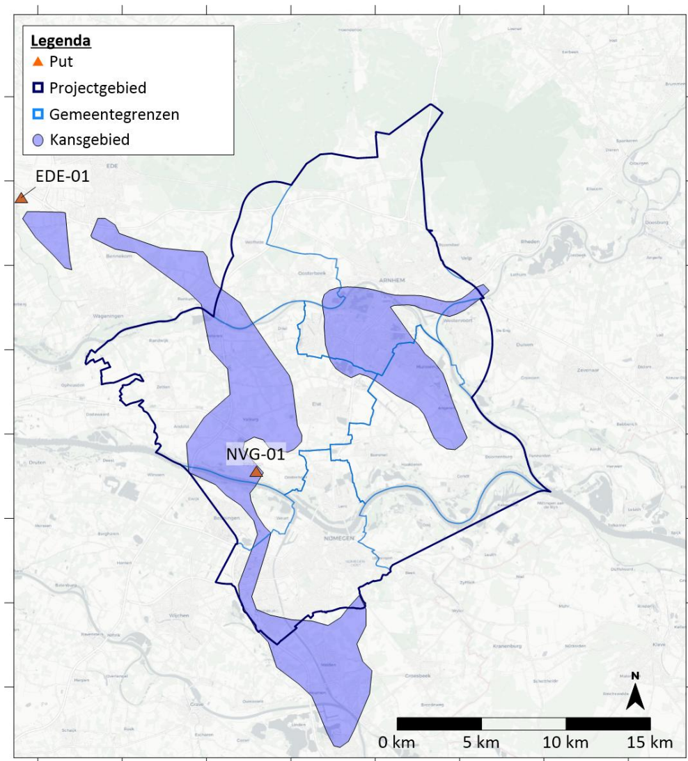
Figuur 7.2 | Kansgebieden binnen het Z1 Randcarbonaat waar mogelijke karstvorming heeft plaatsgevonden.
