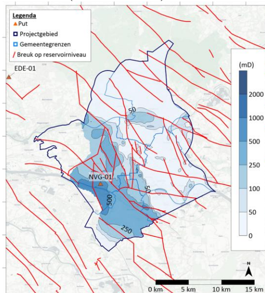
Figuur 4.3 | Boven) Base case doorlatendheid van de Formatie van Slochteren (begravingsanomalie + 0 m). Links onder) Low case doorlatendheid van de Formatie van Slochteren (begravingsanomalie + 300 m). Rechts onder) High case doorlatendheid van de Formatie van Slochteren (begravingsanomalie - 300 m).
