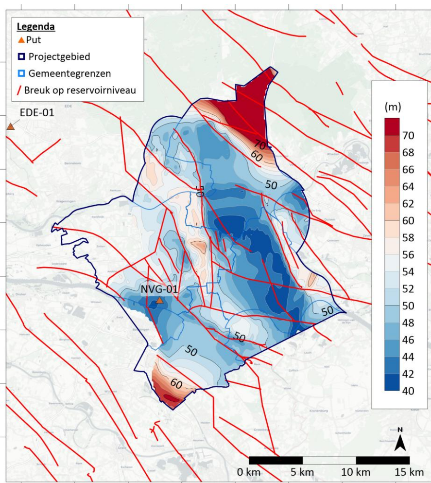
Figuur 6.2 | Temperatuur van de Nederweert Zandsteen Formatie.
