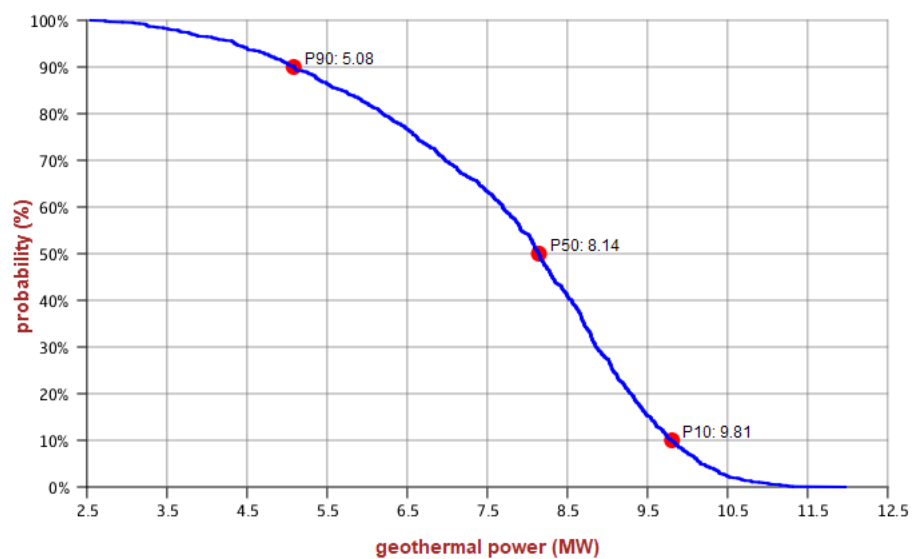
Figuur 8.4 | Waarschijnlijkheidsverdeling van het thermisch vermogen van het geothermiedoublet in de Formatie van Slochteren op locatie 3.
