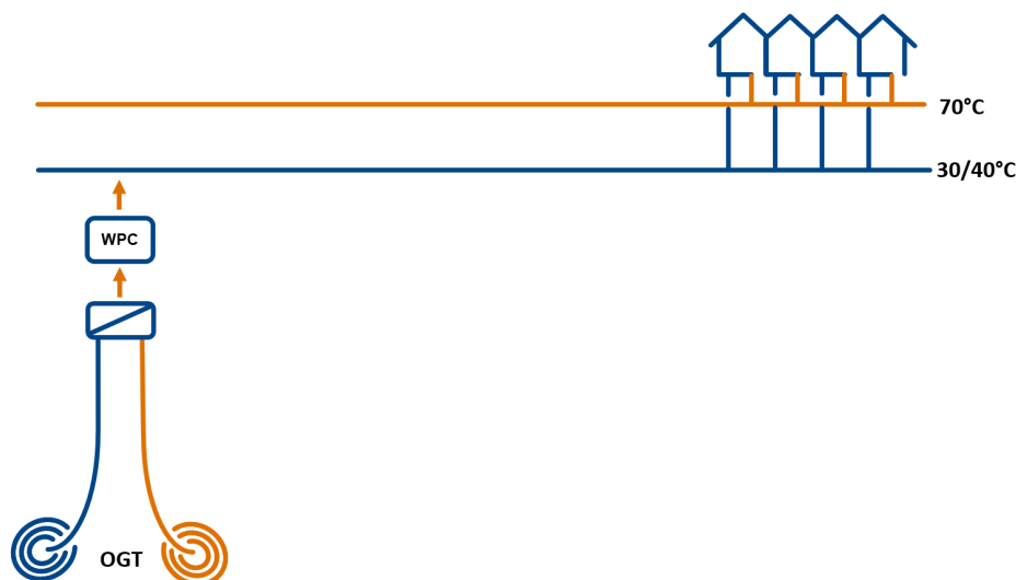
Figuur 8.7 | Schematische weergave systeemconcept basisvariant (WPC = warmtepompcentrale, OGT is ondiepe geothermie).
