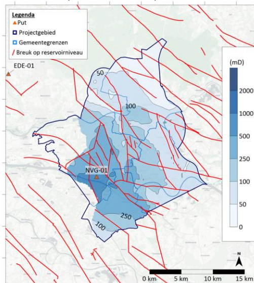
Figuur 6.3 | Boven) Base case doorlatendheid van de Nederweert Zandsteen Formatie (begravingsanomalie + 0 m). Links onder) Low case doorlatendheid van de Nederweert Zandsteen Formatie (begravingsanomalie + 300 m). Rechts onder) High case doorlatendheid van de Nederweert Zandsteen Formatie (begravingsanomalie - 300 m).
