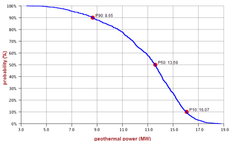
Figuur 8.2 | Waarschijnlijkheidsverdeling van het thermisch vermogen van het geothermiedoublet in de Formatie van Slochteren op locatie 1.
