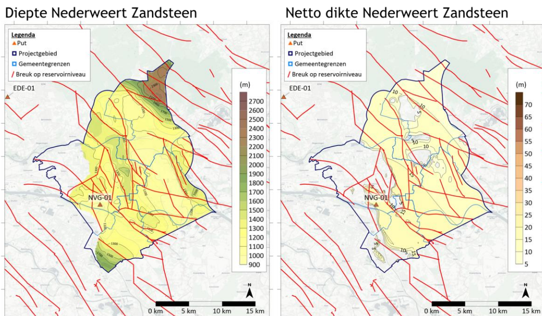
Figuur 6.1 | Links) diepte van de Nederweert Zandsteen Formatie. Rechts) Netto dikte van de Nederweert Zandsteen Formatie.
