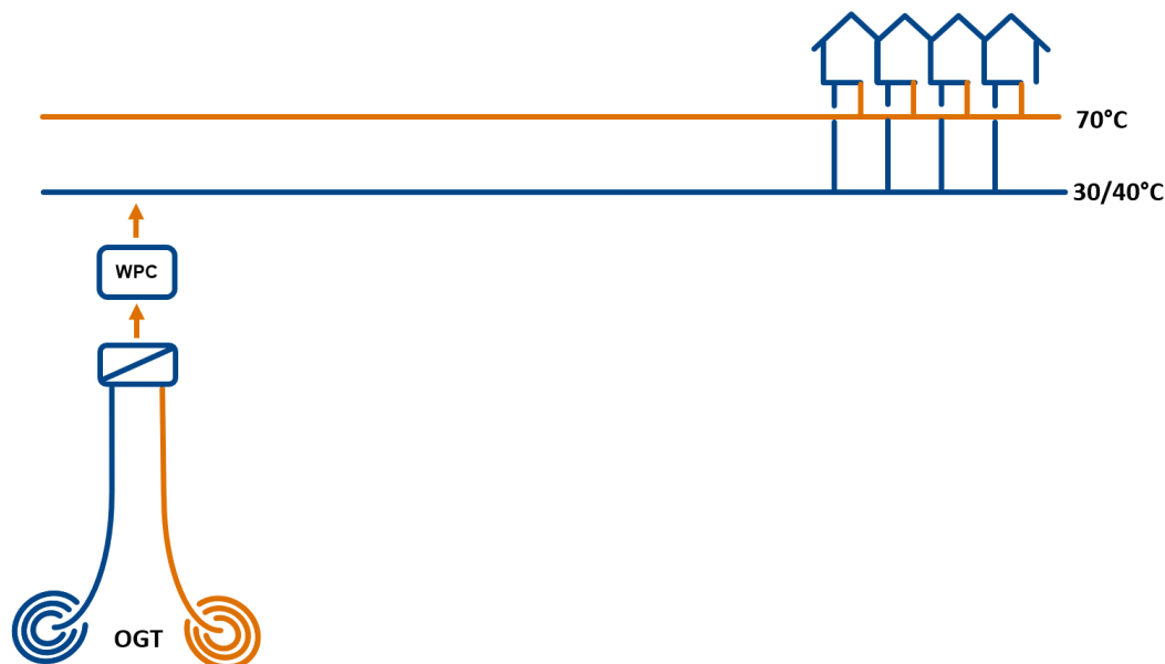
Figuur 8.8 | Schematische weergave systeemconcept (WPC = warmtepompcentrale, OGT = ondiepe geothermie).
