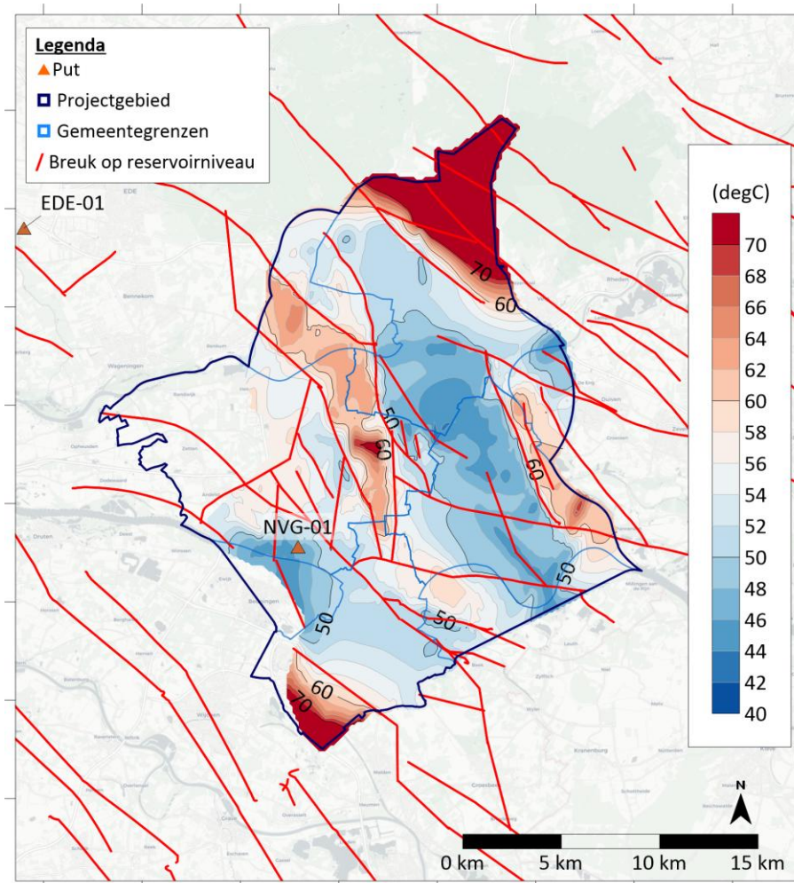
Figuur 4.2 | Temperatuur van de Formatie van Slochteren.
