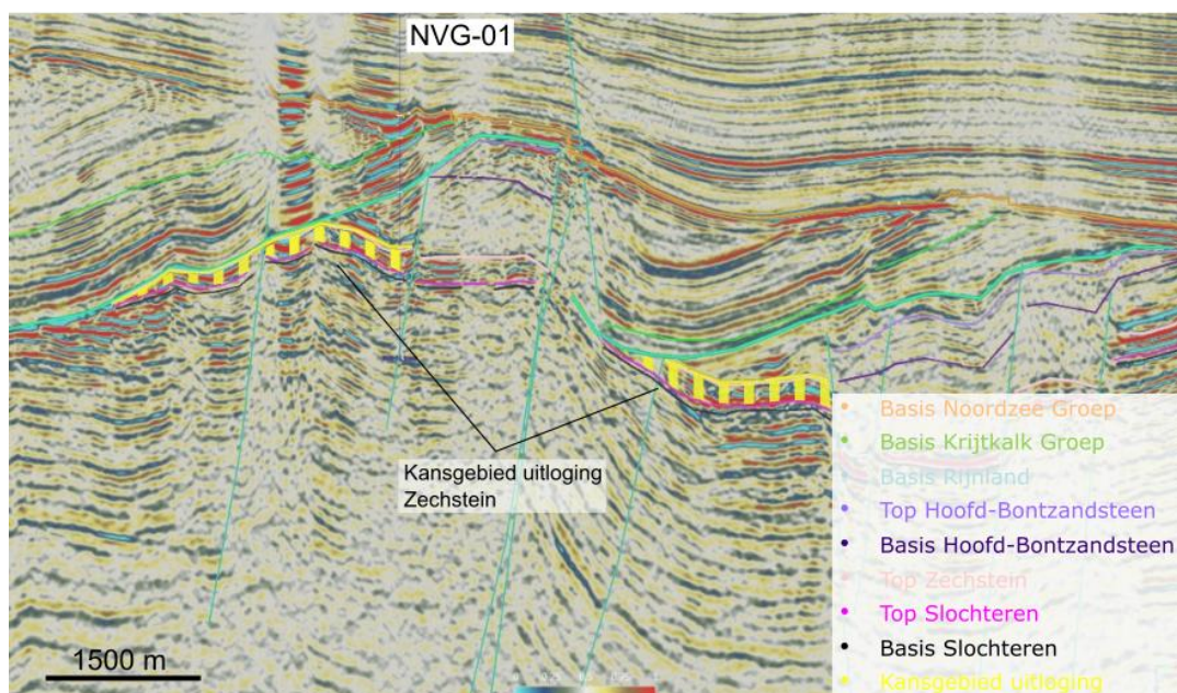
Figuur 7.1 | Seismische sectie waarin een mogelijk uitlogingsgebied van de Zechstein is aangegeven (geel). Op deze locaties ligt de Zechstein direct of vlak onder de basis van de Rijnland Groep.
