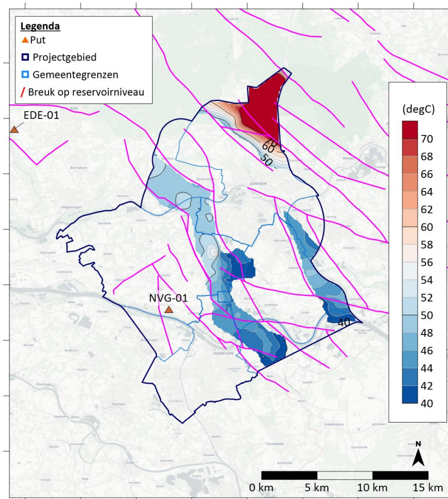
Figuur 5.2 | Temperatuur van de Hoofd-Bontzandsteen Subgroep
