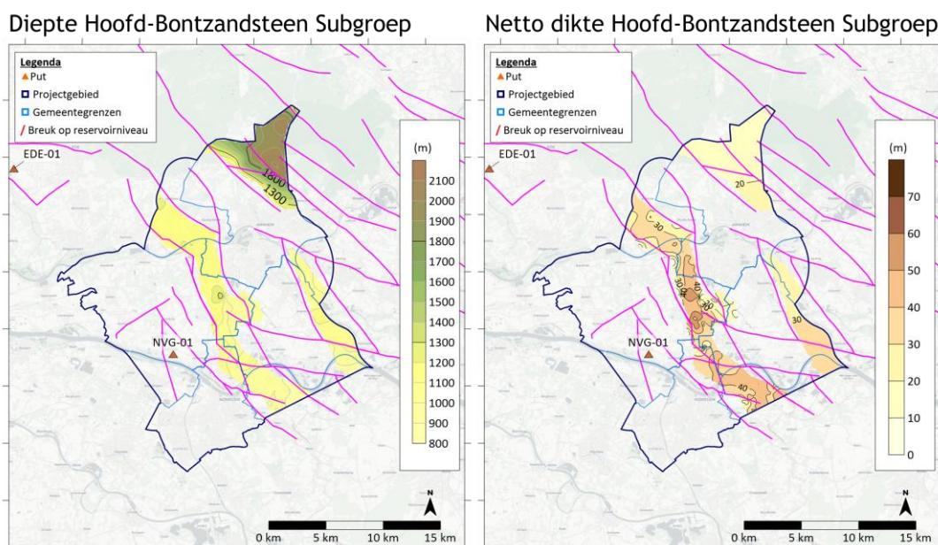
Figuur 5.1 | Links) diepte van de Hoofd-Bontzandsteen Subgroep. Rechts) Netto dikte van de Hoofd-Bontzandsteen Subgroep
