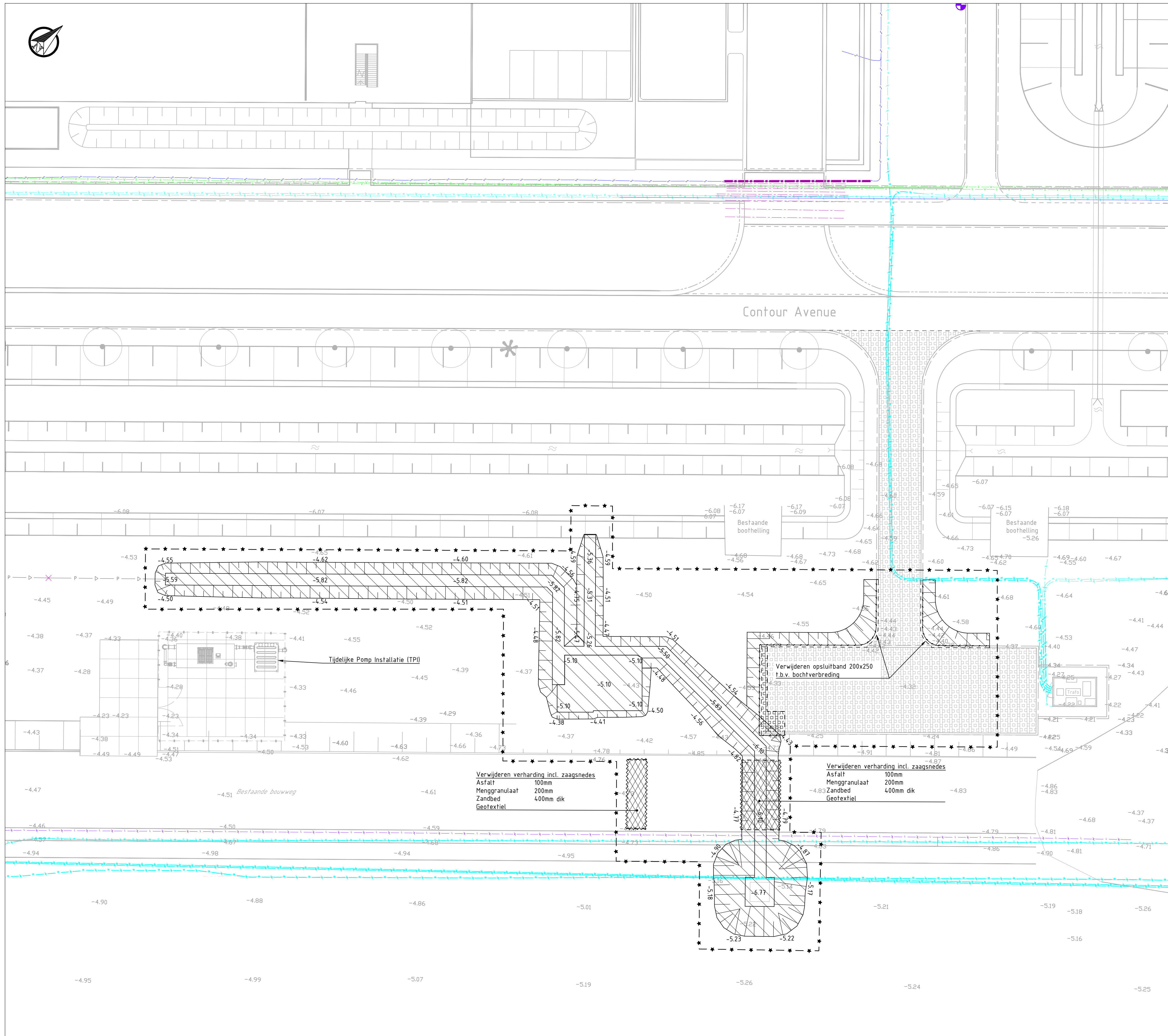
SITUATIE SCHAAL 1 : 200
