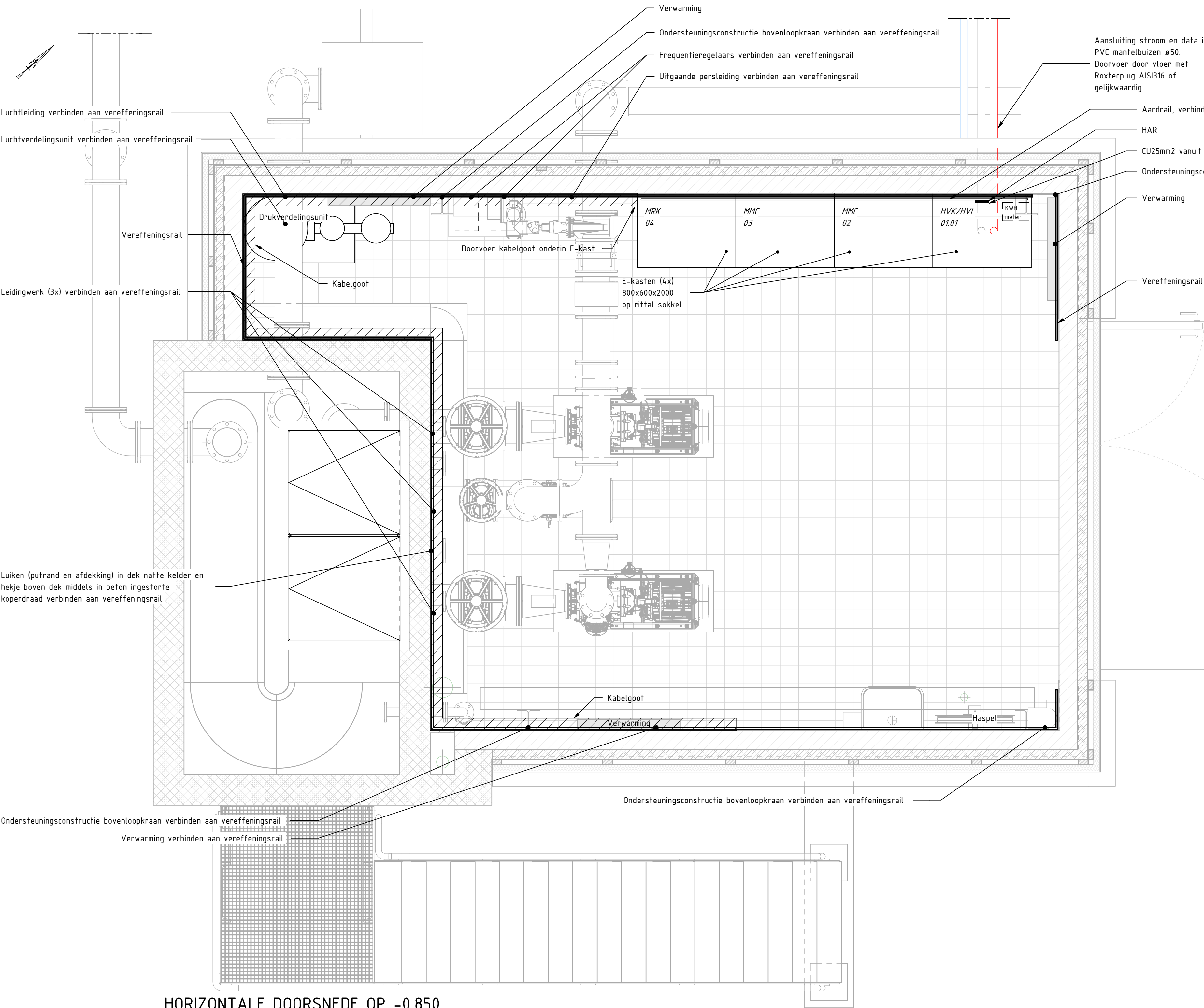
HORizontale Doorsneede op -0.850 schaal: 1 : 20
