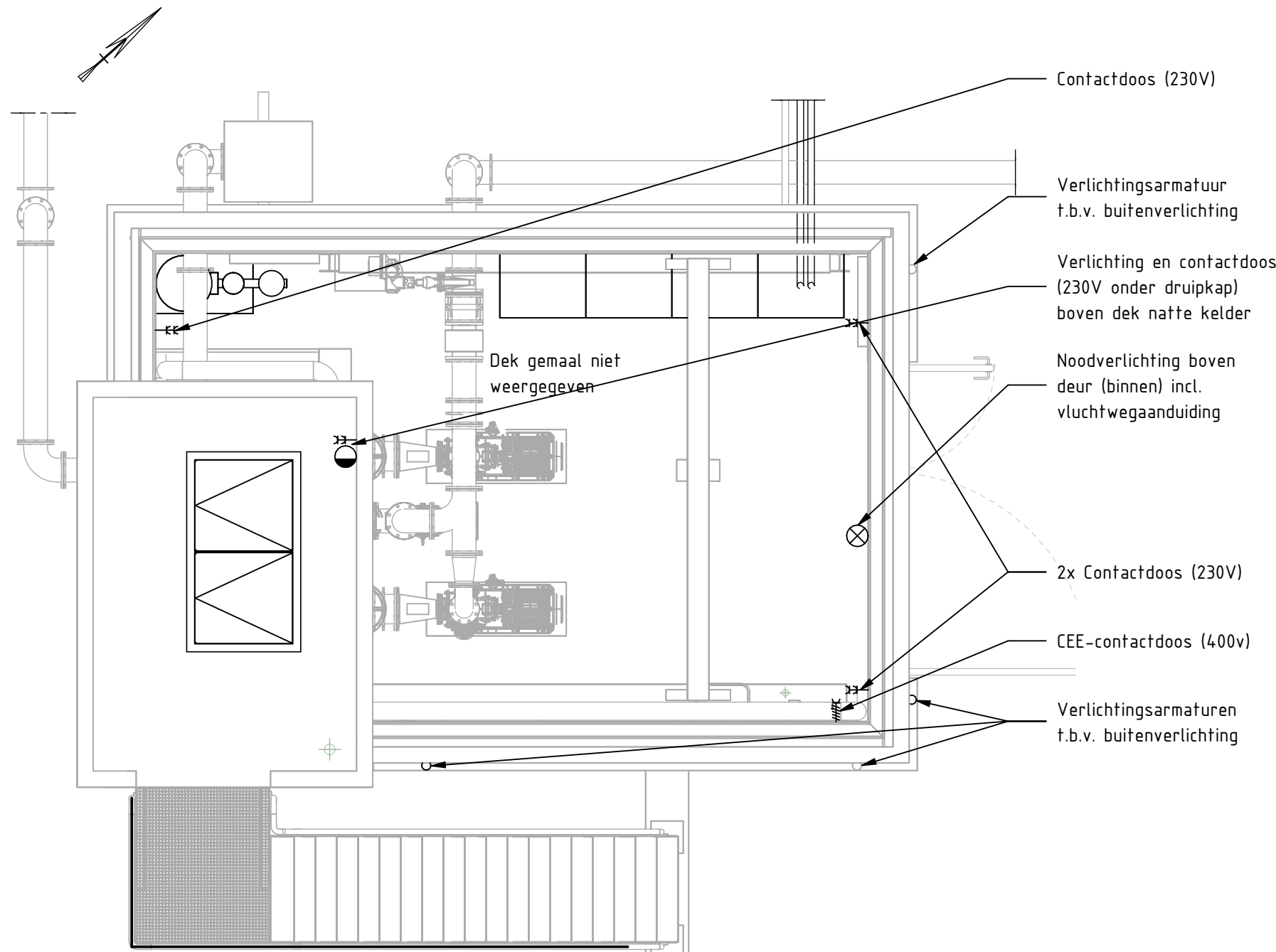
OVERZICHT VERLICHTING EN STROOMPUNTEN schaal: 1 : 50
