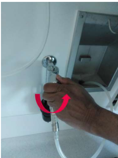
FOTO BIJ A525-52J: Foto 09 Uittrekken Doorspoelslang
