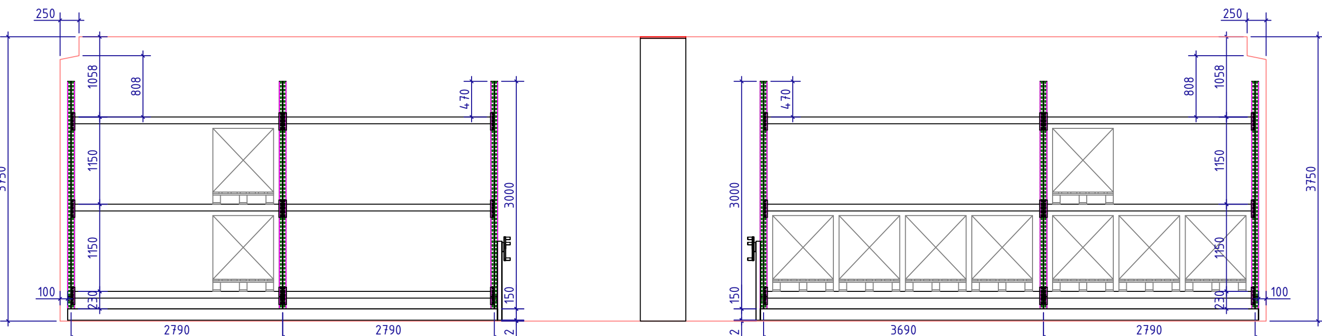
Aanzichten Ruimte D.02.03
