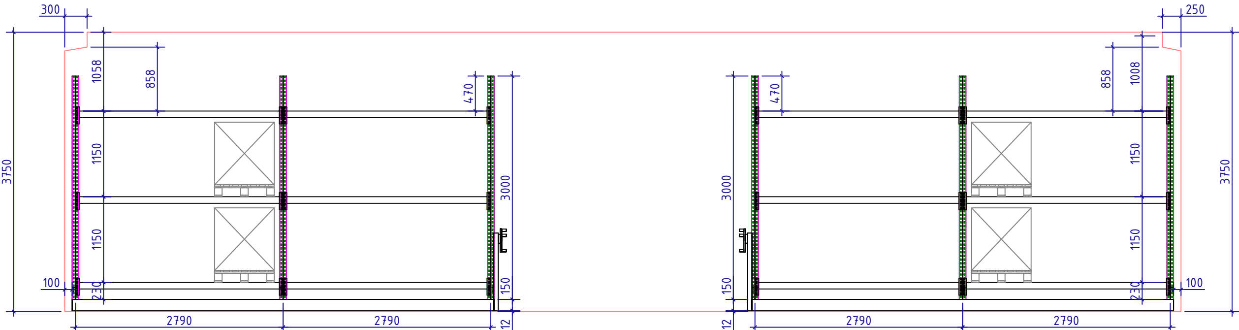
zij aanzicht: Pallet rekken / Pallet rekken
