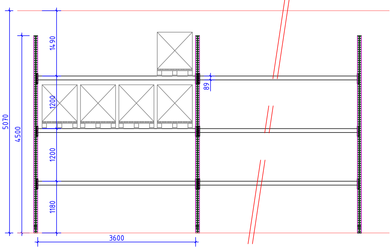
Aanzicht Ruimte D.00.01
