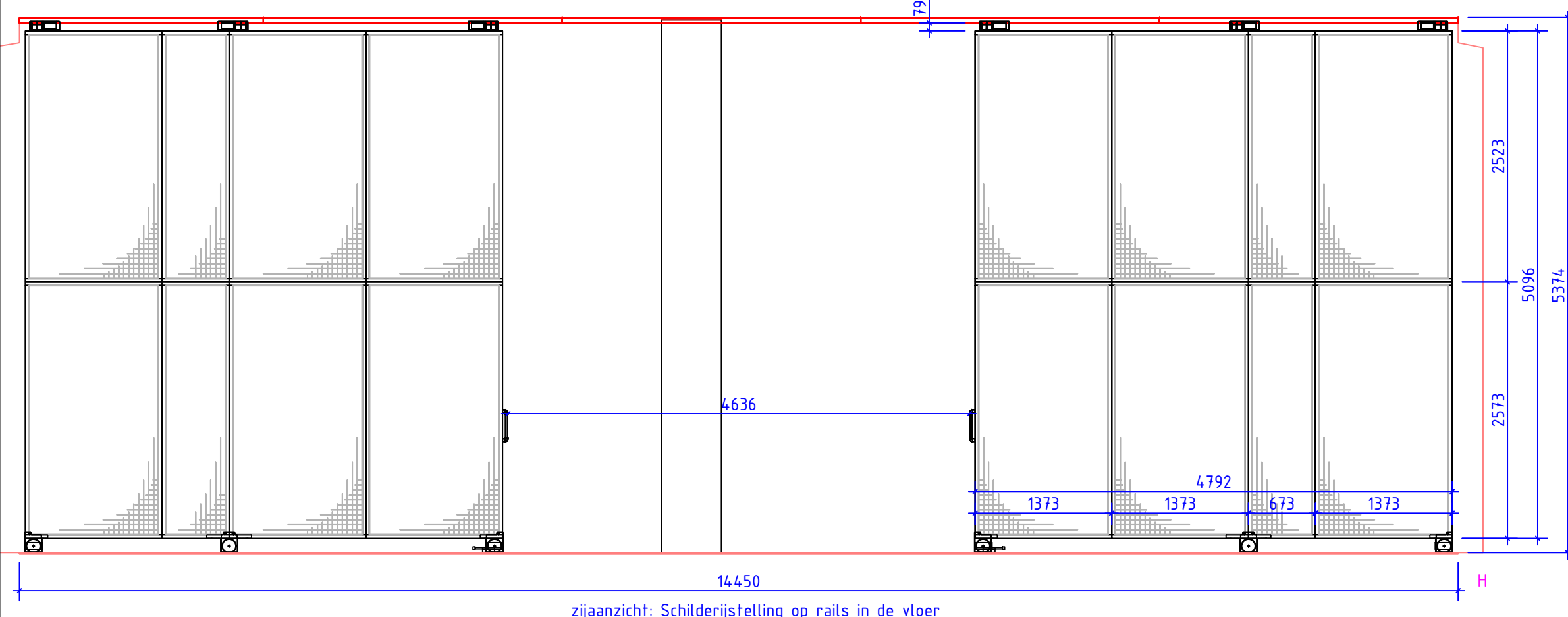
zijaanzicht: Schilderstelling op rails in de vloer
