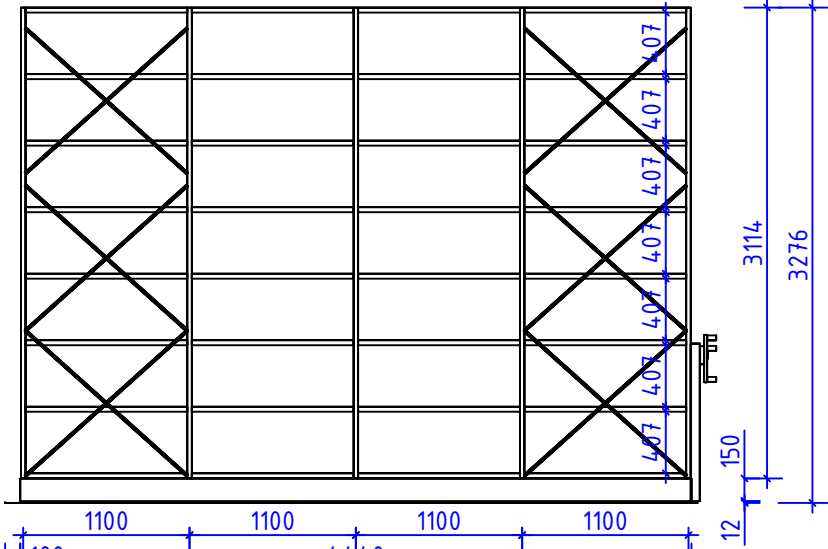
zijaanzicht: legbordsfellingen Quarantaine EG EP
