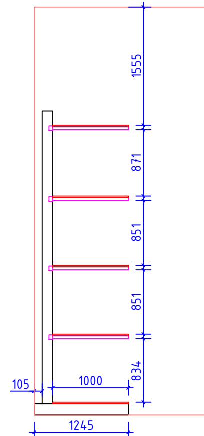
zijaanzicht: statische gaaswand
