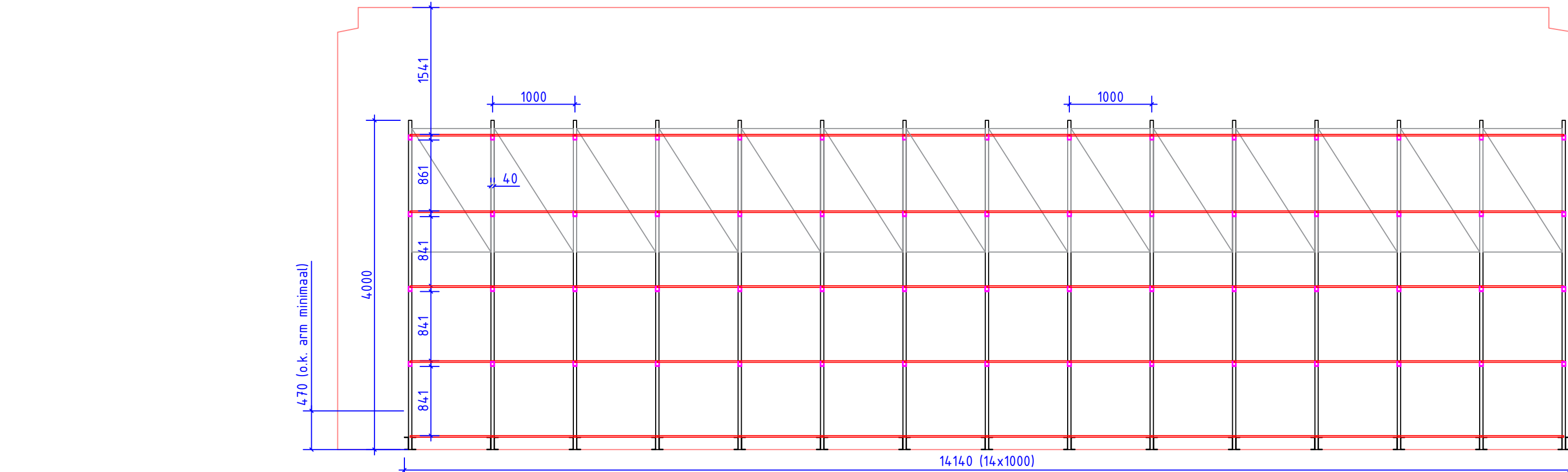
vooraanzicht: draagarmstelling
