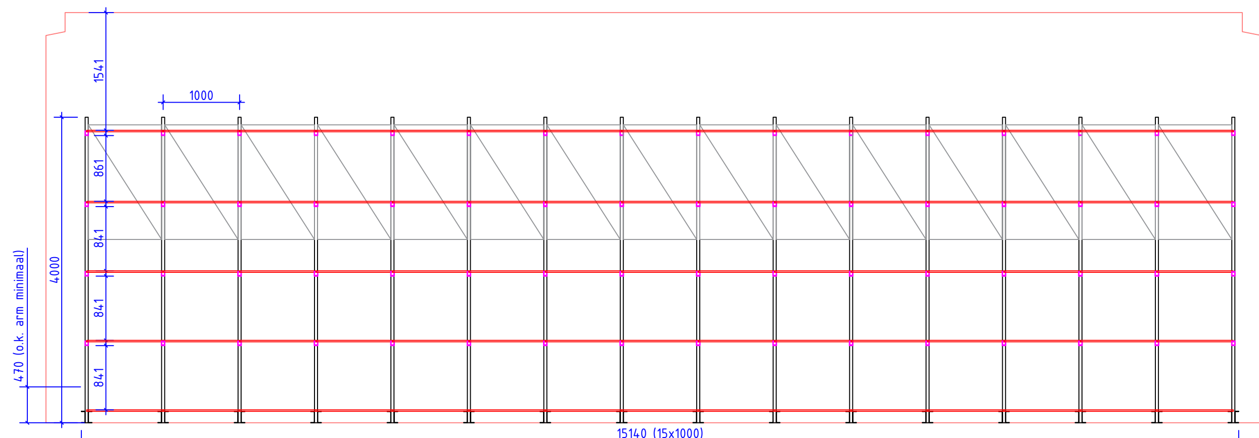
vooraanzicht: draagarmstelling
