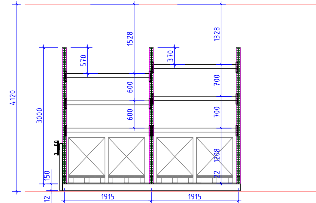
Aanzichten Ruimte S.00.16
