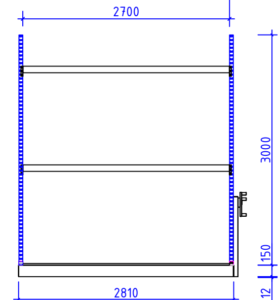
zijaanzicht: breedvak stelling
