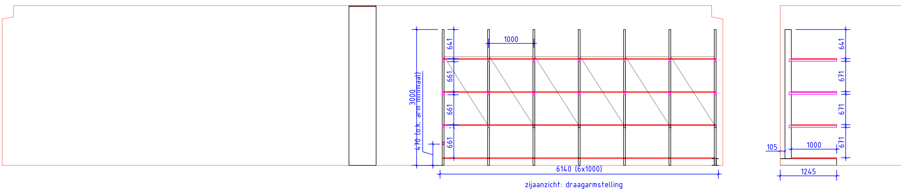
zijaanzicht: draagarmstelling
