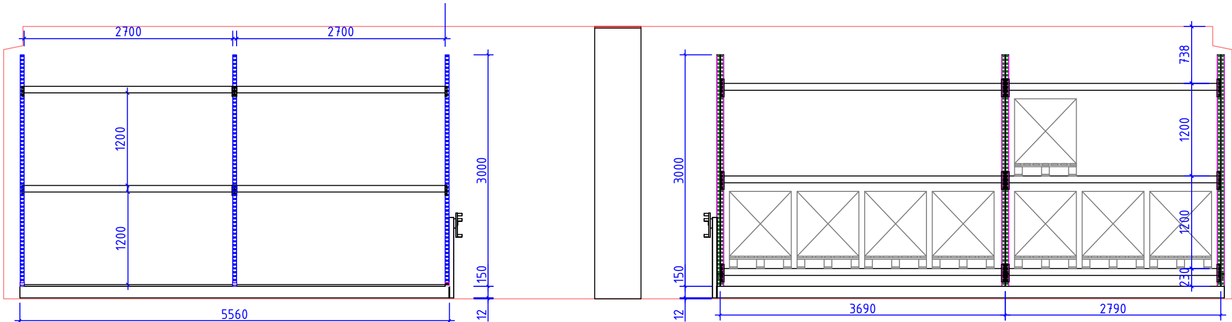
zijaanzicht: breedvak stelling
