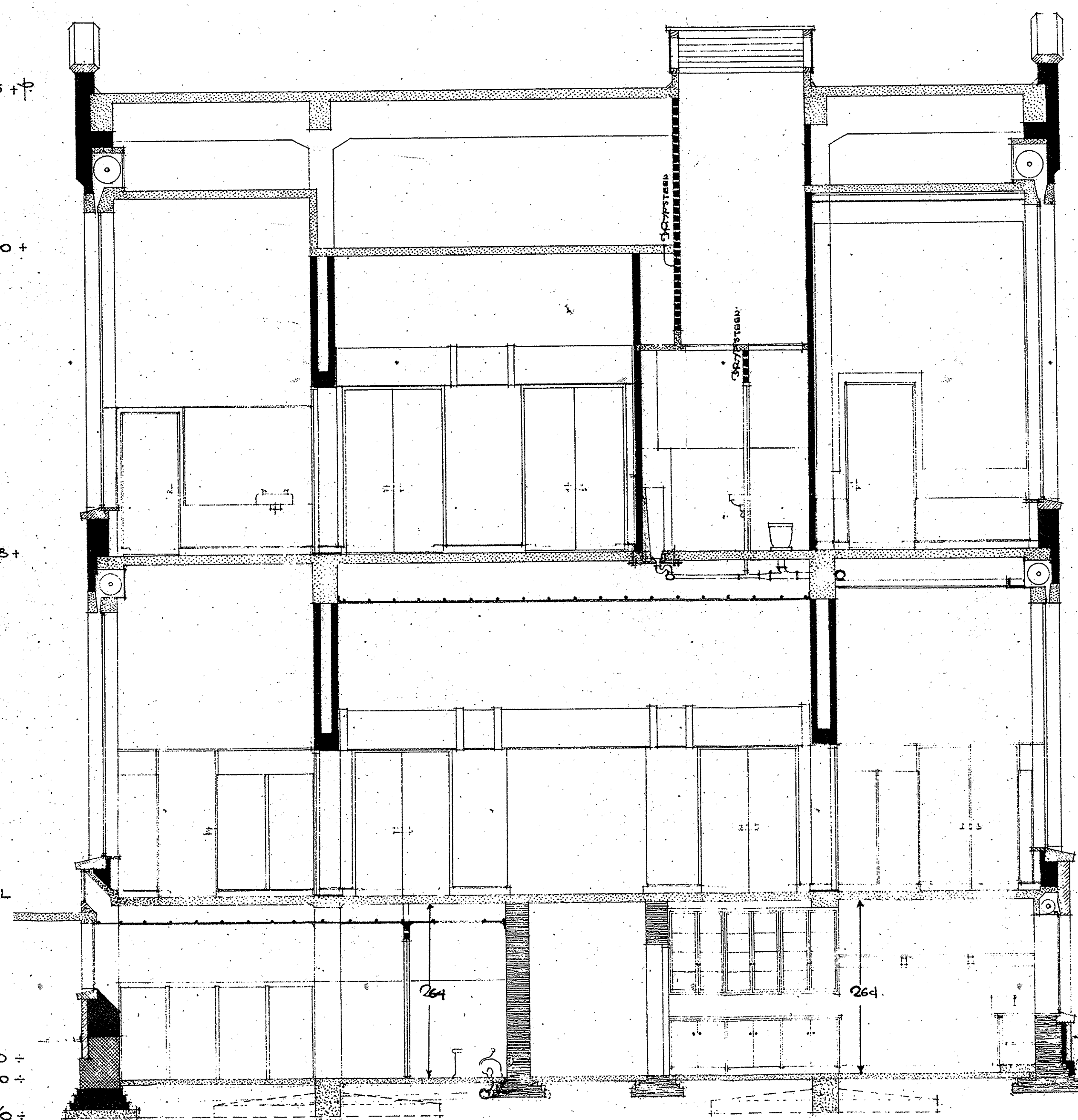
Doorsneden
