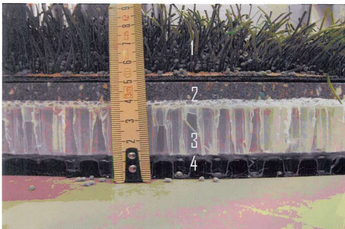
Figuur 1: Zijaanzicht constructie
