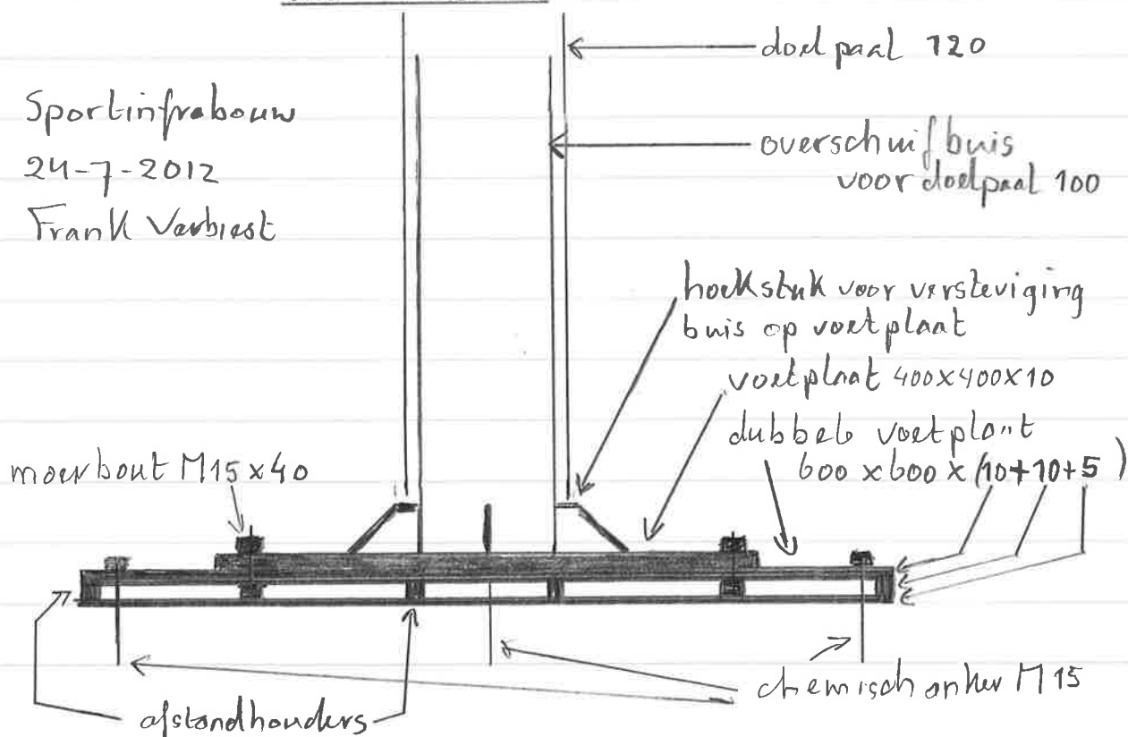
voor aanzicht
