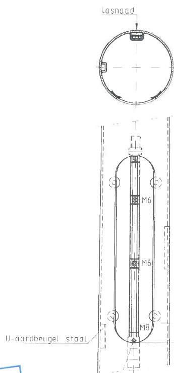
DETAIL BINNENWERK
