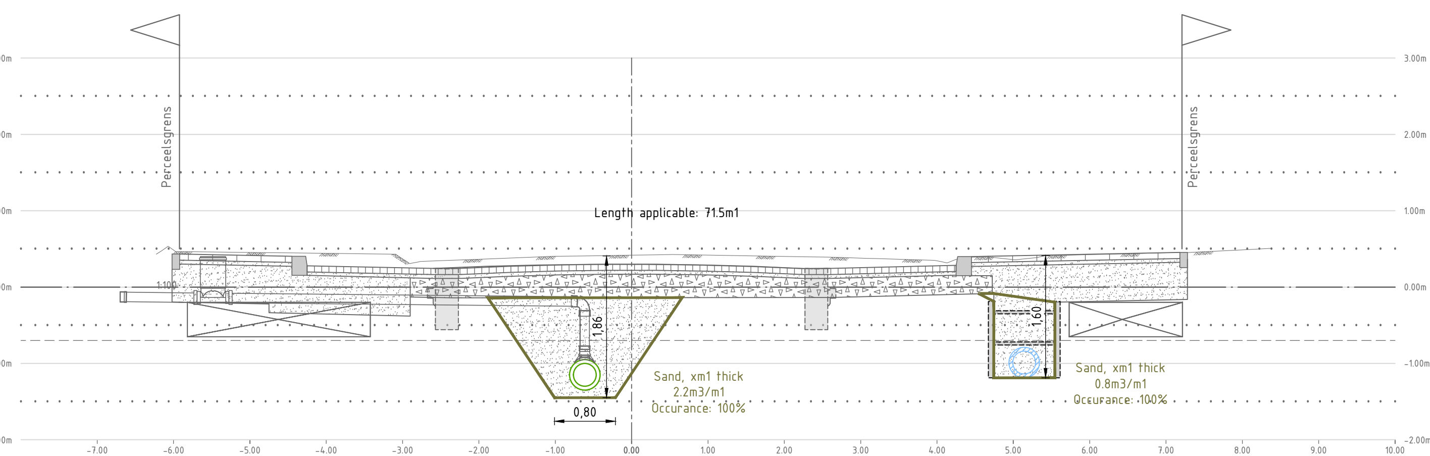
Dwarsprofiel DP-07 - Jan Luikenstraat Schaal 1:50
