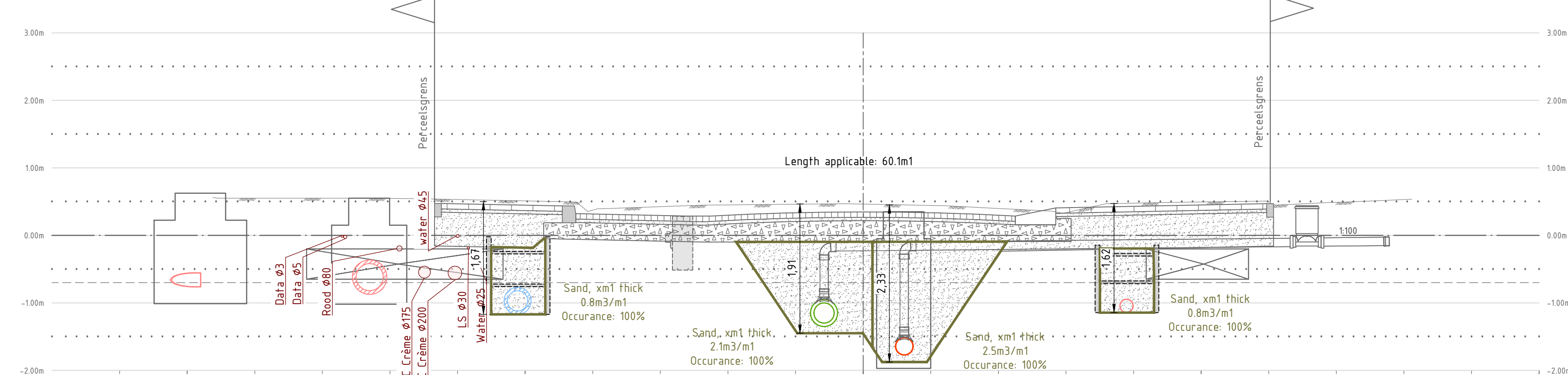
Dwarsprofiel DP-08 - Rijnvis Feithlaan Schaal 1:50
