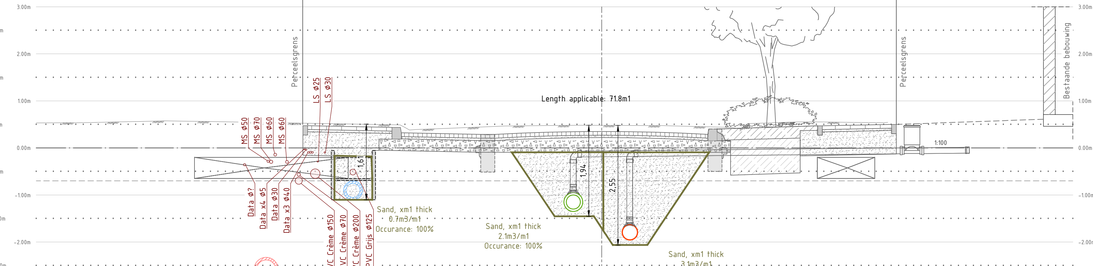
Dwarsprofiel DP-08 - Rijnvis Feithlaan Schaal 1:50
