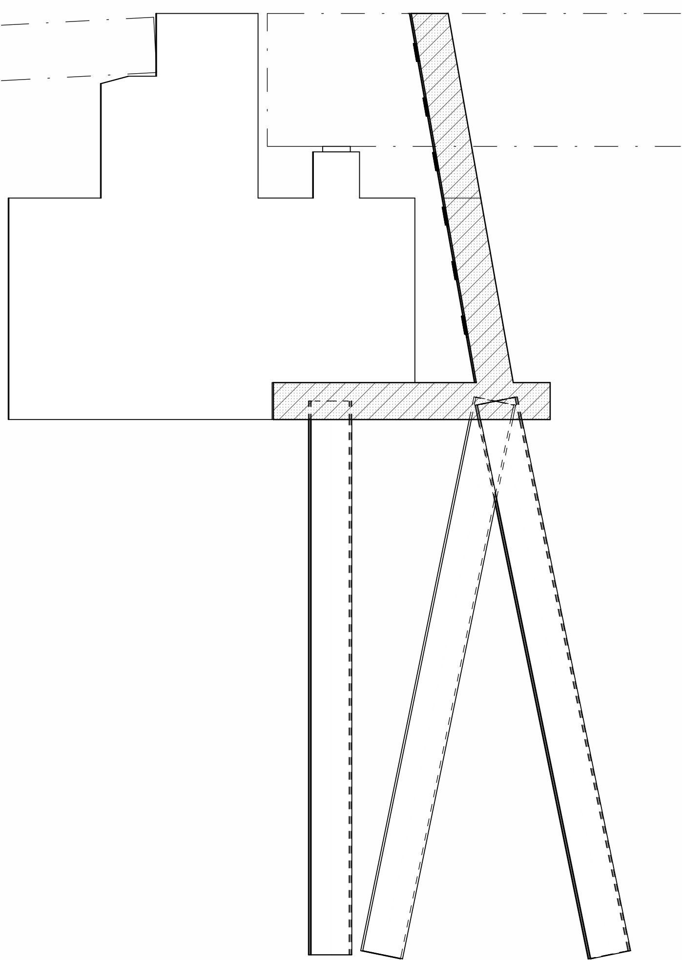
Doorsnede variant 2 schaal: 1:20
