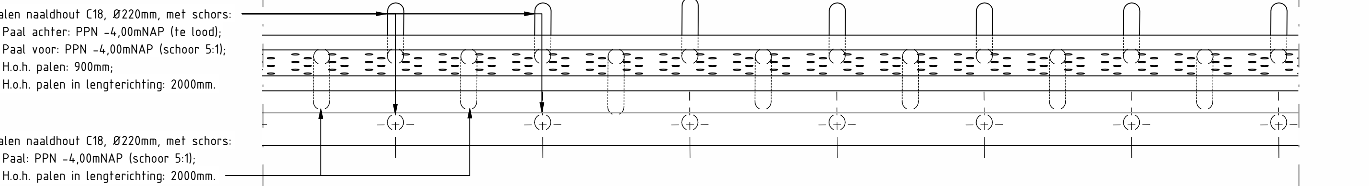
Principedetail locaties palen schaal: 1 : 50
