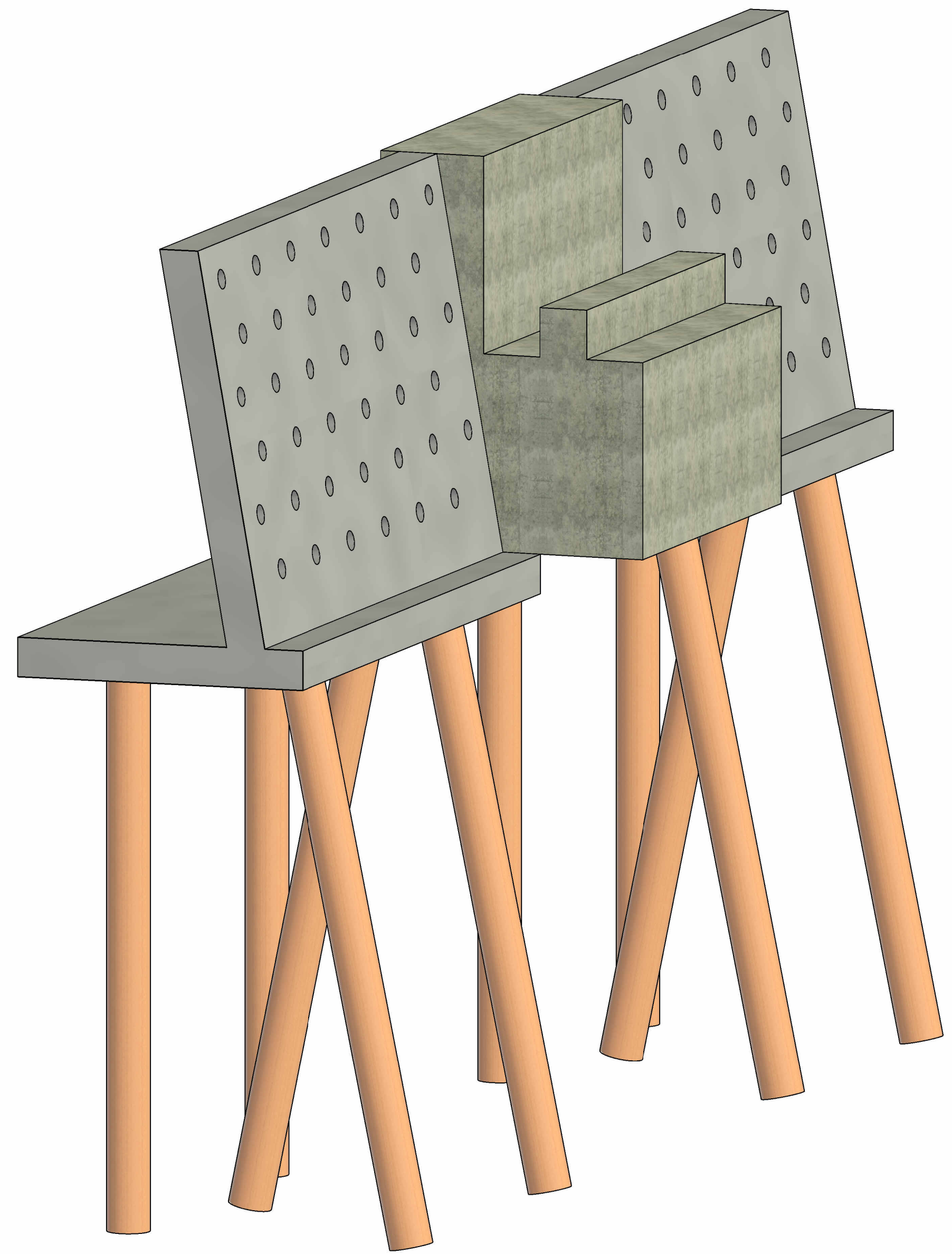
3D aanzicht variant 1 schaal: 1:20
