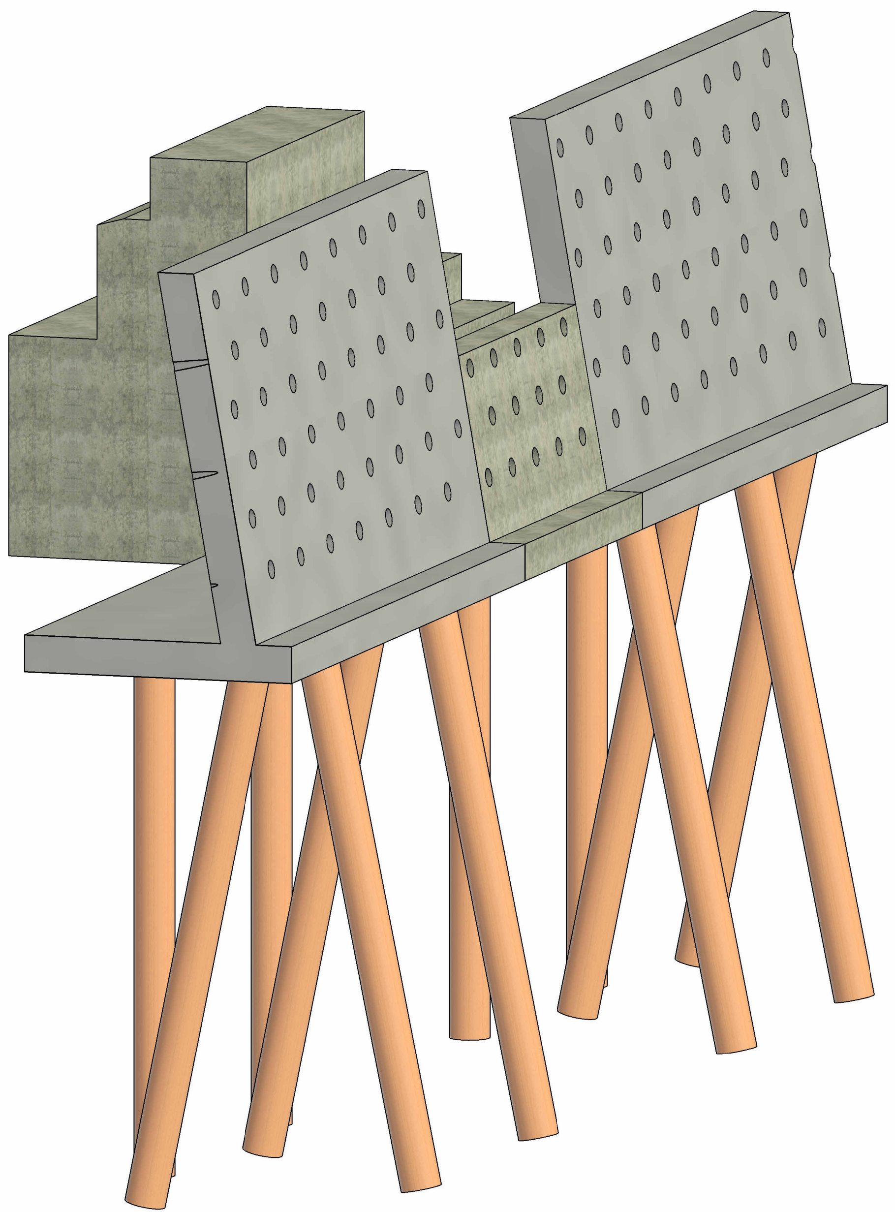
3D aanzicht variant 2 schaal: 1:20
