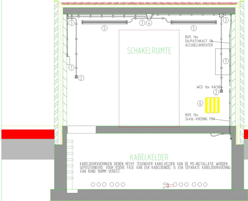
DOORSNEDE A-B
