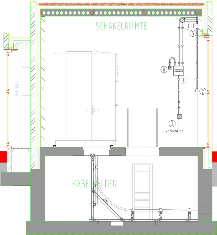
DOORSNEDE E-F
