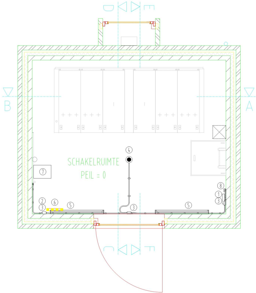
BEGANE GRONDVLOER
