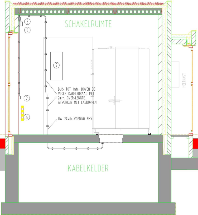
DOORSNEDE C-D
