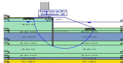
Totale Stabiliteit - Fase 1: Eindsituatie
