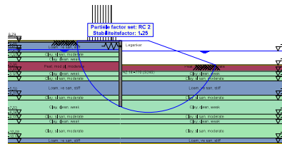
Totale Stabiliteit - Fase 1: Eindsituatie
