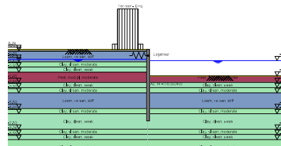
Overzicht - Fase 1: Eindsituatie
