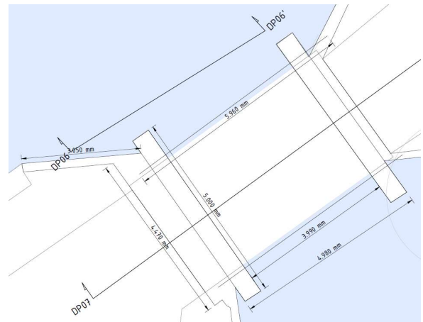
Globale afmetingen bestaande brug (bron: De Aquanoom)
