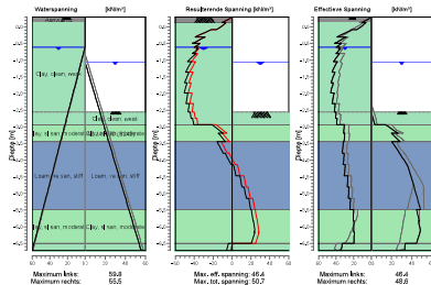
Spanningstoestanden - Fase 1: Eindsituatie
