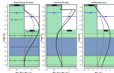
Momenten/Krachten/Verplaatsingen - Fase 1: Eindsituatie Stap 6.3 - Partiele factor set: RC 2
