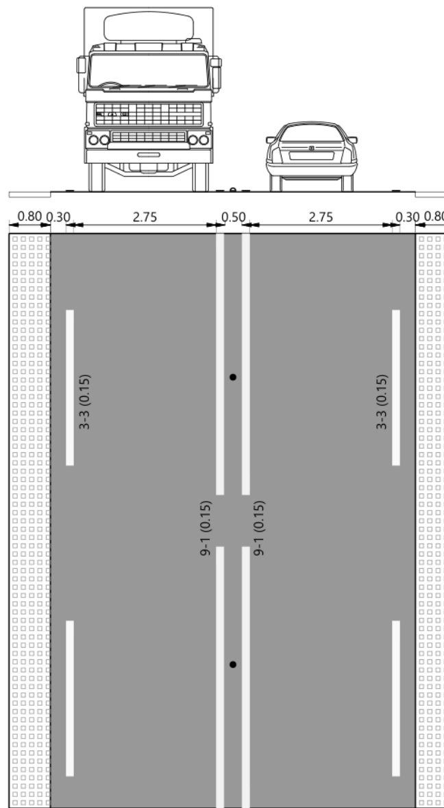
Principeprofiel: BuBeKo Schaal 1:100
