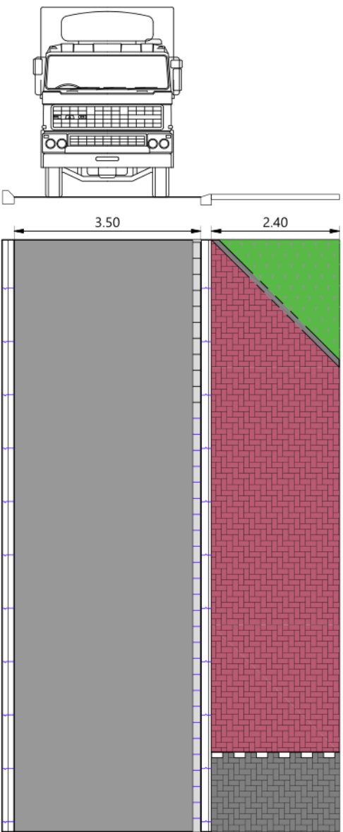
Principeprofiel: kom Slagharen Schaal 1:100
