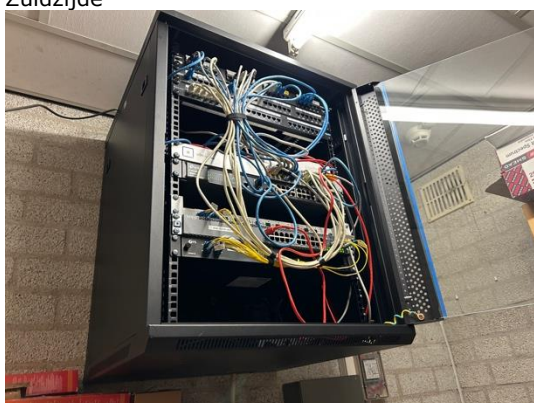
Patchkast
