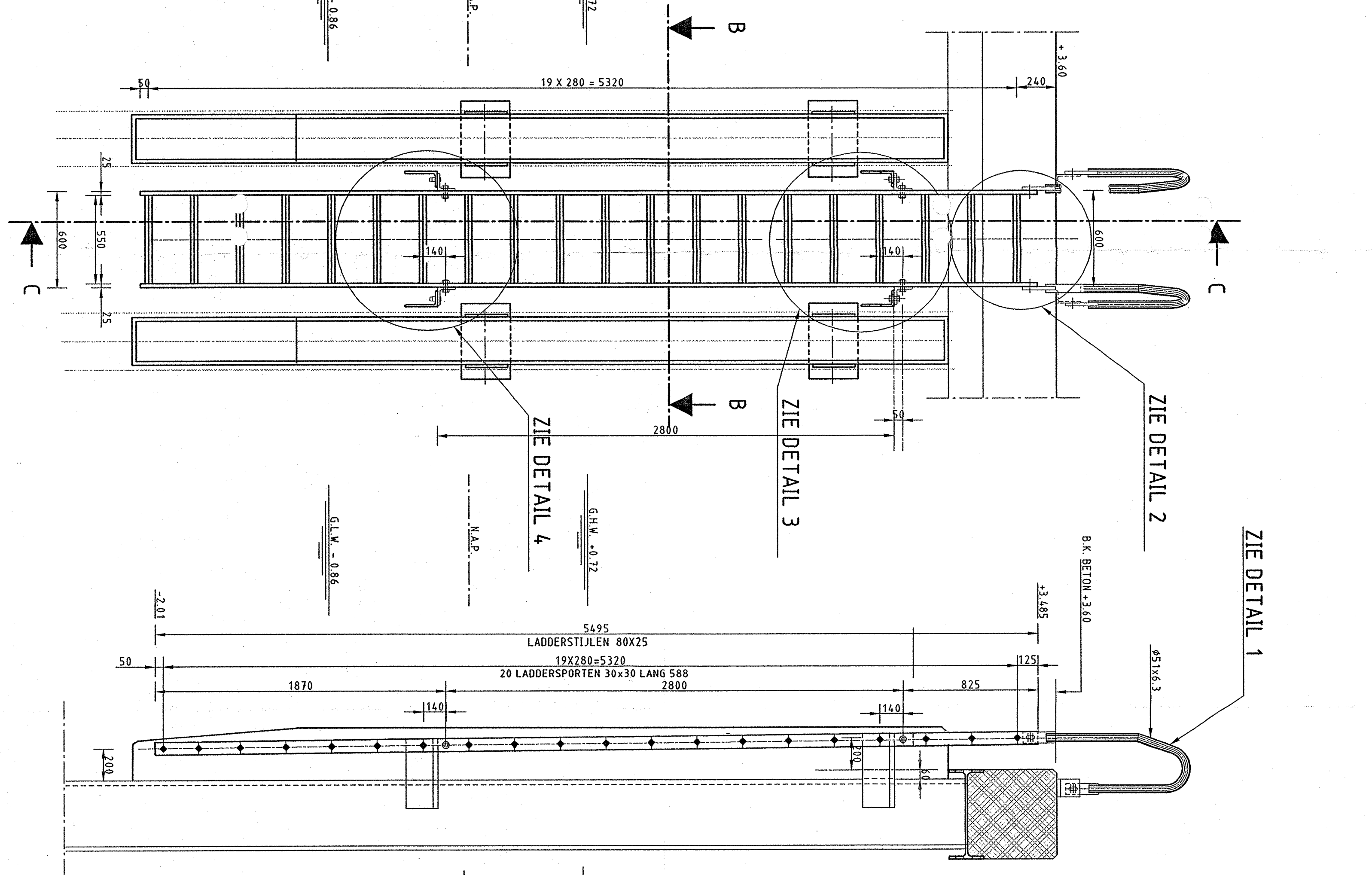
VOORANZICHT - LADDER (1:10)
