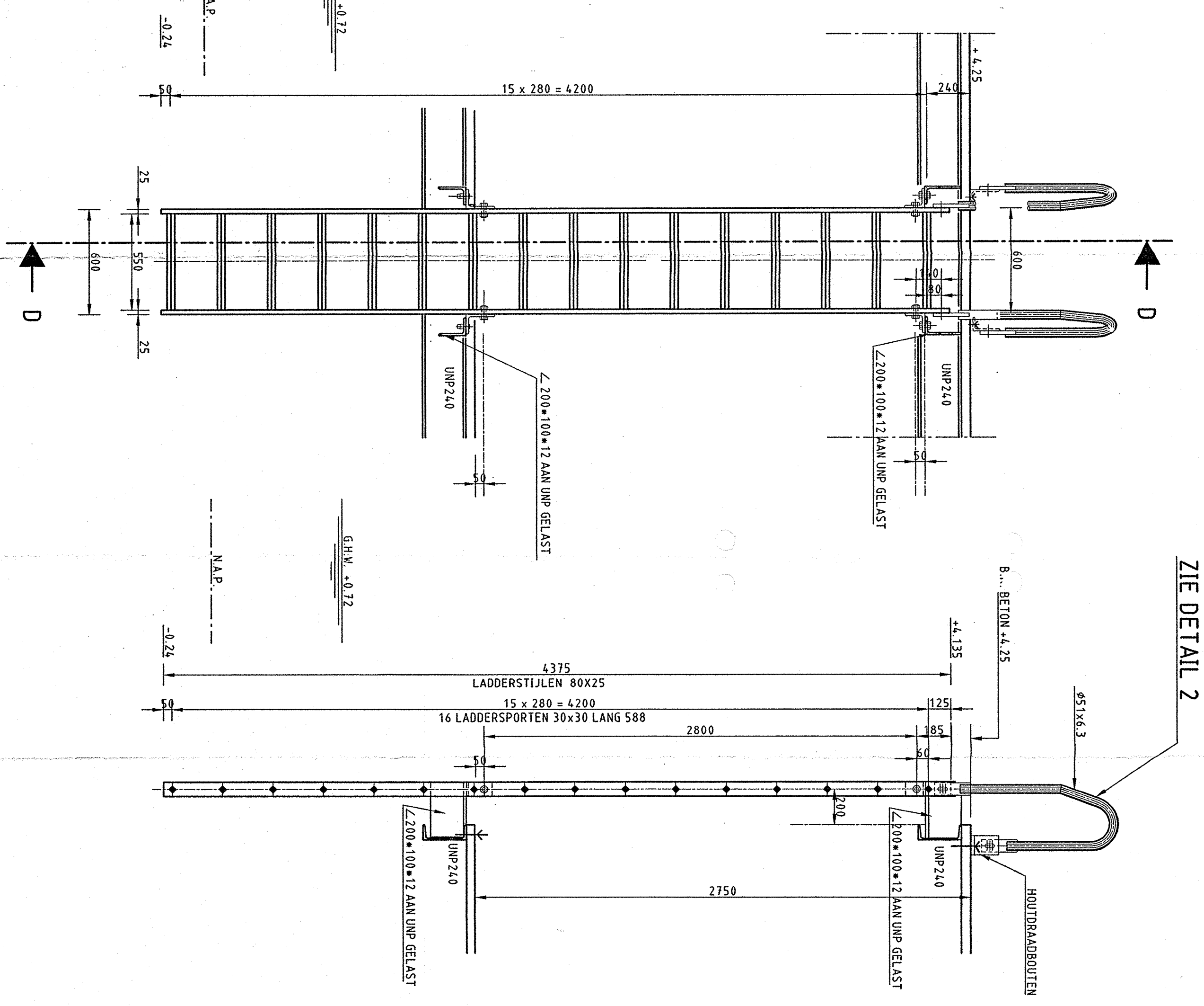
VOORANZICHT - LADDER (1:10)
