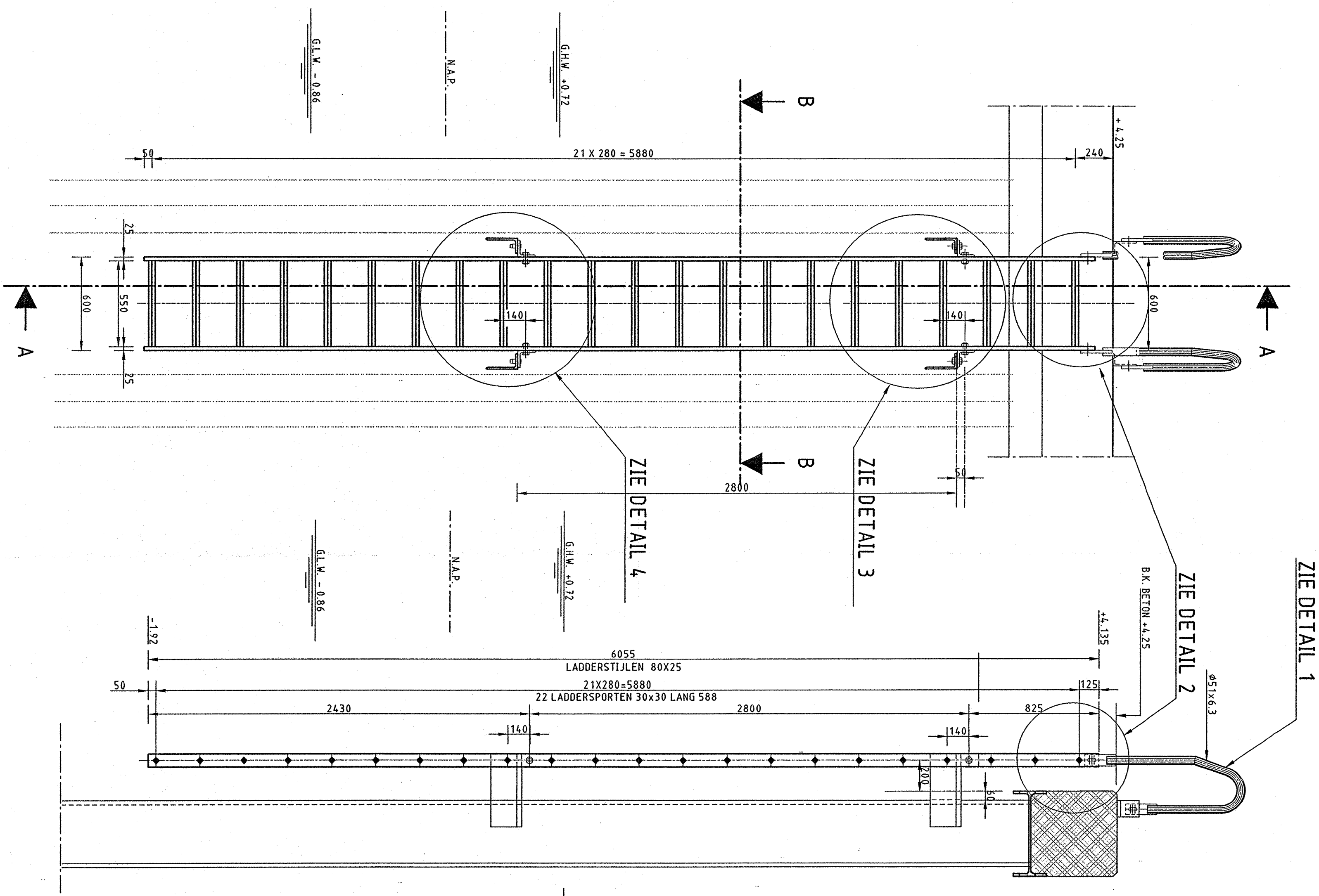
VOORANZICHT - LADDER (1:10)
