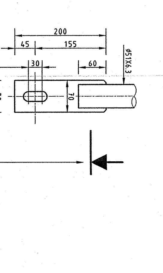
ZIJANZICHT (1:5)
