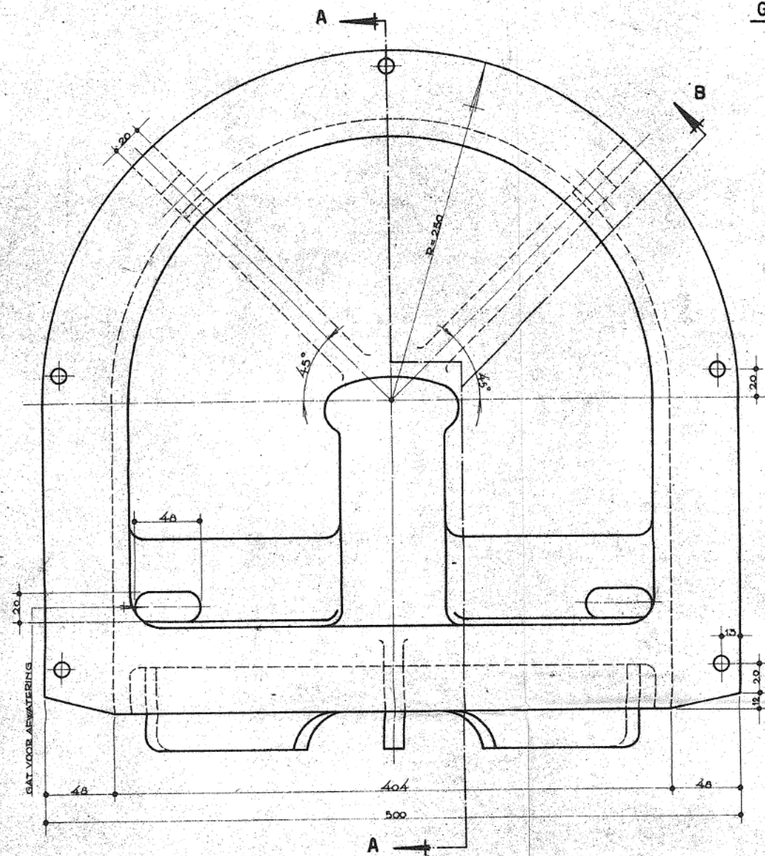
VOORAANZICHT.
