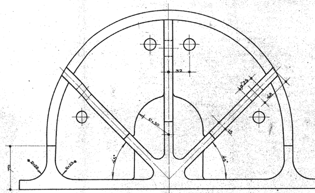
ONDERAANZICHT.
