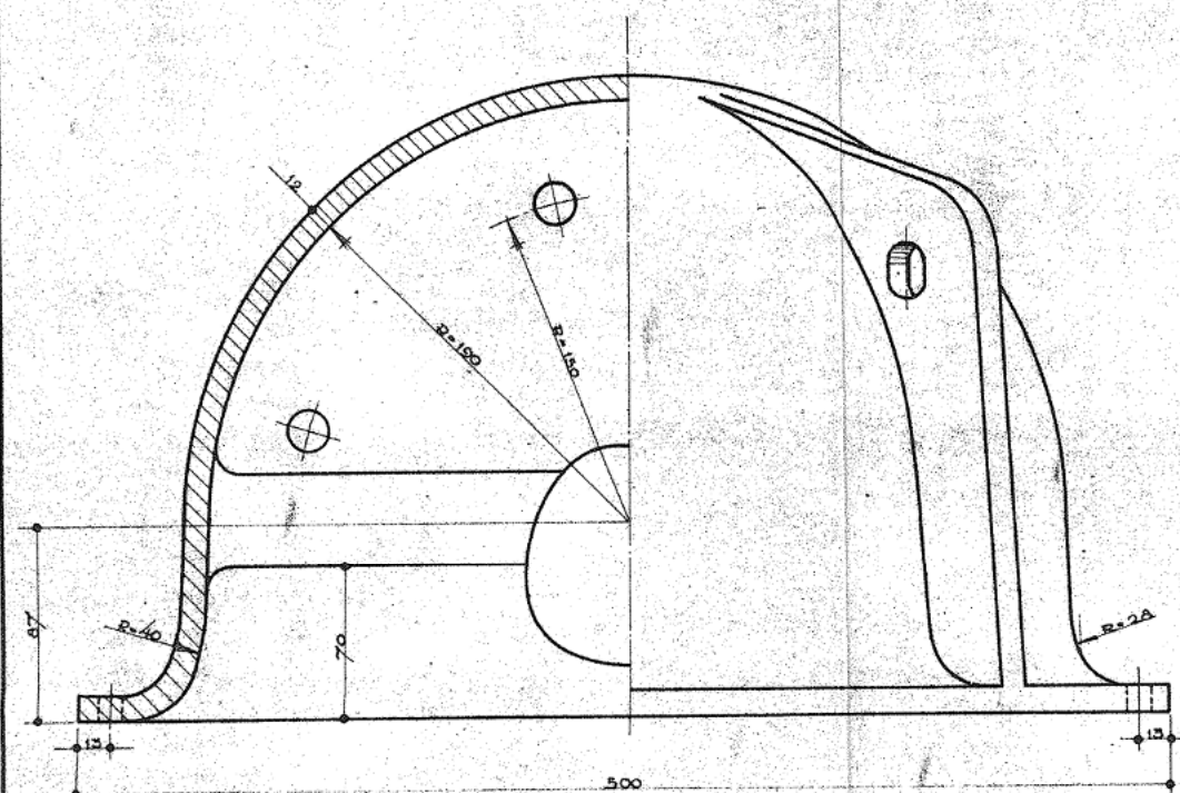
HALVE DOORSNEDE
