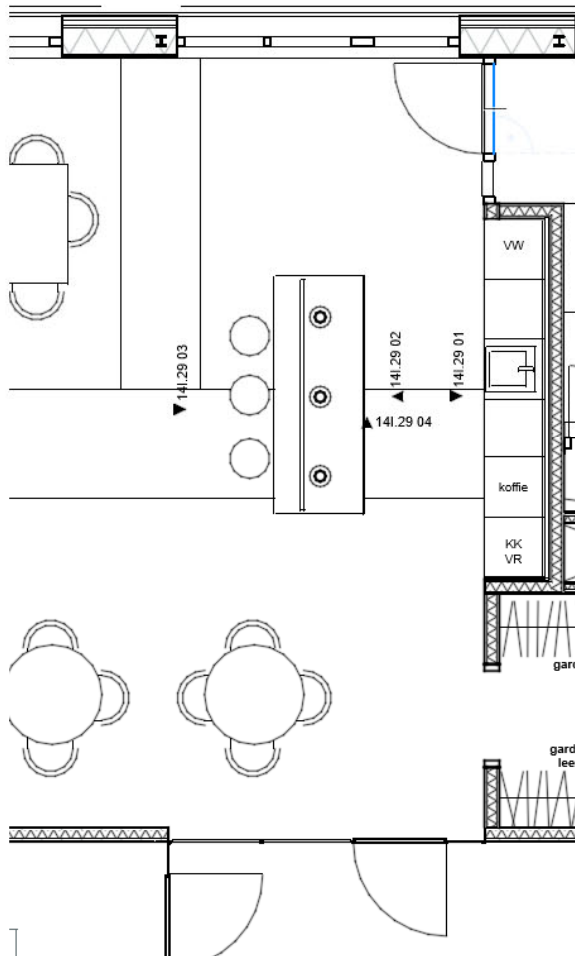
01 1e verdieping
