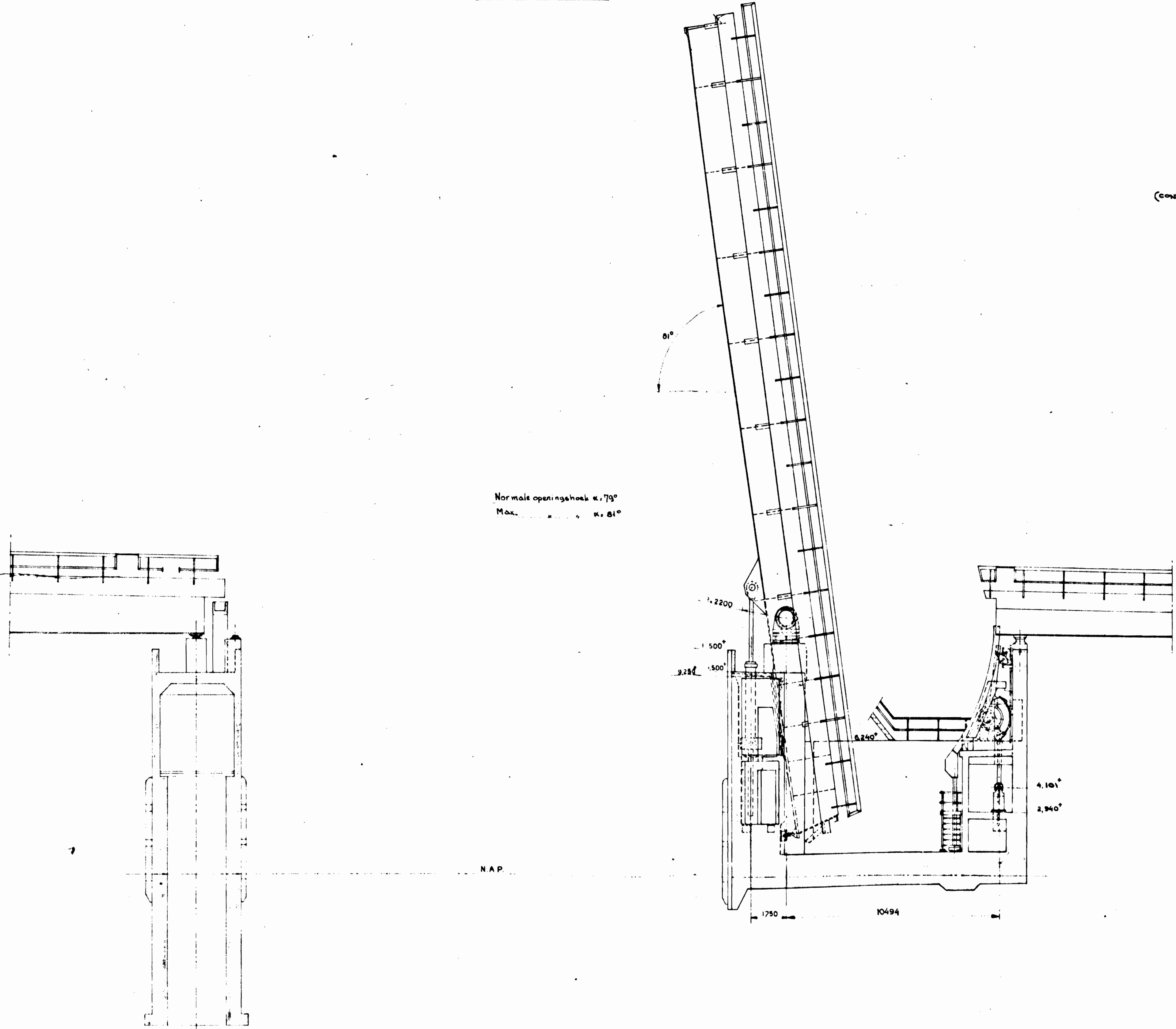
DOORSNEDE A-A.
