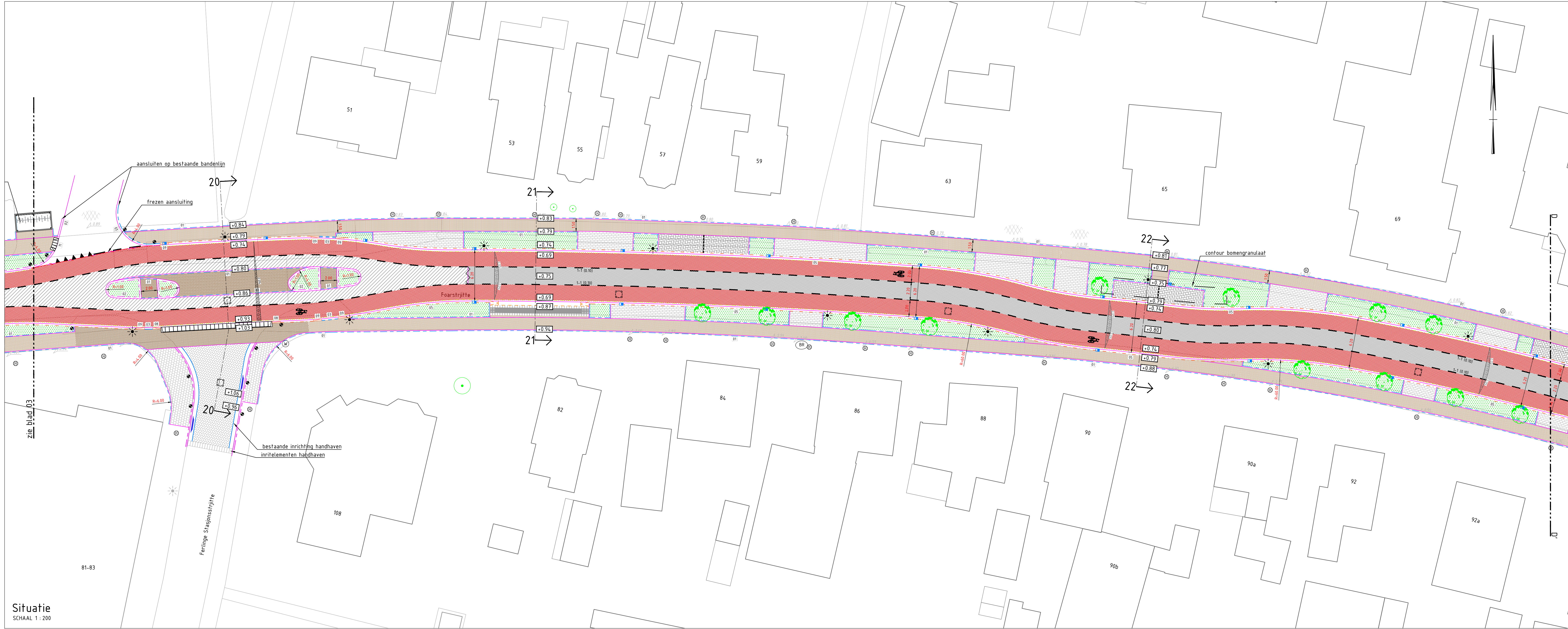
Overzichtstekening SCHAAAL 1:1000
