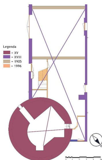
Voorbeeld van een gedetailleerde faseringstekening (opname).
