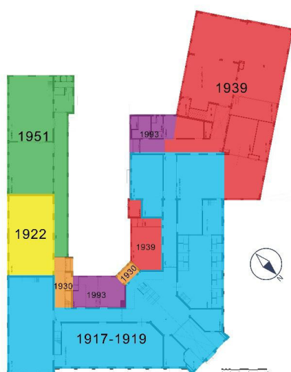
Voorbeeld van een globale faseringstekening (verkenning).
