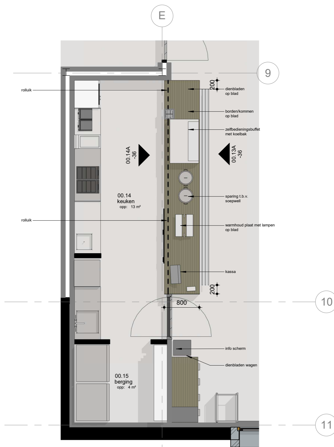
PLATTEGROND schaal : 1 : 50
