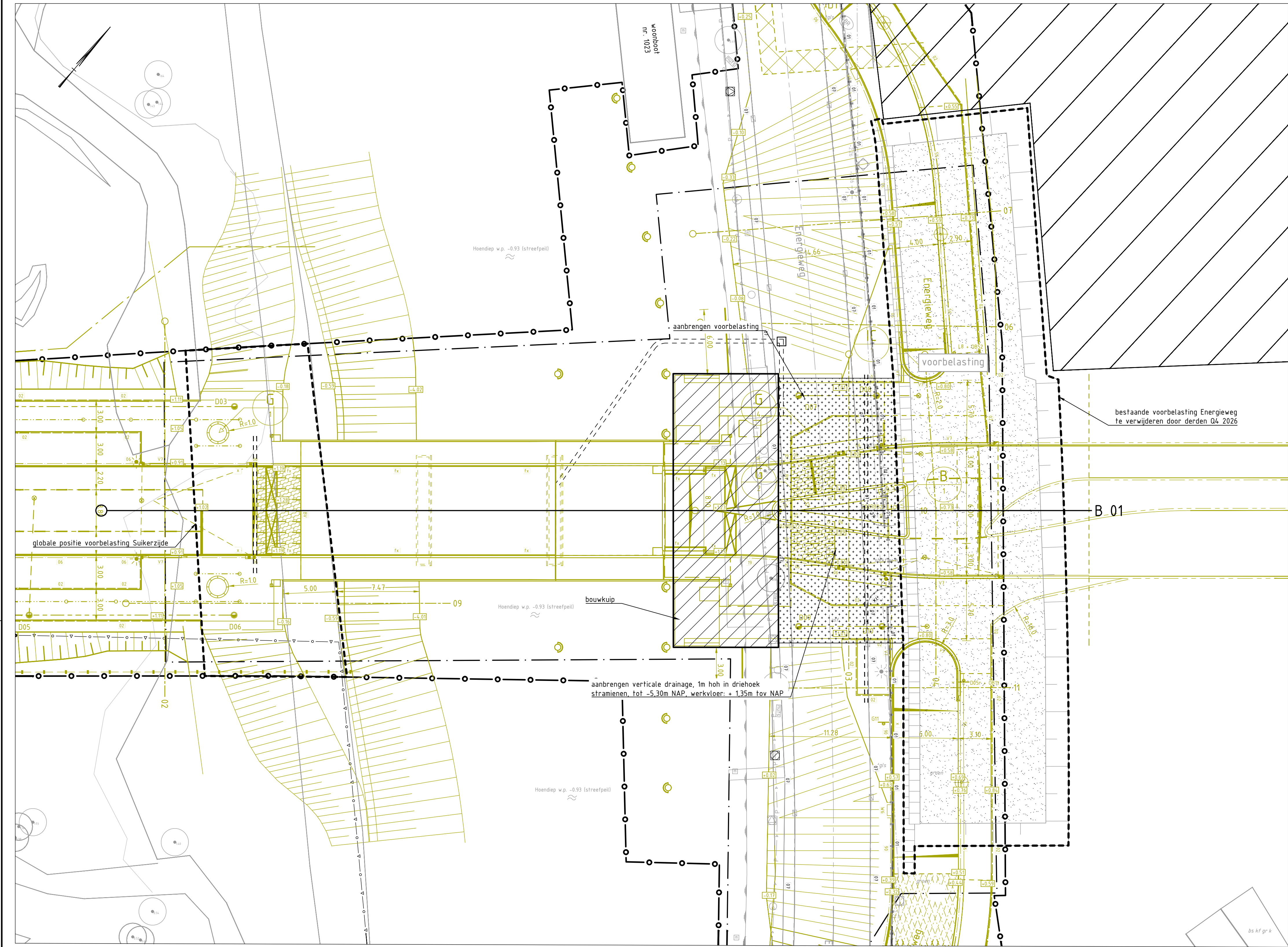
SITUATIE - COMBINATIE BESTAAND EN NIEUW schaal 1:200
