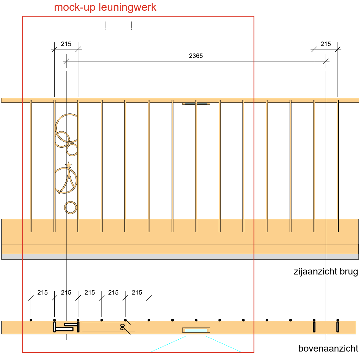
bovenaanzicht
