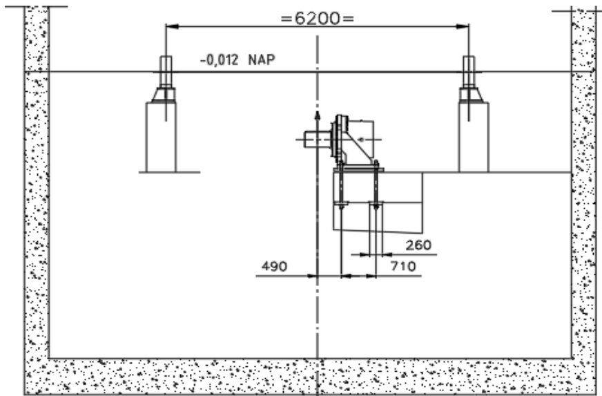
Doorsnede B-B
