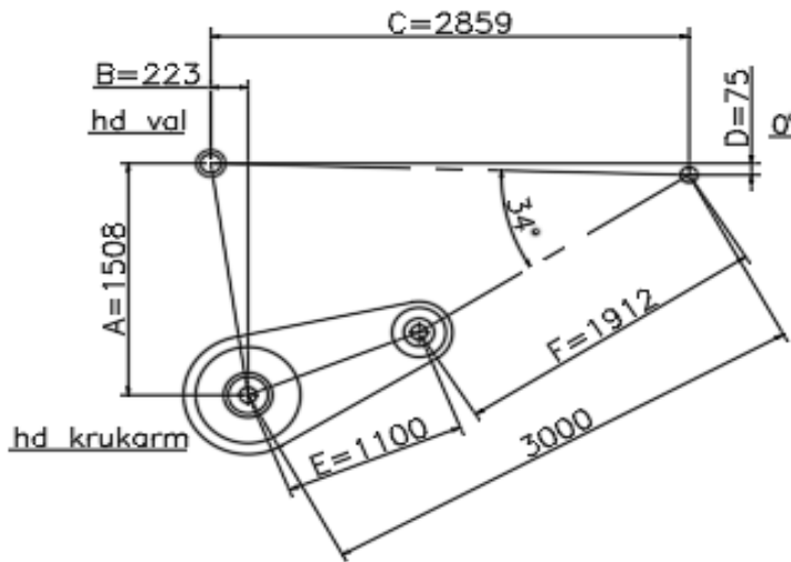
Geometrie krukarm en trekduwstang opgezet en niet opgezet
