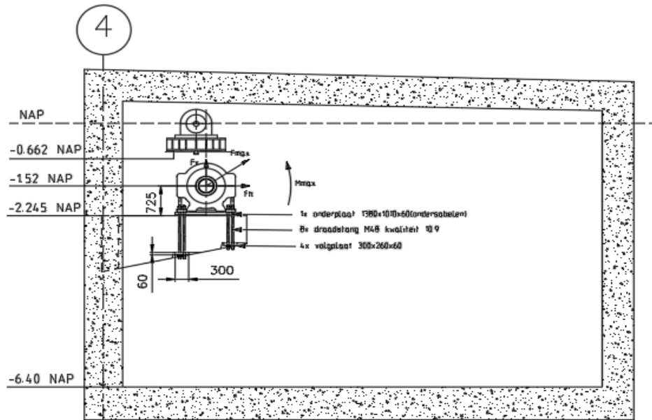
Doorsnede A-A
