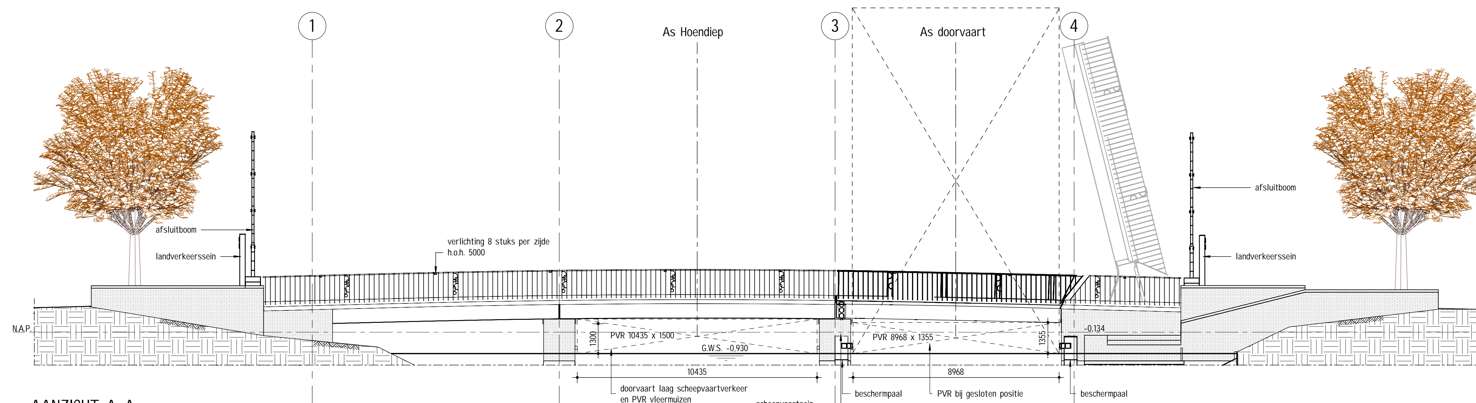
AANZICHT A-A schaal: 1 : 100
