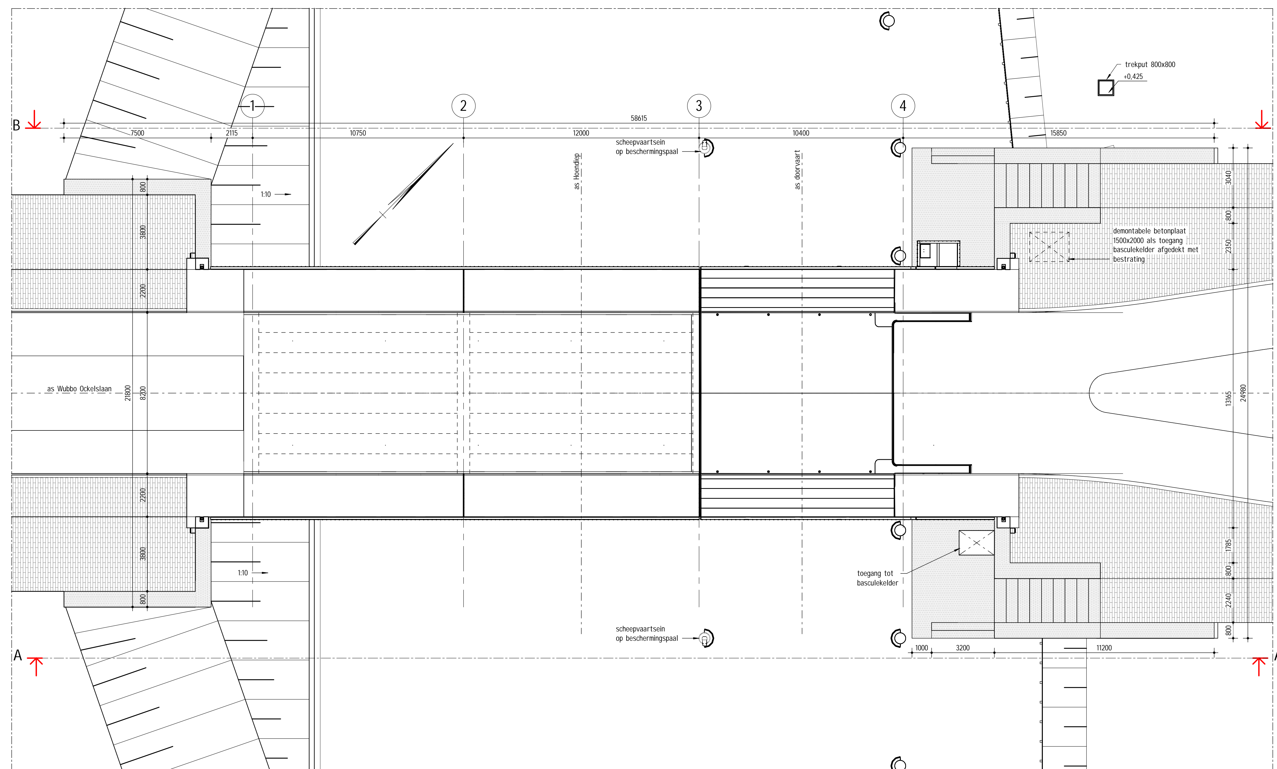
BOVENAANZICHT schaal: 1 : 100
