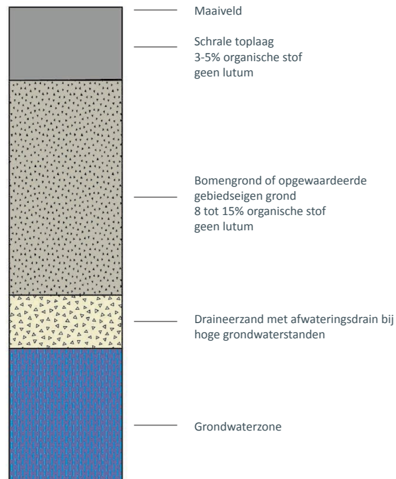
Profiel bodemopbouw gras/kruidentvegetatie
