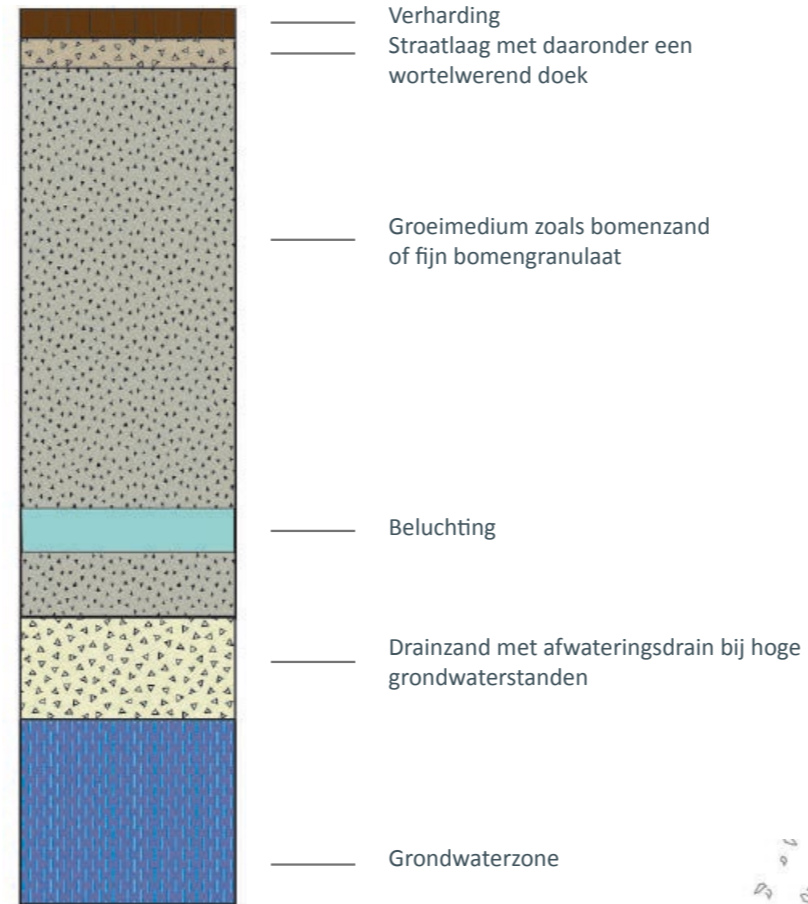
Profiel bodemopbouw
