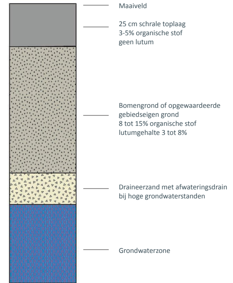
Profiel bodemopbouw
