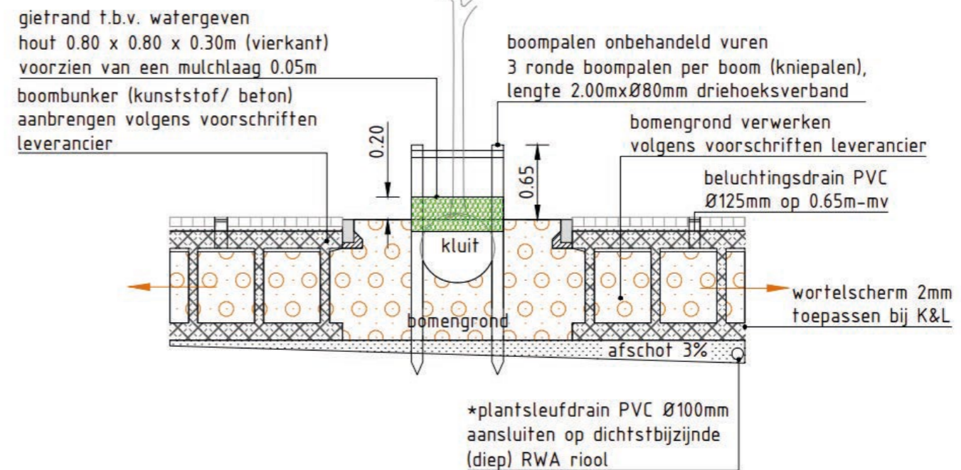
Standaard detail 3.1.4 Boom in verharding - Boombunker
