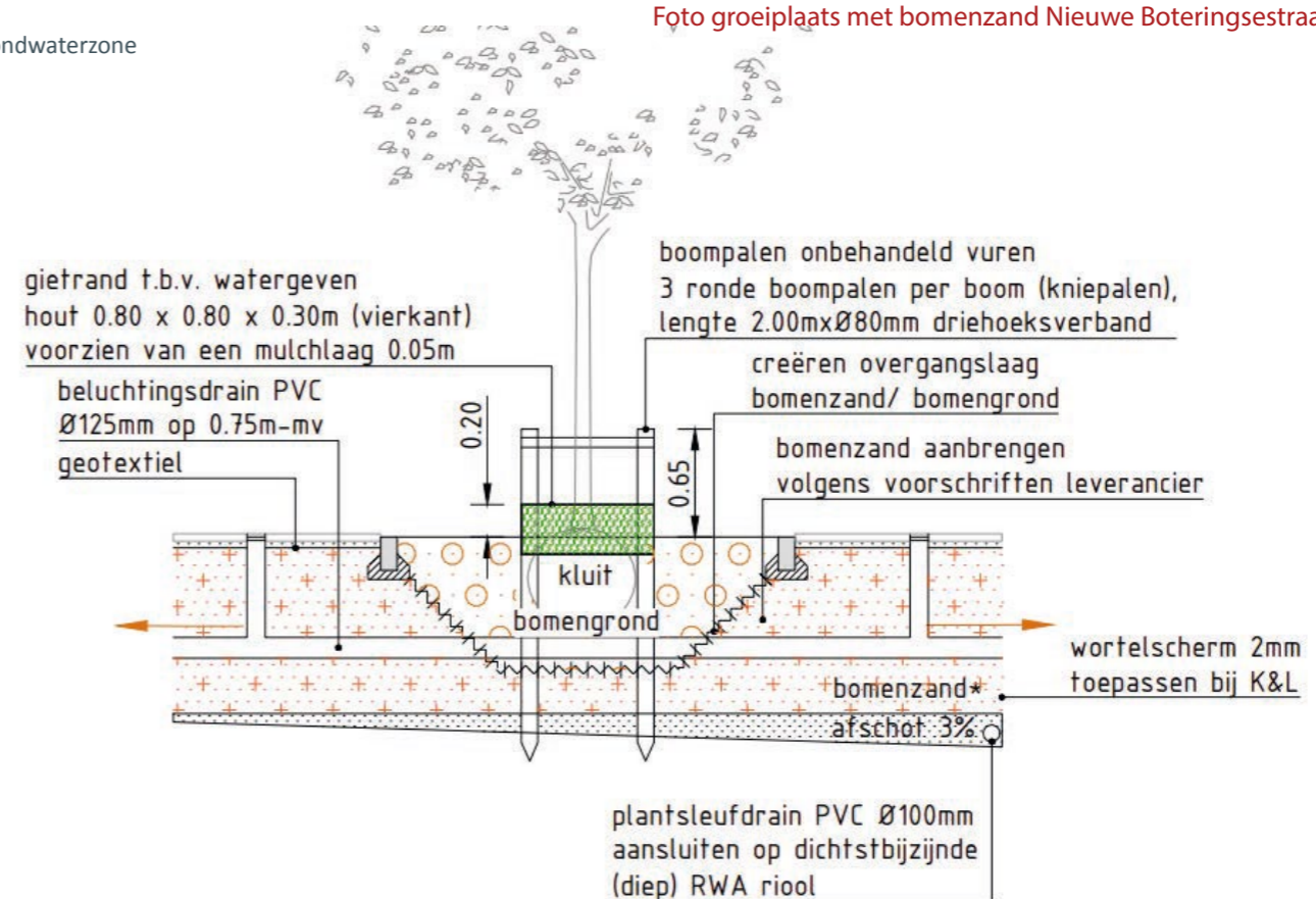
Standaard detail 3.1.1. Boom in verharding - Verkeersklasse A
