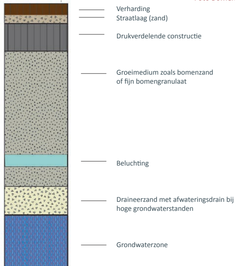
Profiel bodemopbouw
