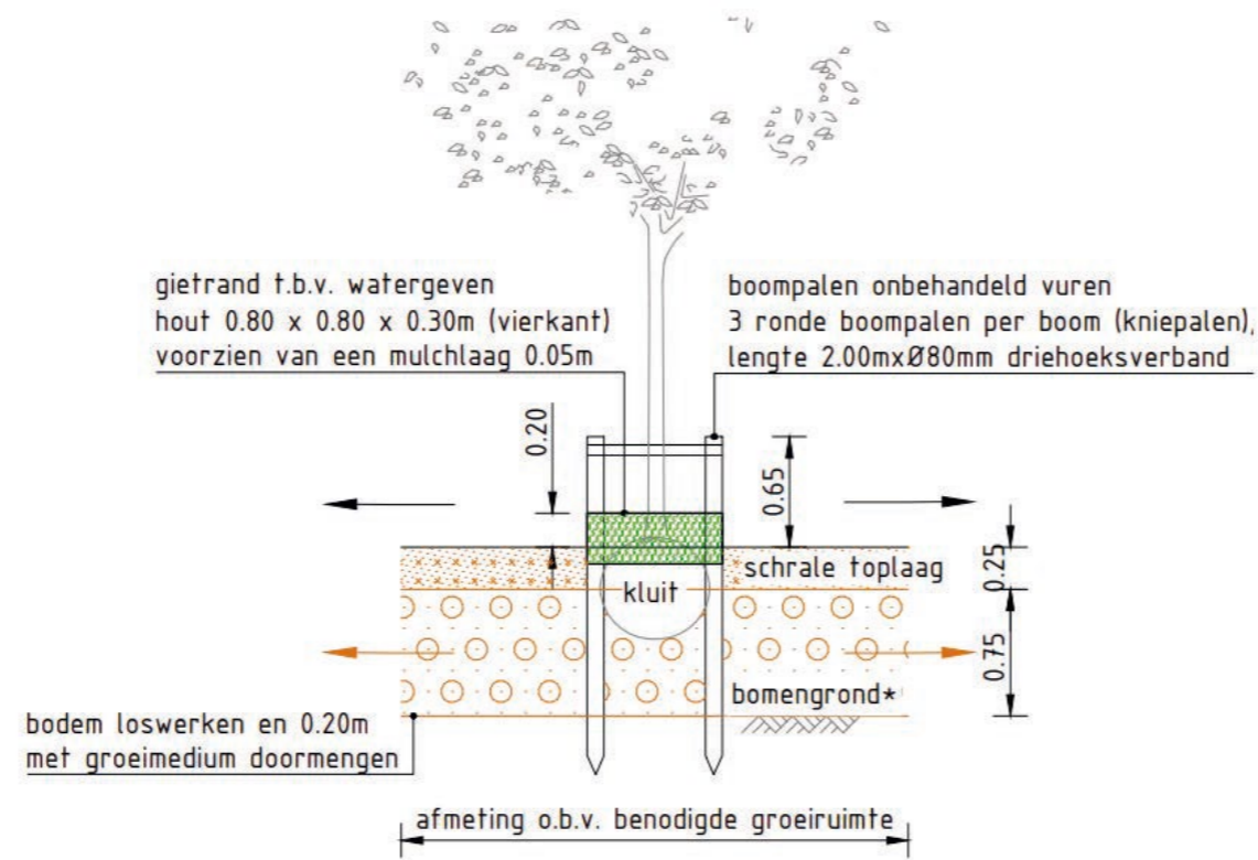
Standaard detail 3.1.7. Boom in schrale bloemrijke - grasvegetaties
