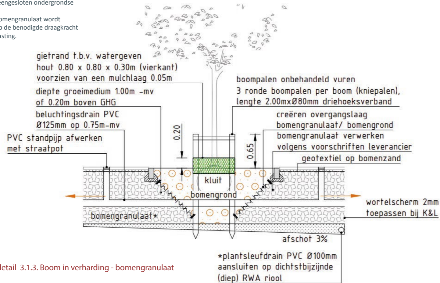
Profiel bodemopbouw
