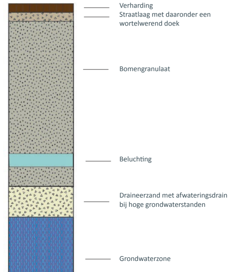
Profiel bodemopbouw
