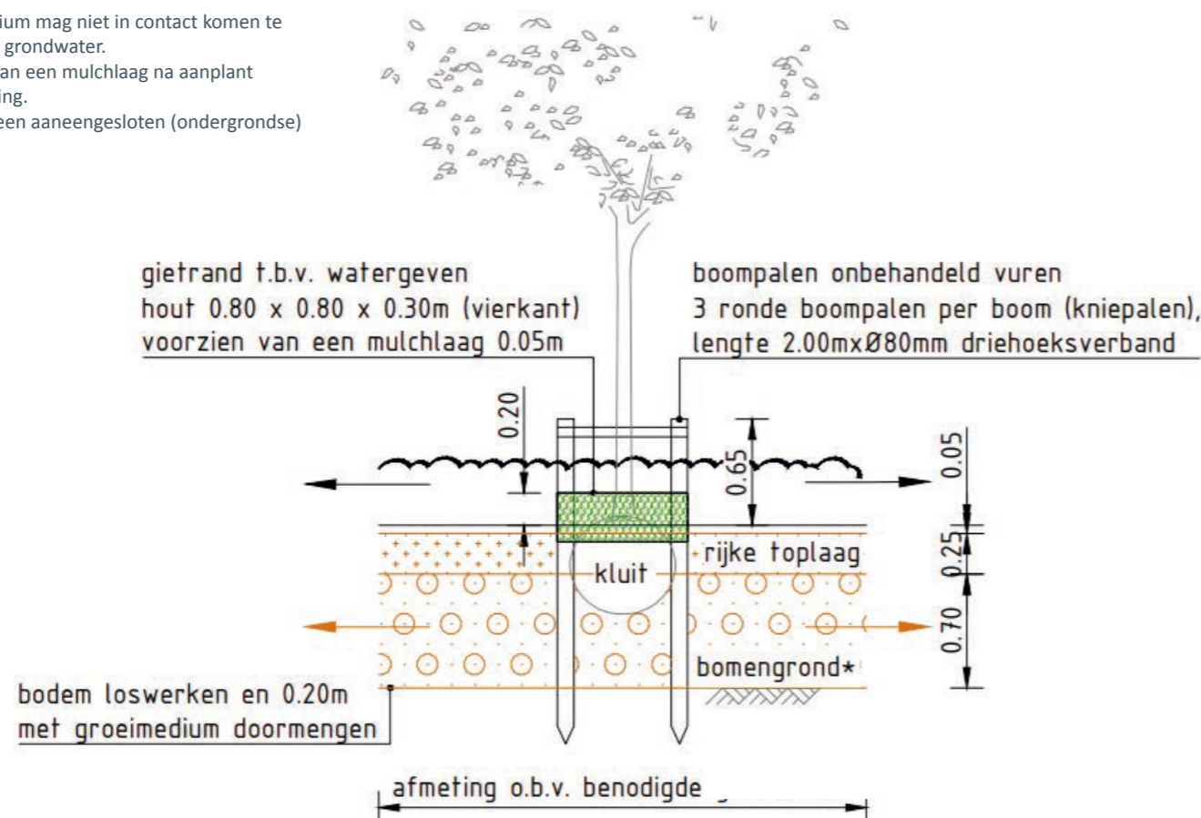
Standaard detail 3.1.6 Boom in open grond - Beplantingen
