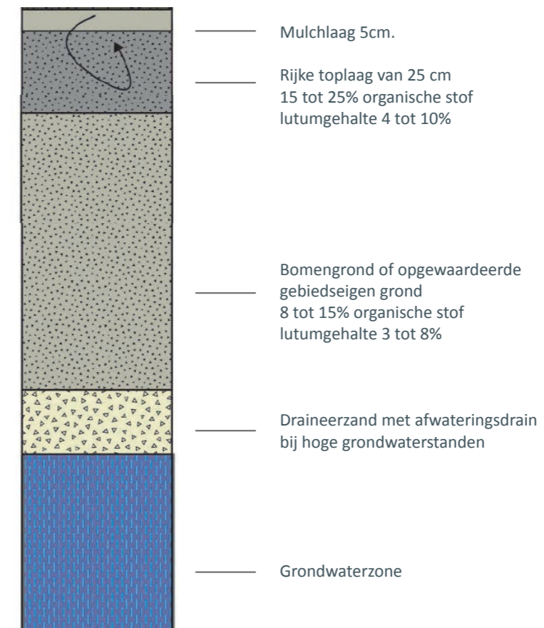
Principeprofiel bodemopbouw
