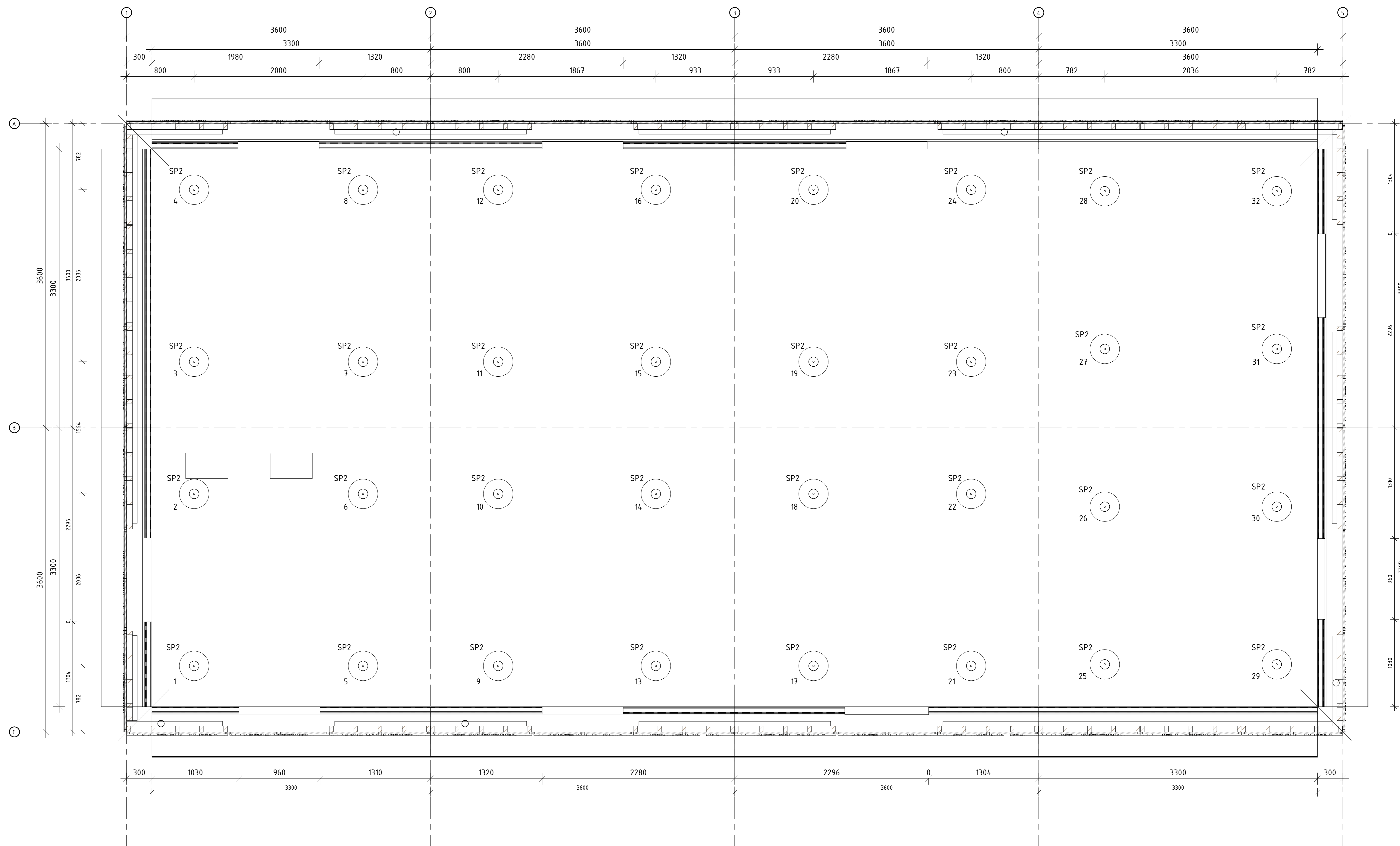
plattgrond fundering schaal 1:20
