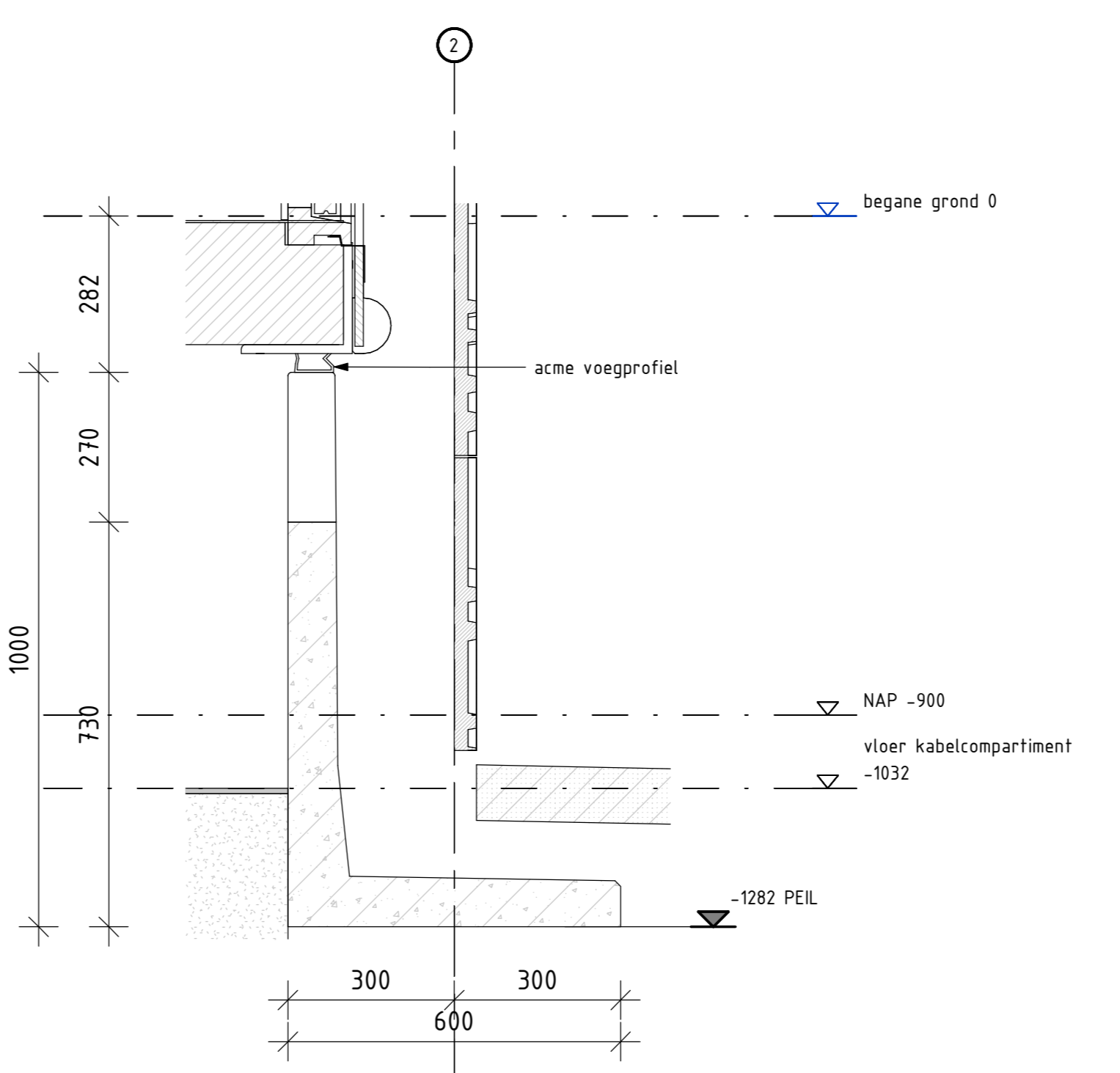
keerwand trapparing schaal 1:10
