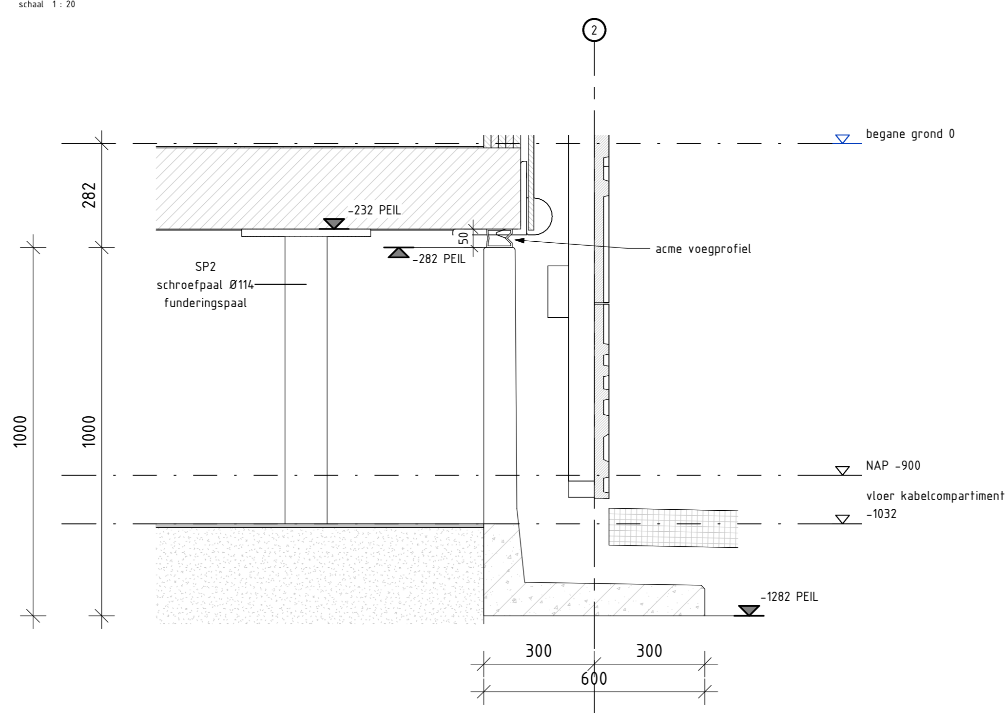
keerwand deurparing schaal 1:10
