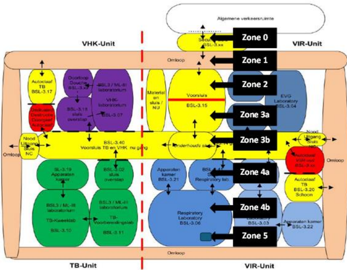
Figuur 1: Relatieschema ML-III faciliteit
