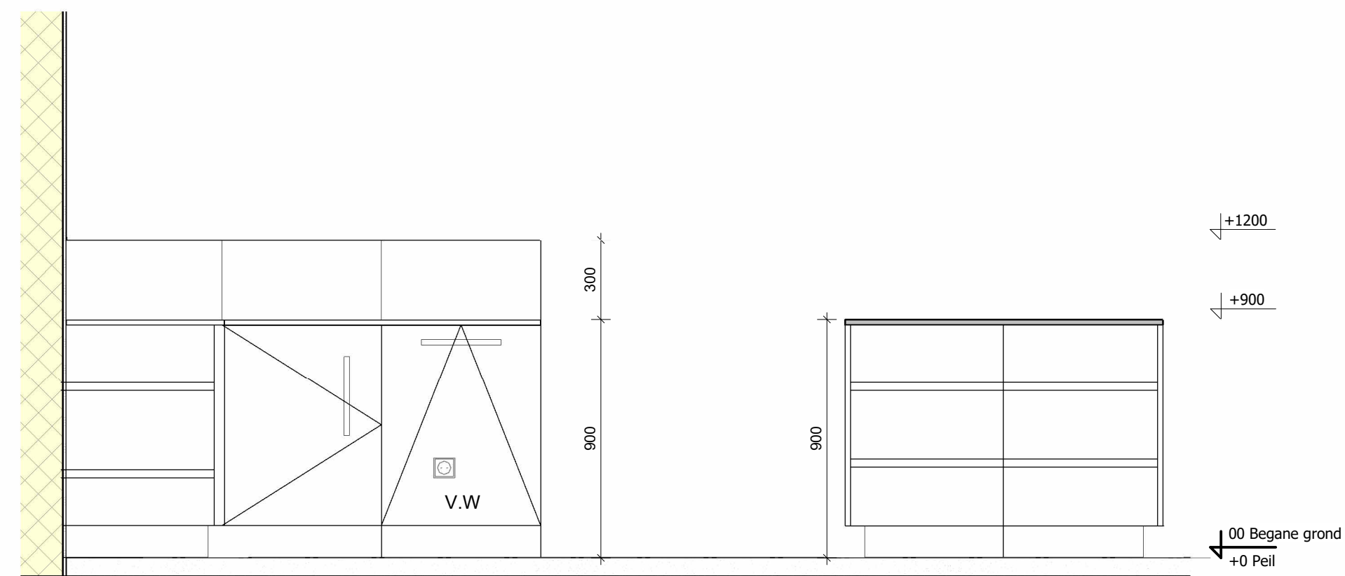
Doorsnede AA
