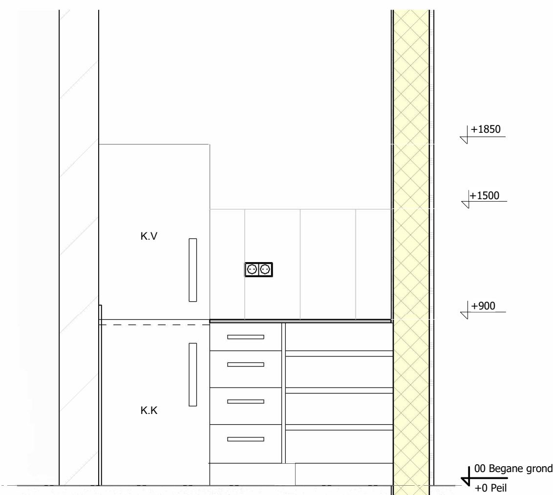
Aanzicht keukeneiland
