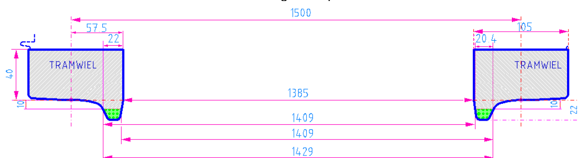
Figuur 1: Schematisch voorbeeld nominale Wielgeleidenmaten
