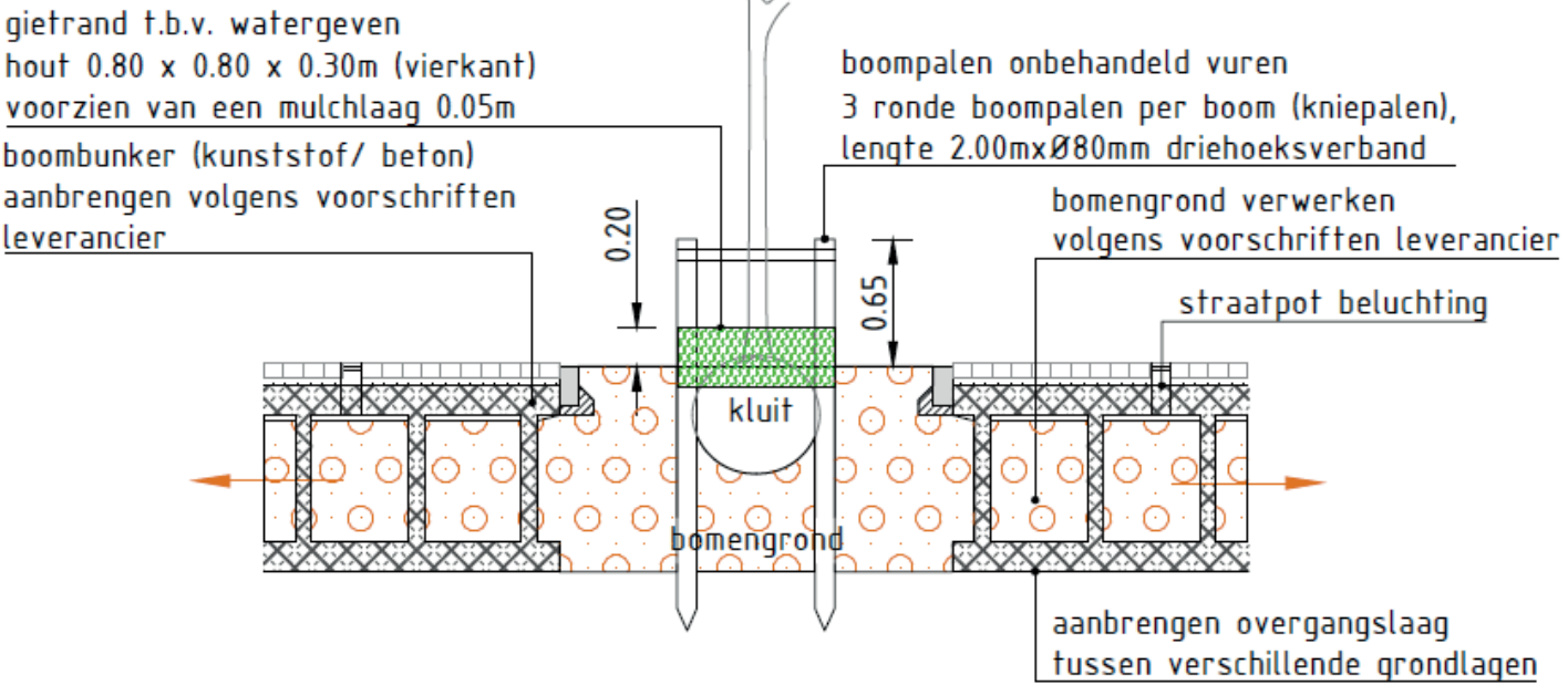
Standaard detail 3.1.4 Boom in verharding - Boombunker
