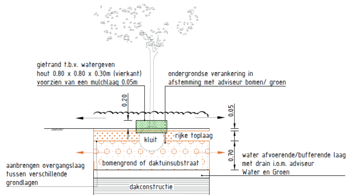
Standaard detail 3.1.8. Boom op dakconstructie
