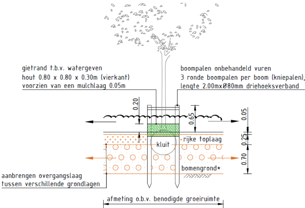
Standaard detail 3.1.6 Boom in open grond - Beplantingen
