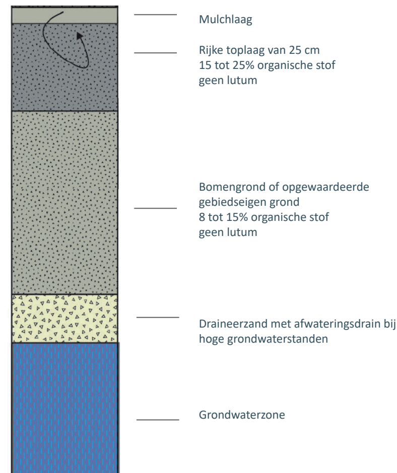
Principeprofiel bodemopbouw vaste planten/sierheesters
