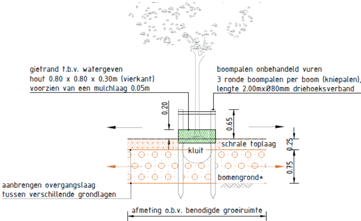
Standaard detail 3.1.7. Boom in schrale bloemrijke - grasvegetaties
