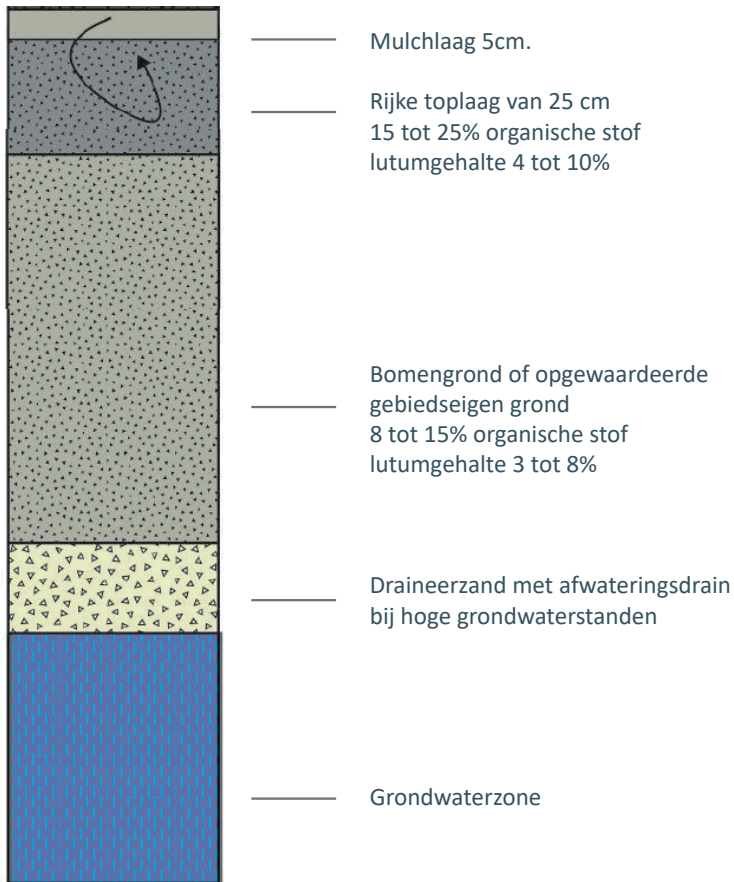
Principeprofiel bodempopbouw
