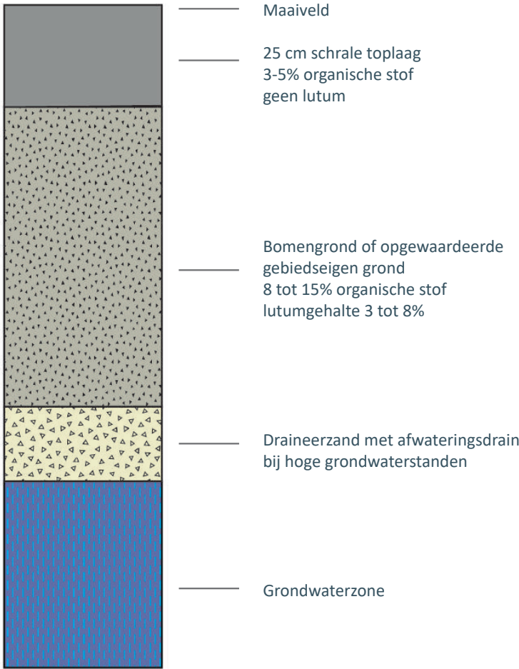
Profiel bodemopbouw
