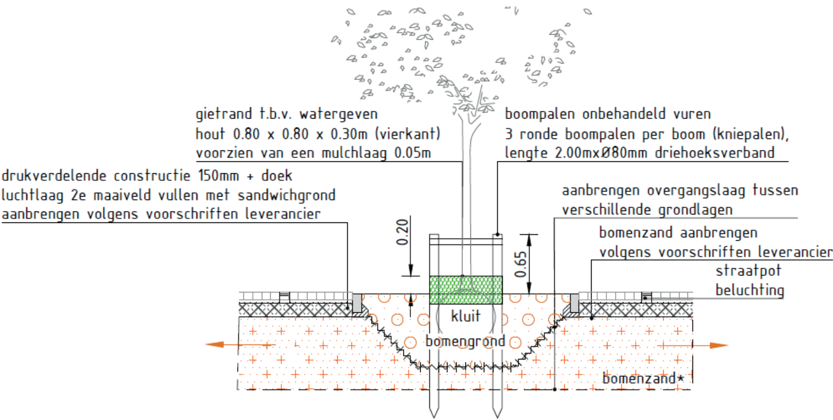
Standaard detail 3.1.2 Boom in verharding - Verkeersklasse B
