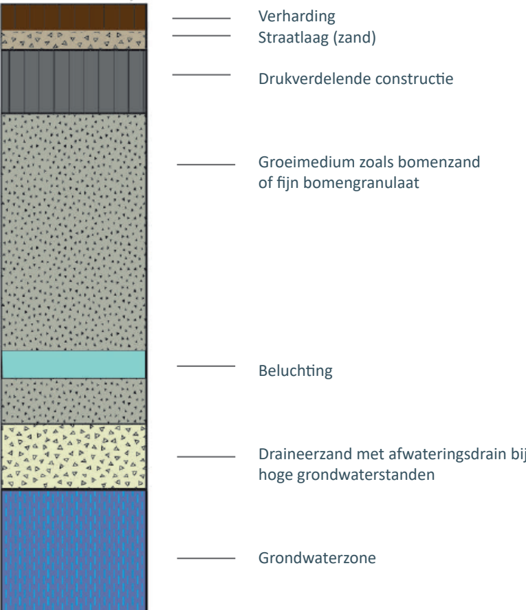
Profiel bodemopbouw
