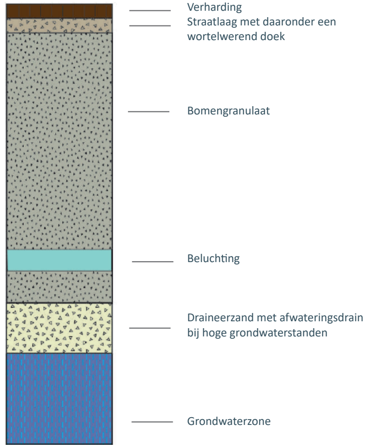
Profiel bodemopbouw
