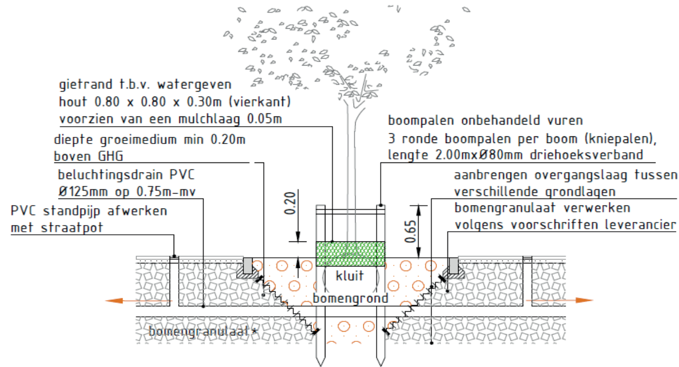
Standaard detail 3.1.3. Boom in verharding - bomengranulaat
