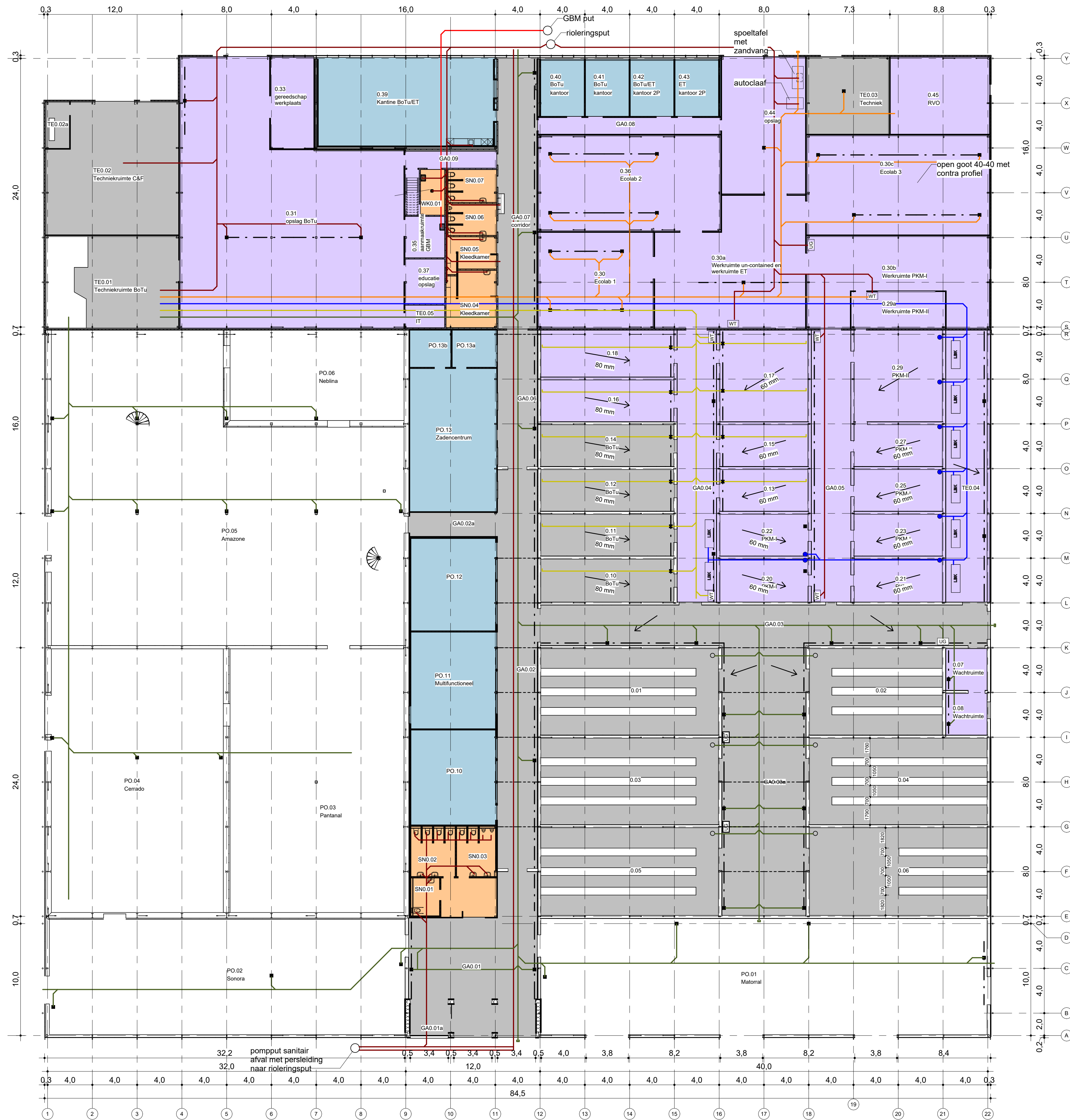
Begane grond 1 : 200
