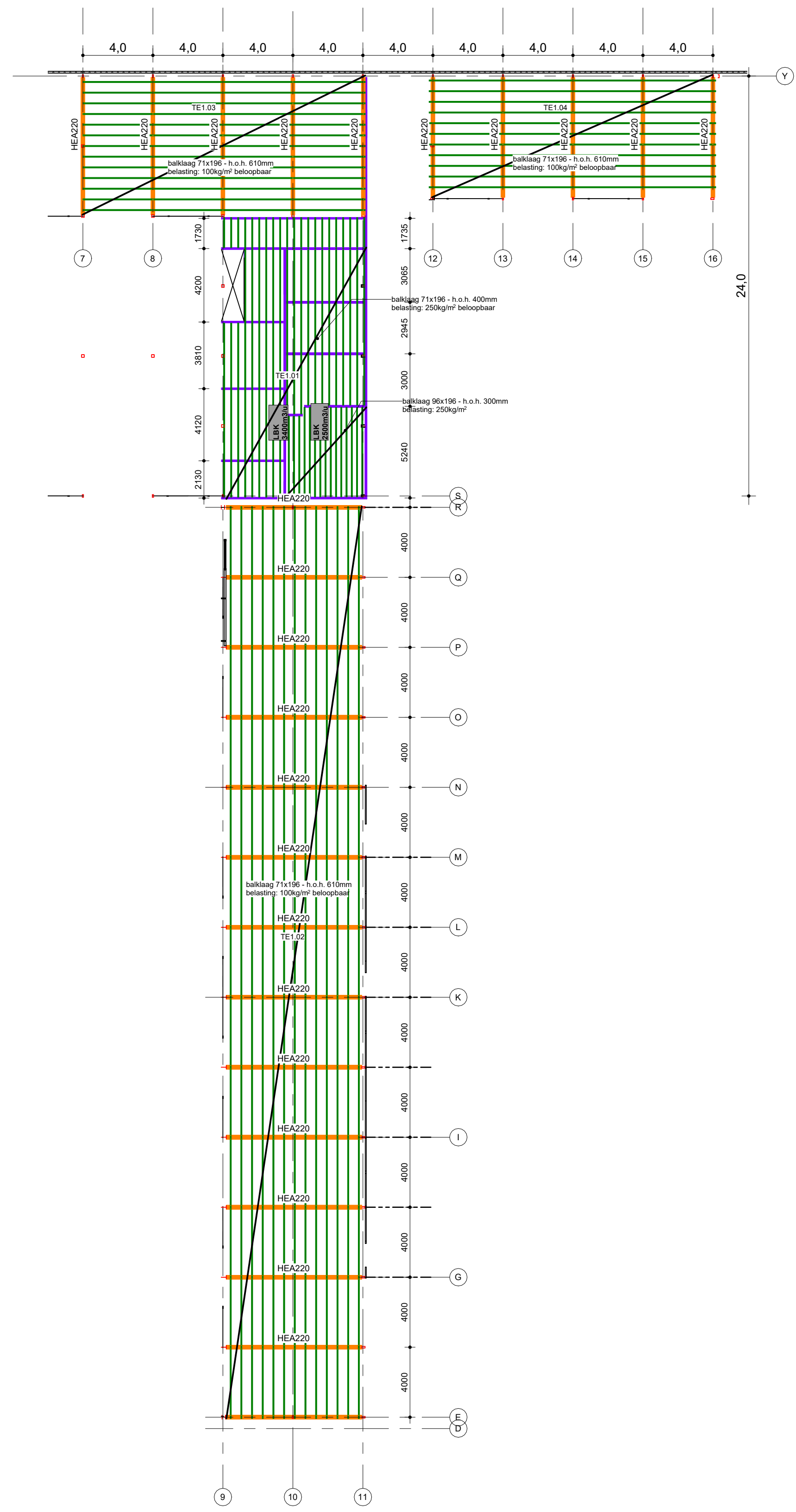
Eerste verdieping 1 : 200
