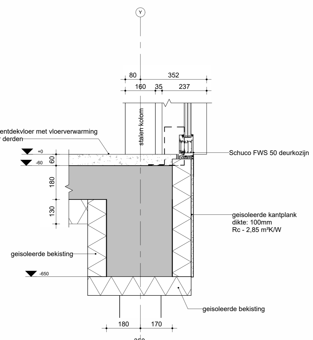
Detail 03 1 : 10
