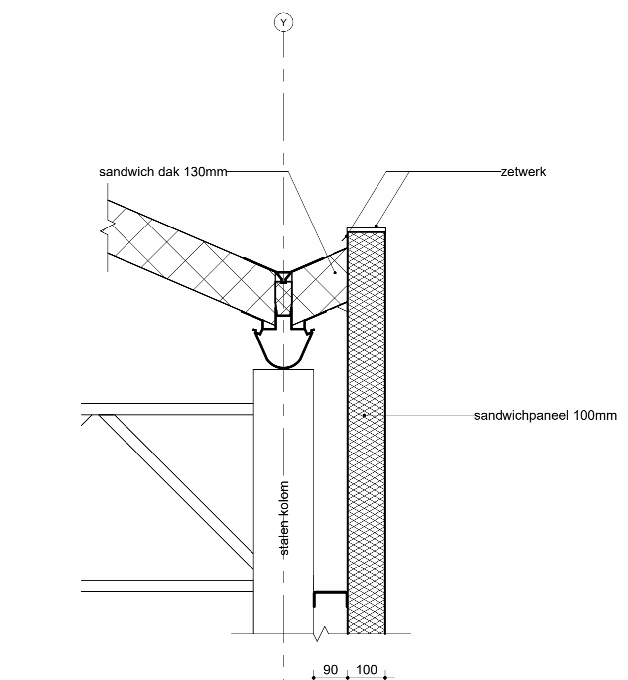
Detail 05 1 : 10
