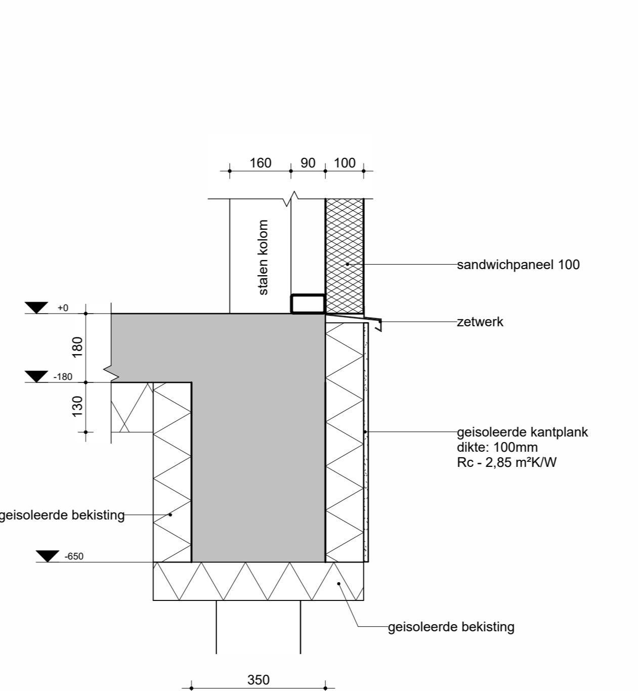
Detail 04 1 : 10
