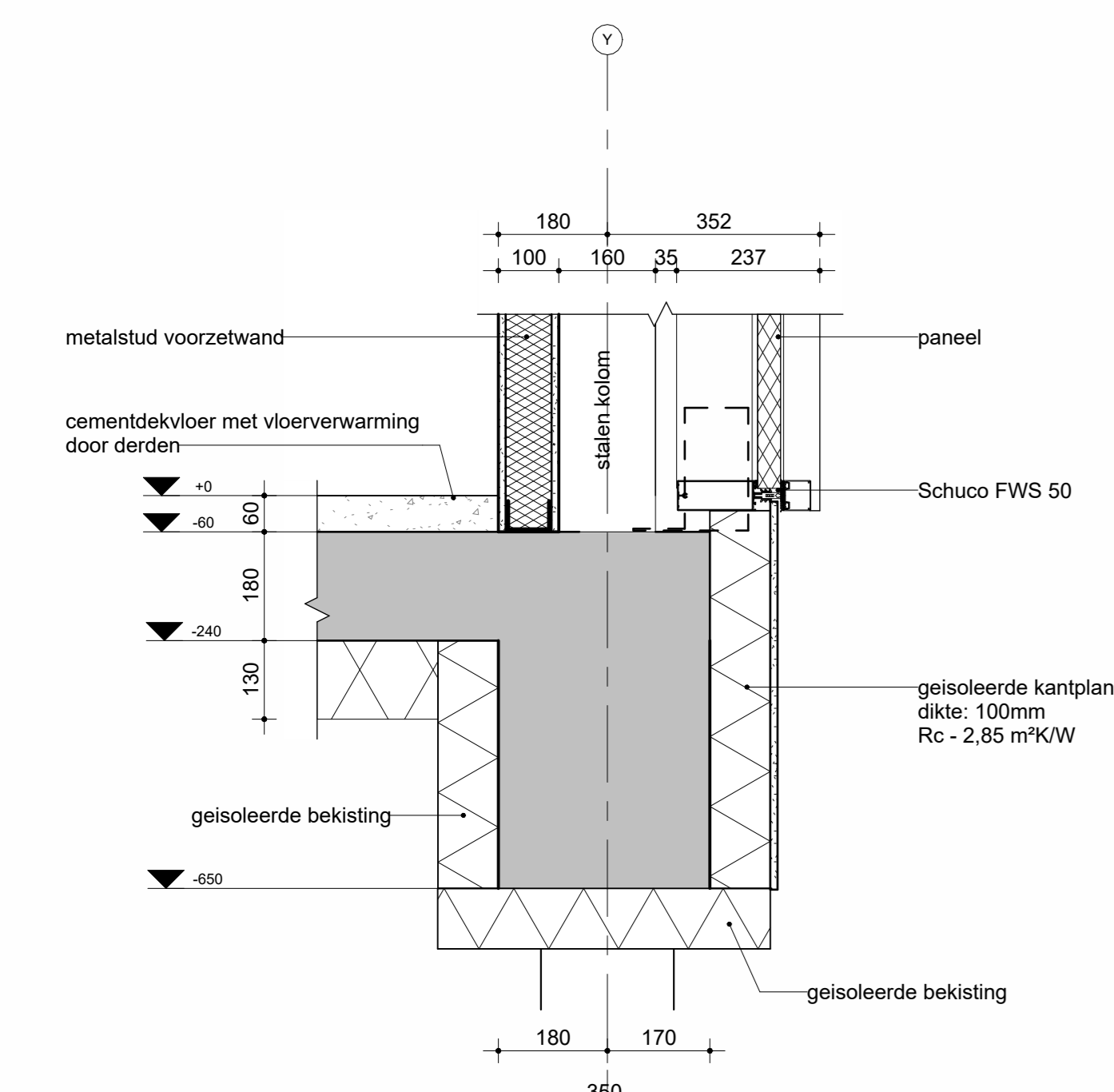
Detail 01 1 : 10
