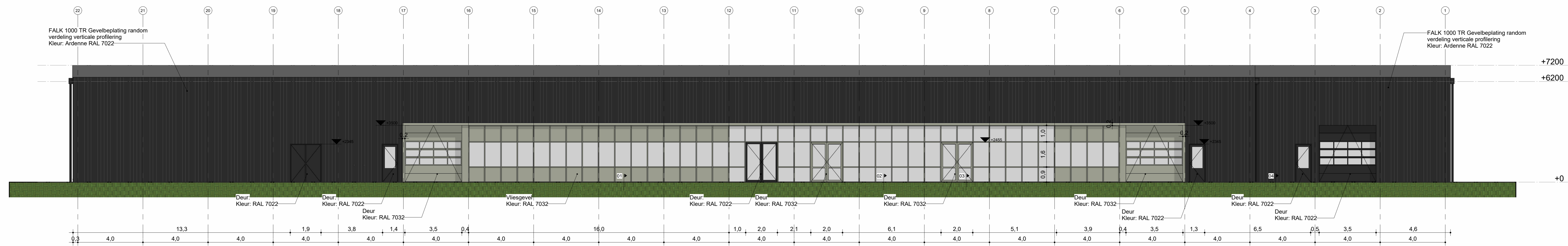
Achtergevel 1 : 100
