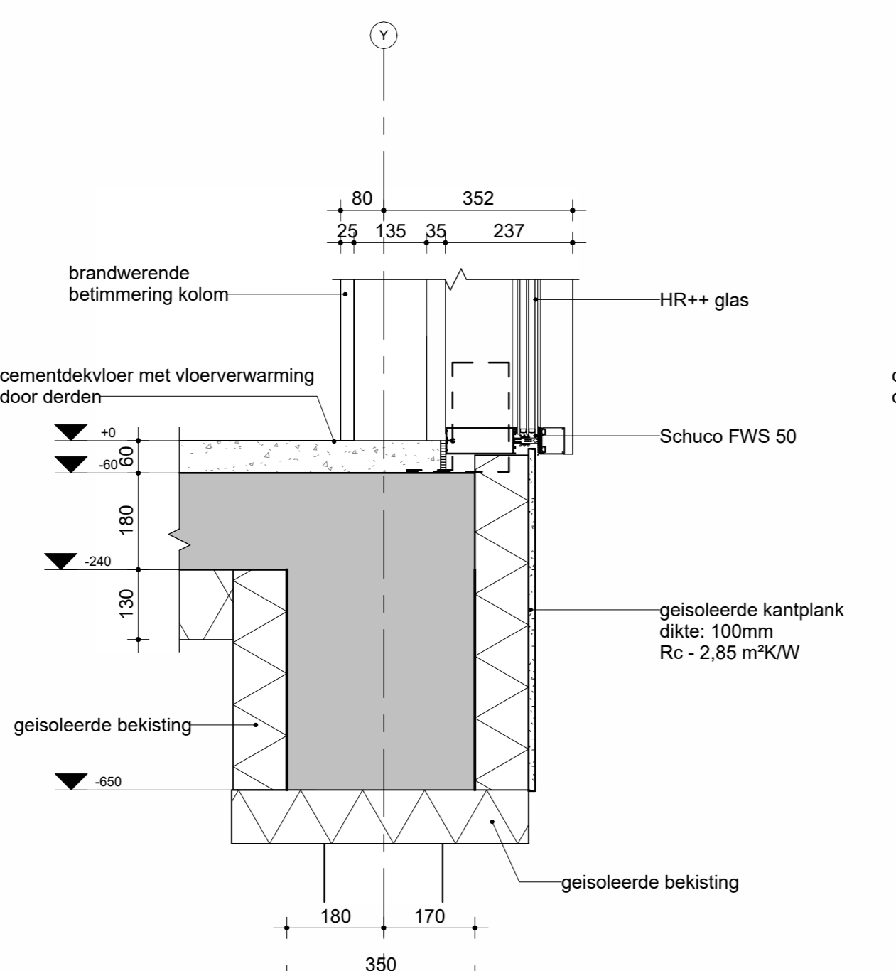
Detail 02 1 : 10
