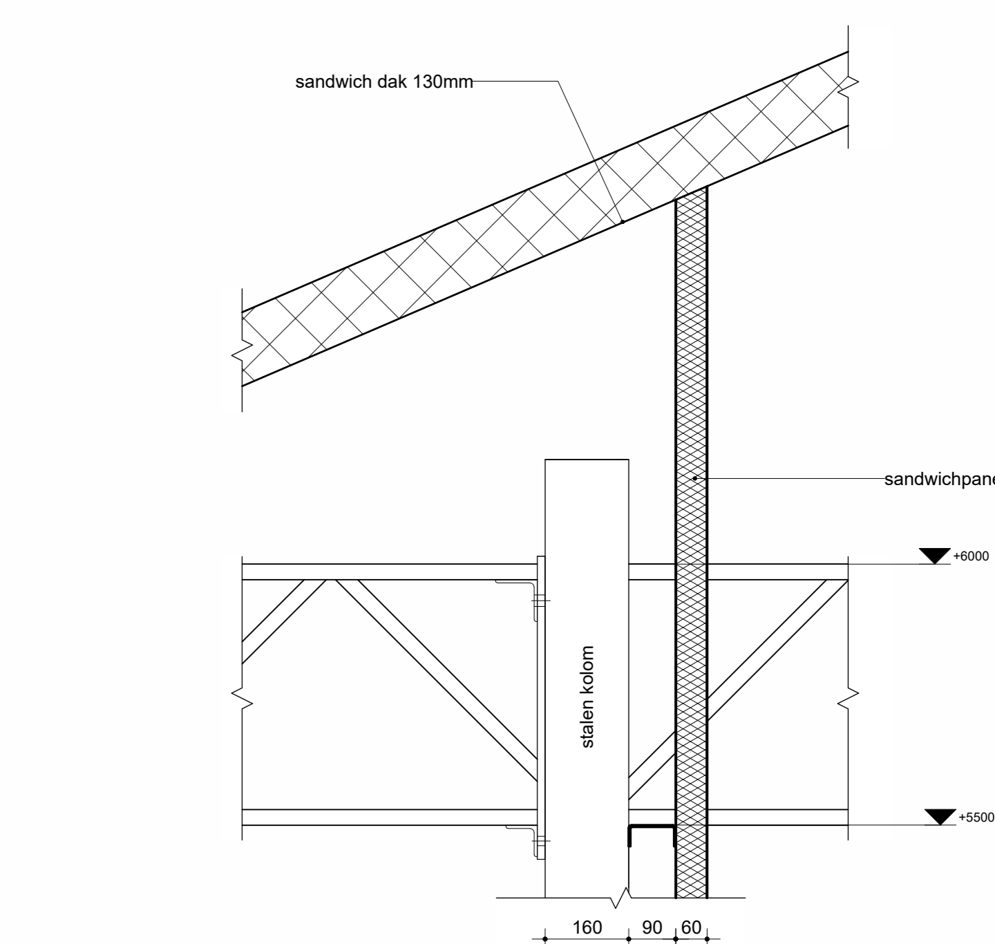
Detail 06 1 : 10
