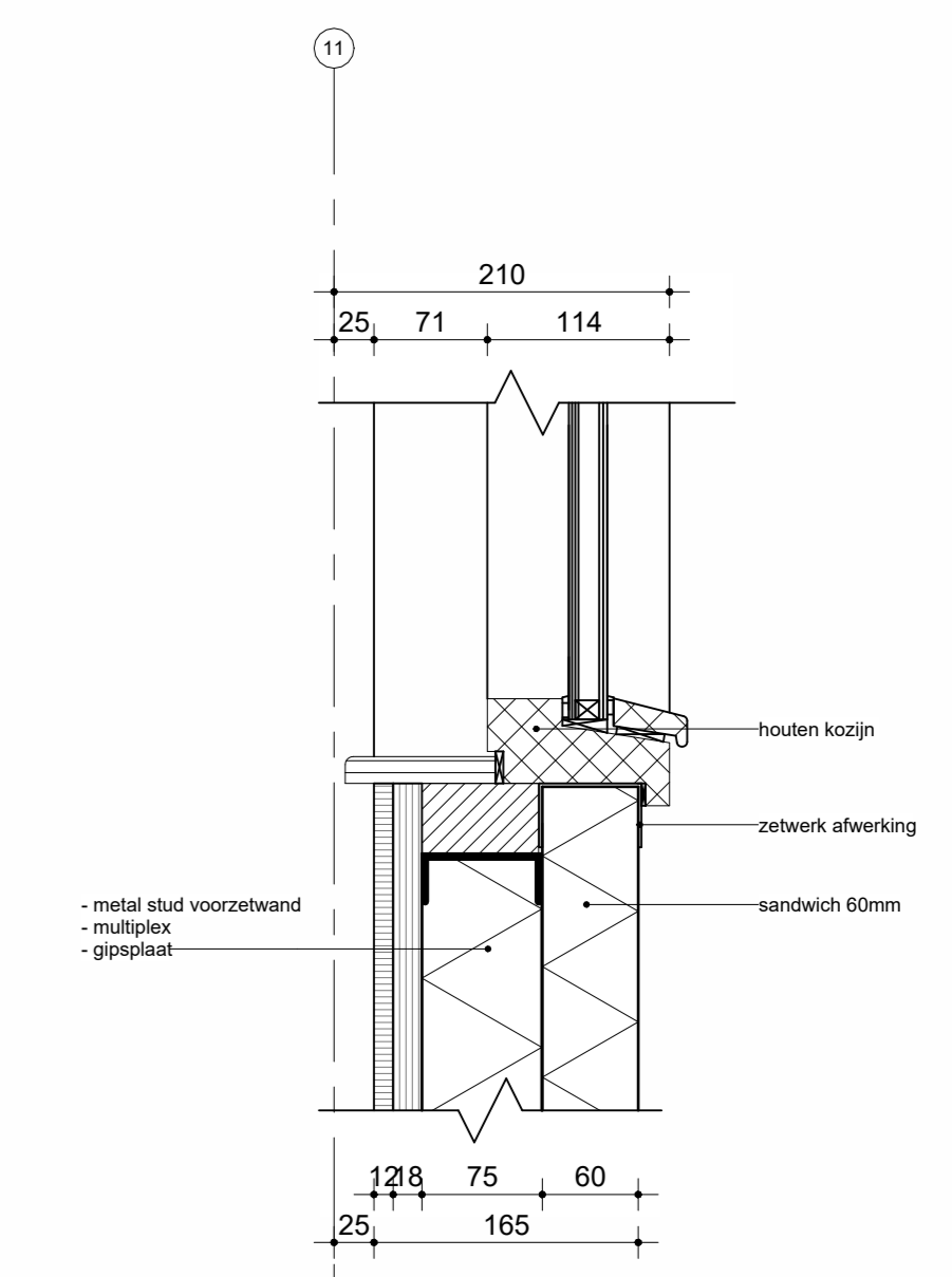
Kozijnaansluiting 1 : 5
